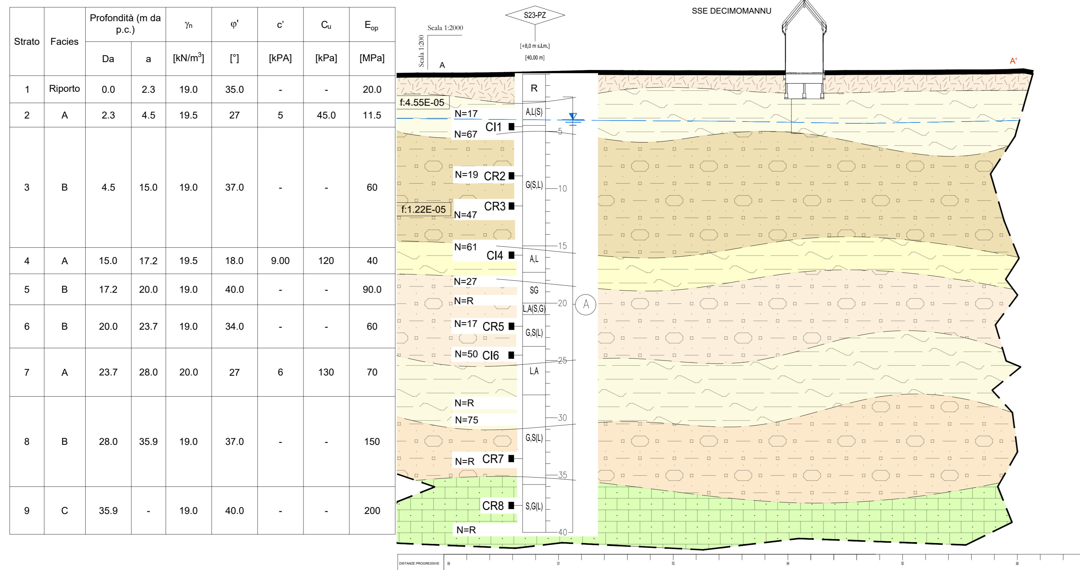
Profilo Geologico - Scala 1:2000/200
