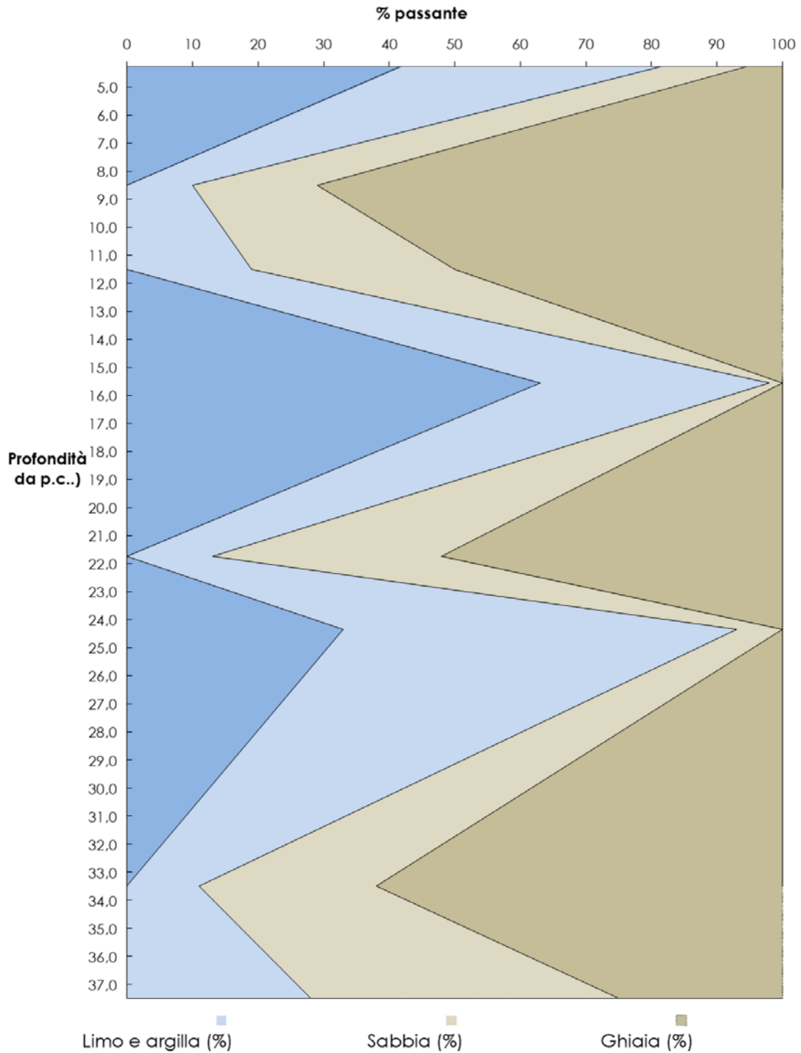
Figura 8-9 – Ripartizione granulometrica
