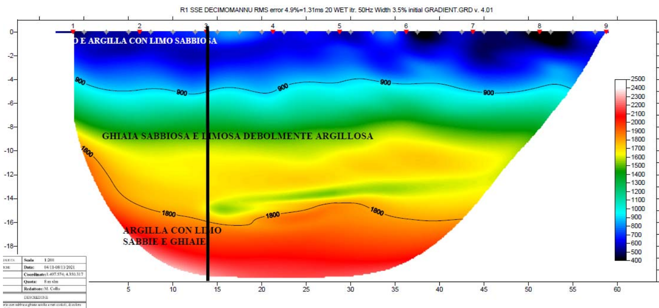
Figura 8-6 – Estratto dei risultati delle prove sismiche a rifrazione
