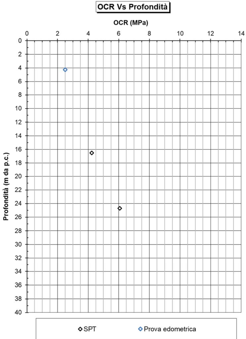
Figura 8-15 – Valori di OCR con la profondità
