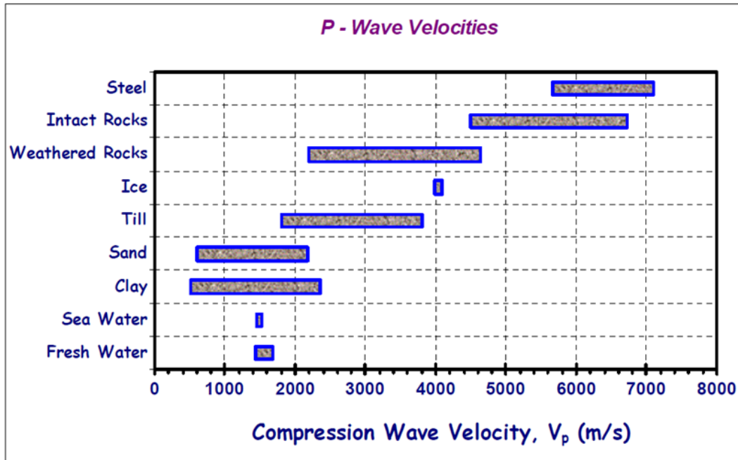
Figura 8-7 – Valori della velocità delle onde di corpo V_p per differenti materiali
