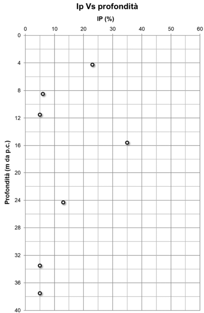
Figura 8-13 – Caratteristiche di plasticità: Indice di plasticità
