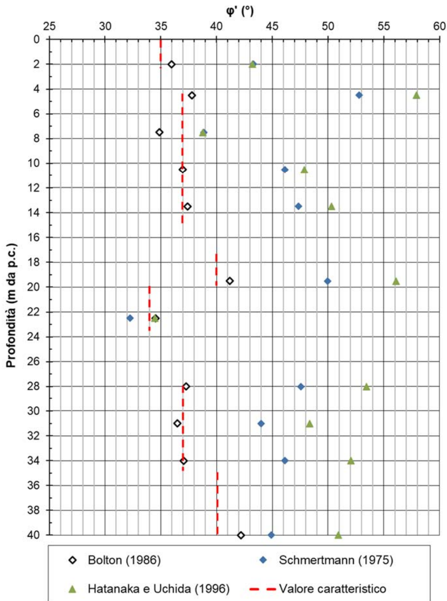
Figura 8-2 – Angolo d'attrito \phi' da N_{spt}
