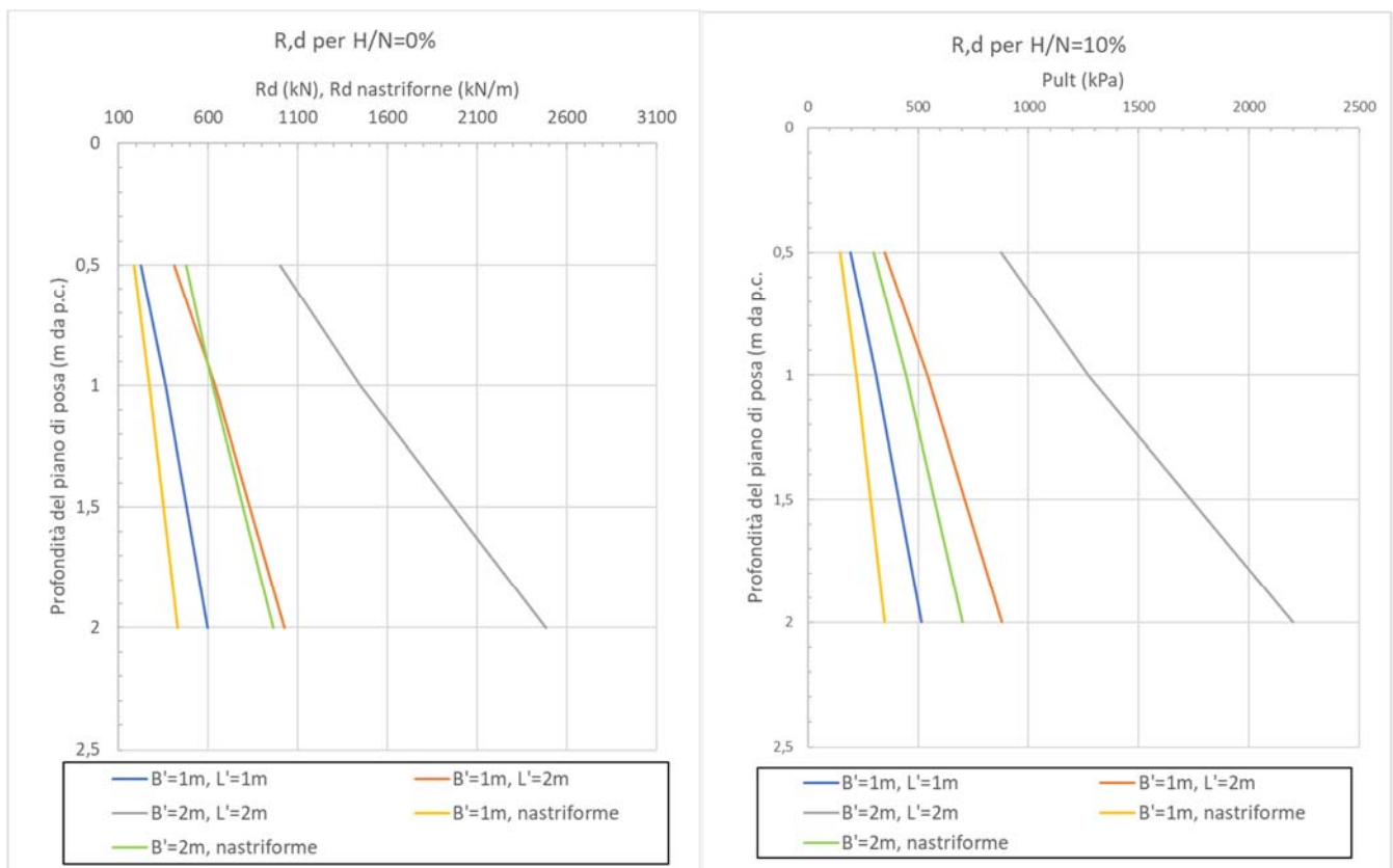
Figura 10-7 – Valori di R_d ottenuti per H/N=0\% (a sinistra) e H/N=10\% (a destra)
