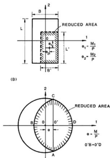
Figura 10-6 – Dimensioni efficaci per fondazioni quadrate e circolari sottoposte a carichi eccentrici (Meyerhof, 1963 [42])
