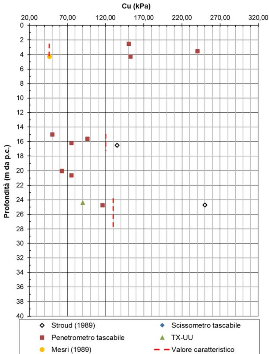
Figura 8-16 – Resistenza al taglio non drenata Cu
