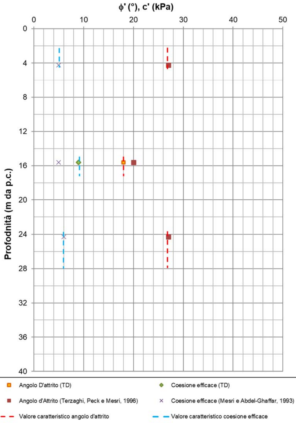
Figura 8-17 – Parametri di resistenza al taglio in condizioni drenate
