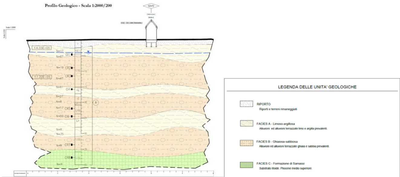
Figura 4-1 – Estratto della sezione geologica (Doc. Rif. [18])
