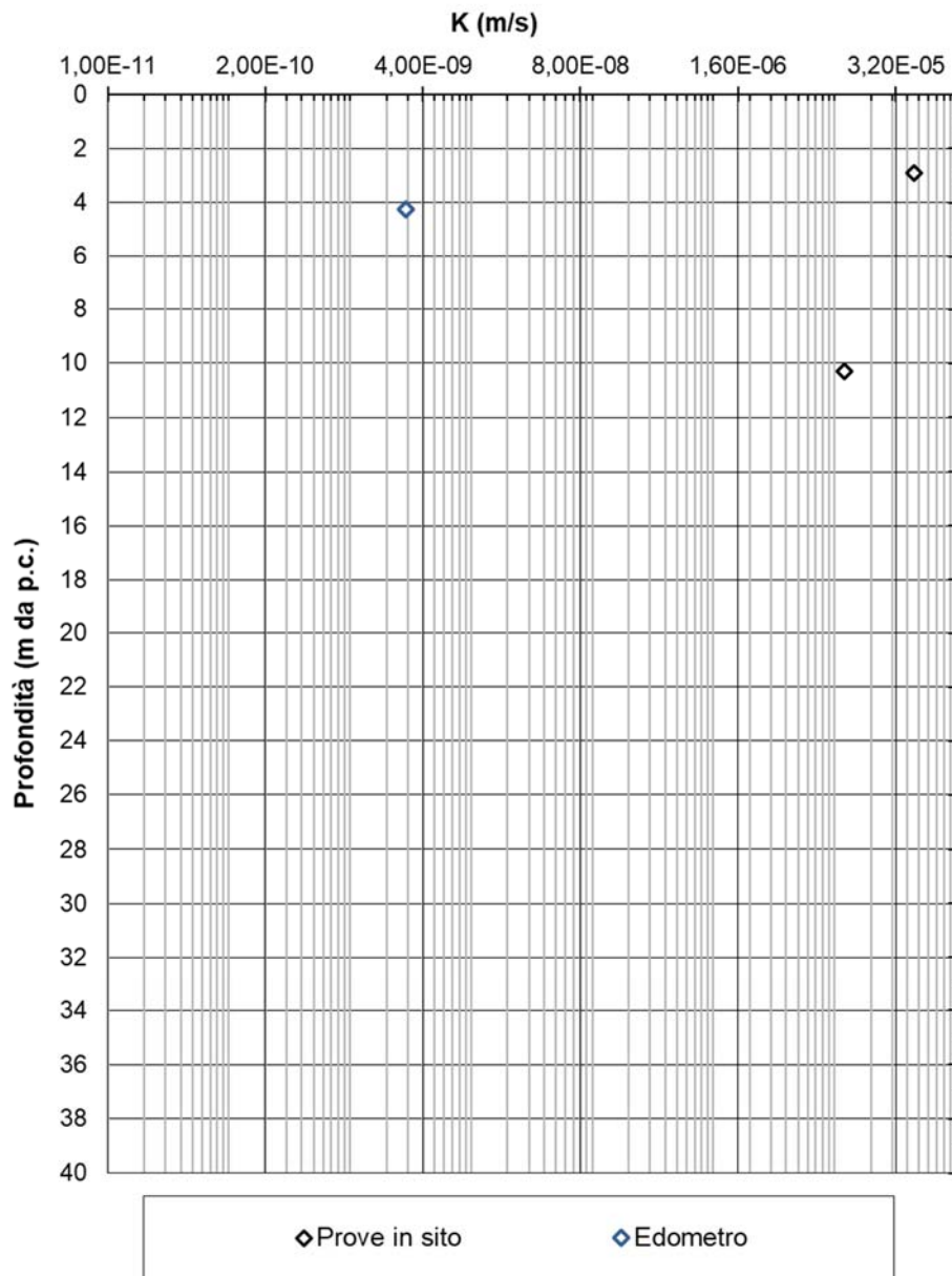
Figura 8-18 – Coefficienti di permeabilità
