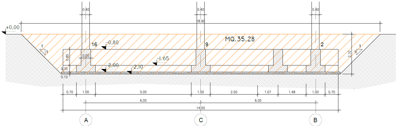
Figura 10-2 – Esempio di sezione trasversale delle fondazioni tipiche per strutture come quella in progetto
