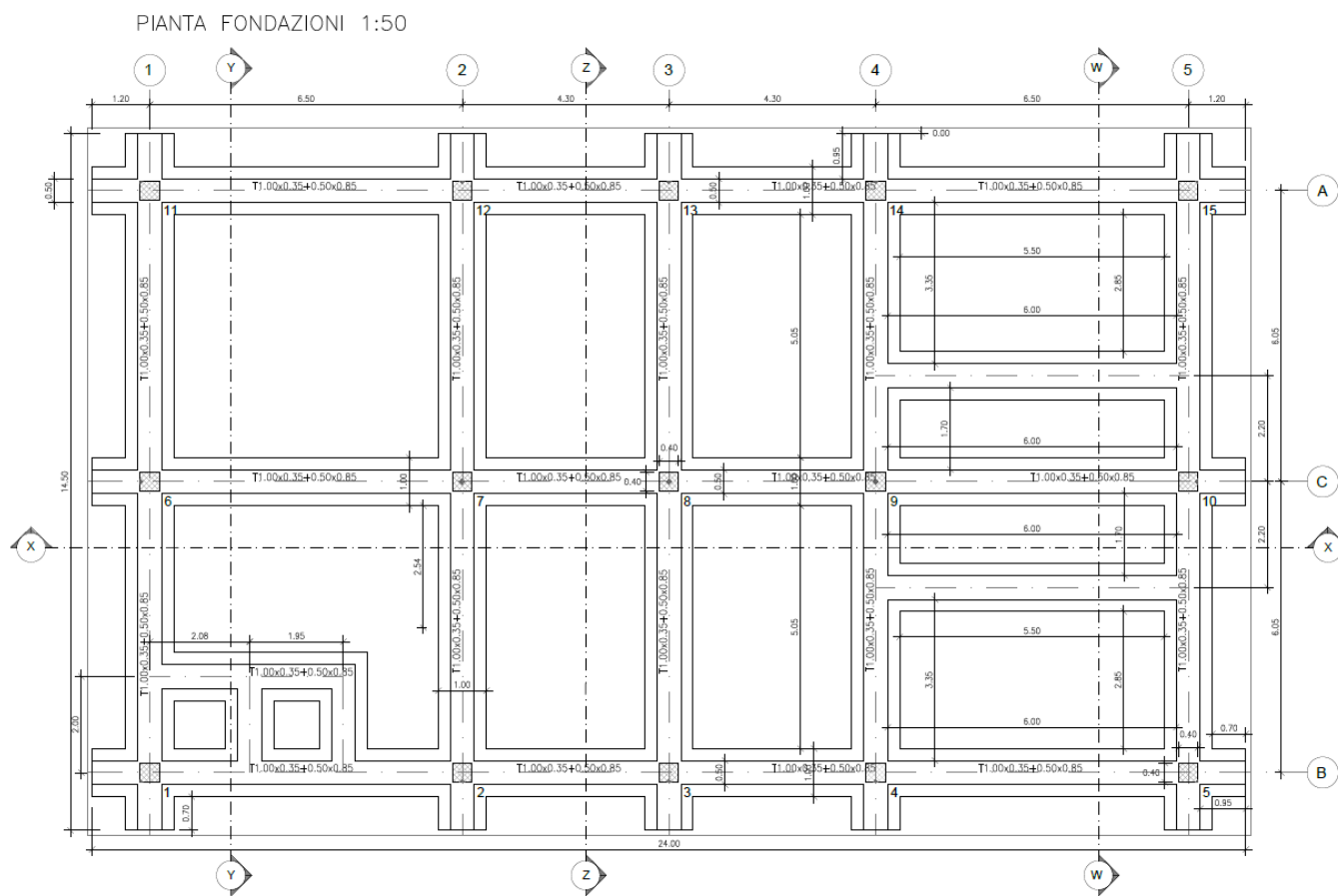
Figura 10-1 - Esempio di pianta fondazioni per strutture come quella in progetto
