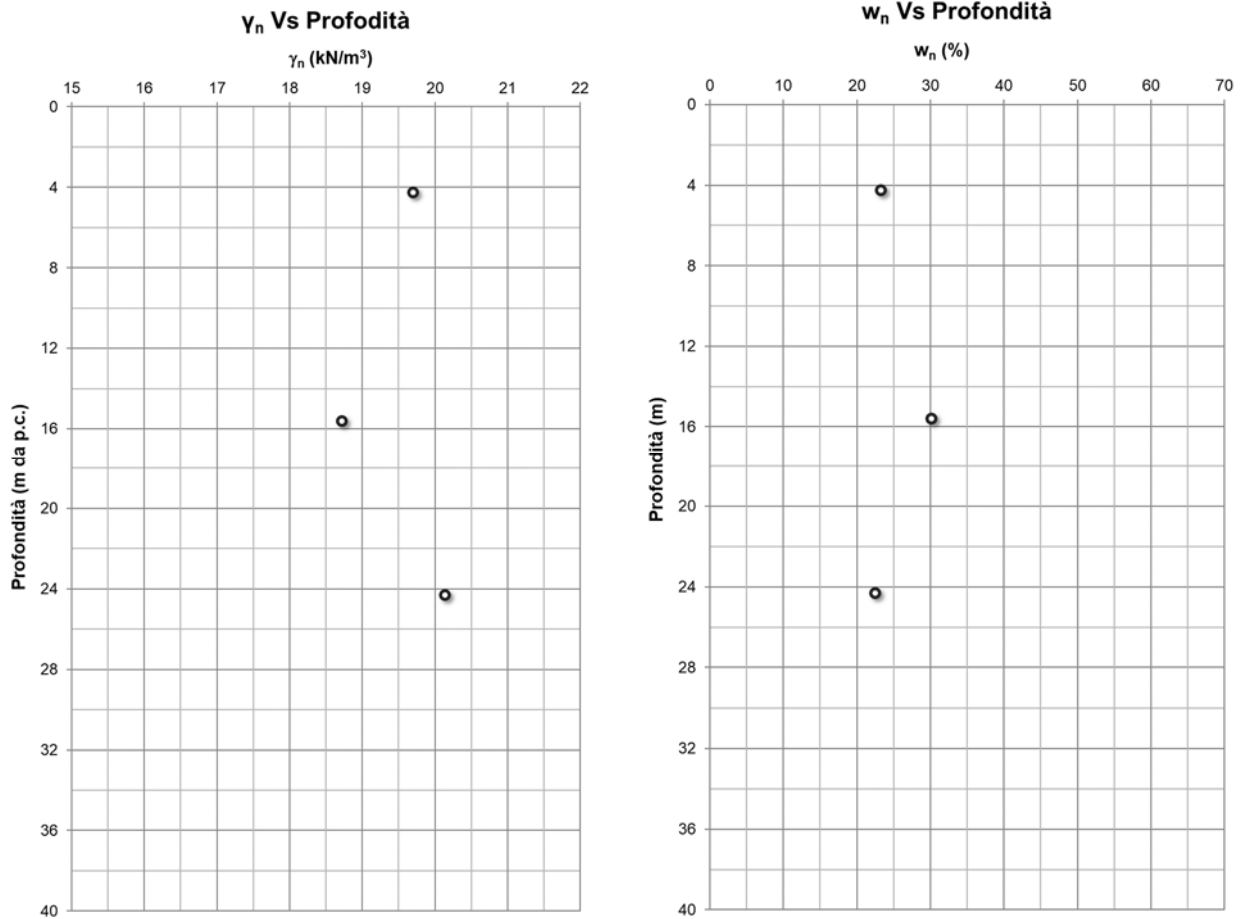
Figura 8-10 – Peso di volume naturale (a sinistra) e contenuto d'acqua naturale (a destra)
