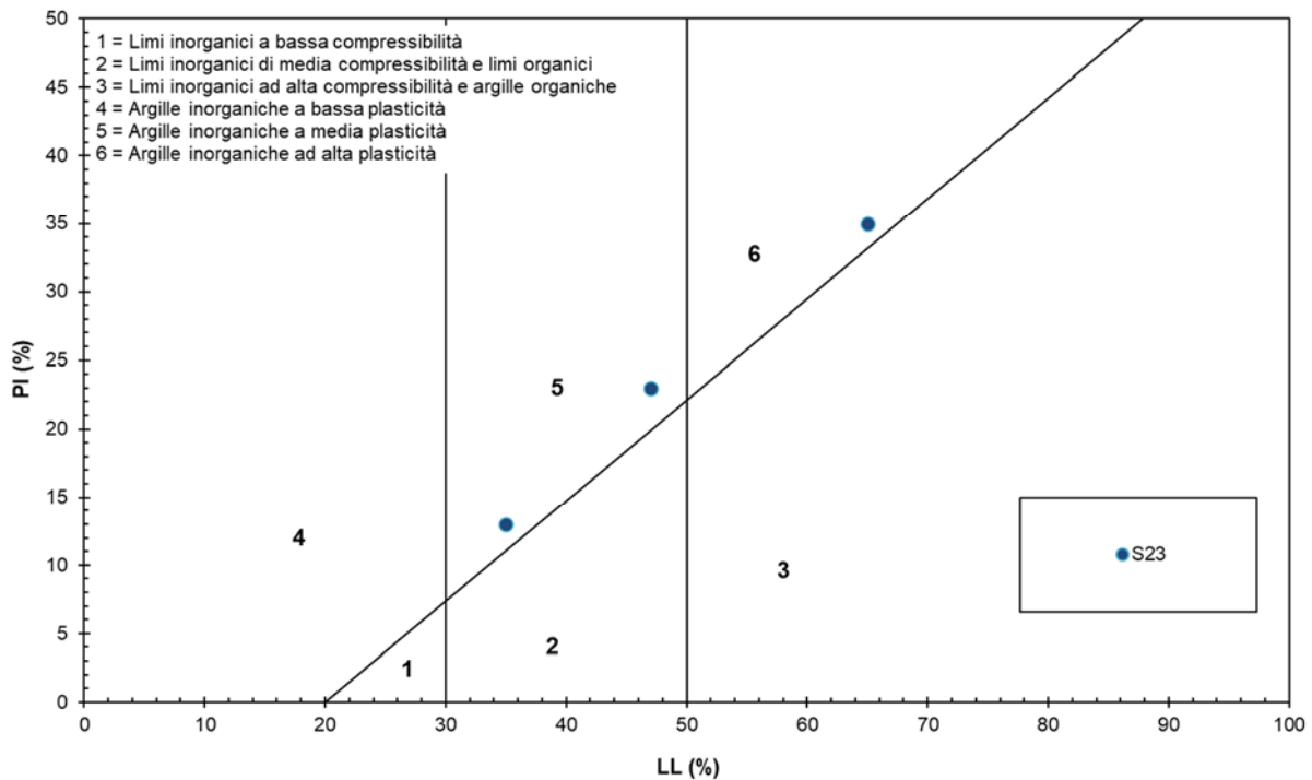
Figura 8-14 – Carta di plasticità di Casagrande
