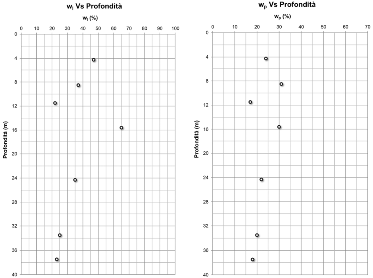
Figura 8-12 – Caratteristiche di plasticità: Limite liquido (a sinistra) e Limite plastico (a destra)
