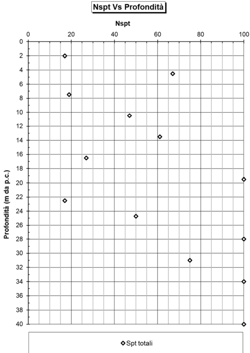
Figura 5-2 – Risultati delle prove penetrometriche dinamiche (SPT) NSPT
