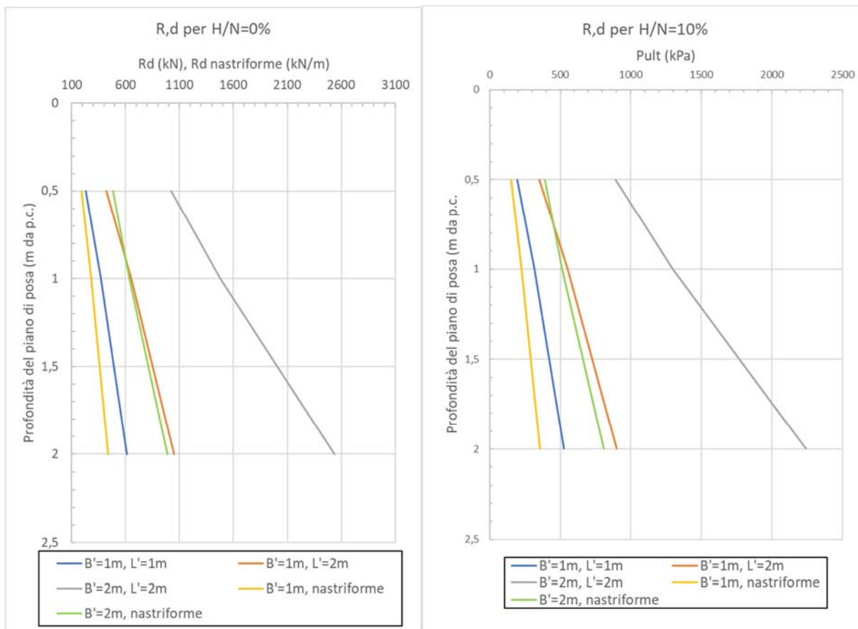
Figura 10-7 – Valori di R_d ottenuti per H/N=0\% (a sinistra) e H/N=10\% (a destra) – Condizioni drenate
