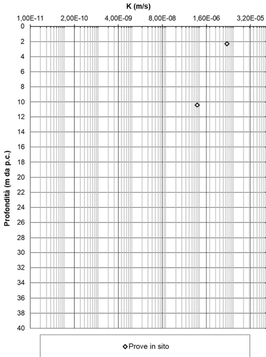
Figura 8-19 – Coefficienti di permeabilità
