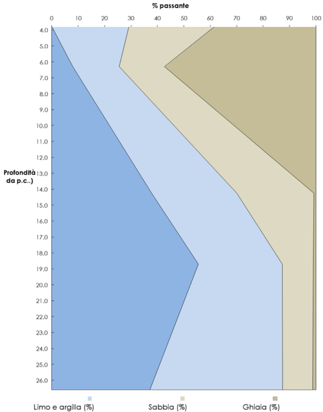
Figura 8-10 – Ripartizione granulometrica
