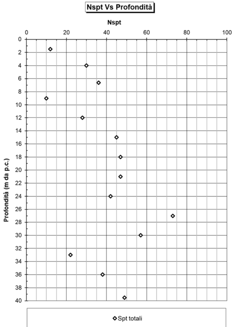
Figura 5-2 – Risultati delle prove penetrometriche dinamiche (SPT) N_{SPT}
