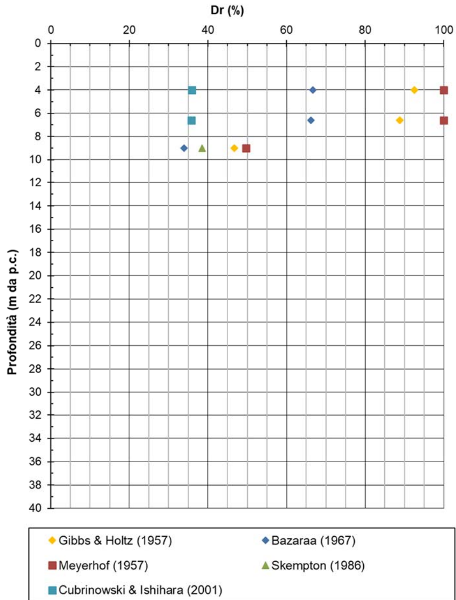
Figura 8-1 - Densità relativa D_r da N_{spt}
