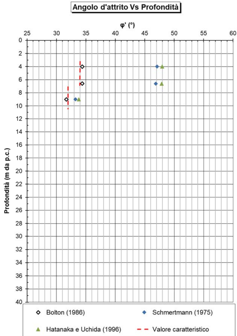
Figura 8-2 – Angolo d'attrito \phi' da N_{spt}
