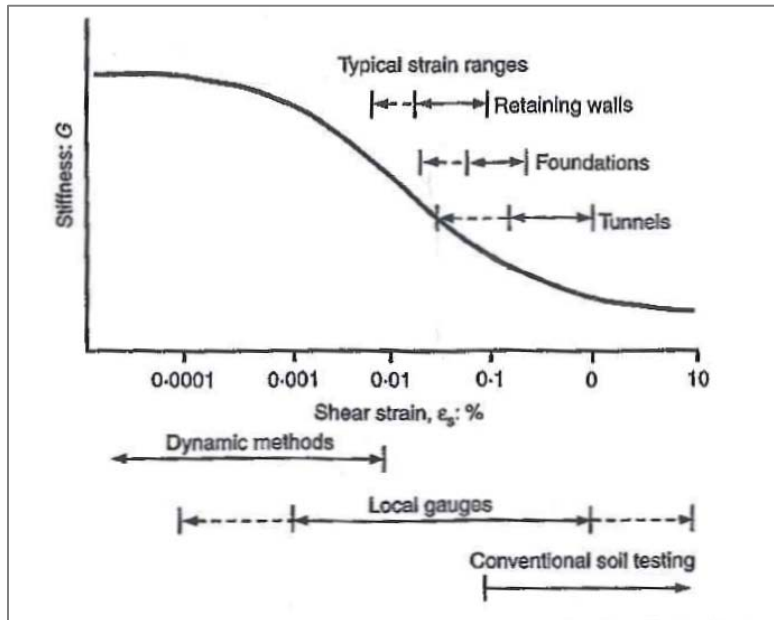
Figura 7-1 - Decadimento del modulo di taglio di un terreno con il livello di deformazione ed intervalli di deformazione tipici nei problemi geotecnici (Atkinson, 2000 [22])
