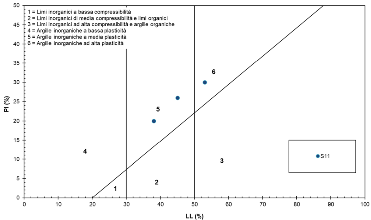
Figura 8-15 – Carta di plasticità di Casagrande
