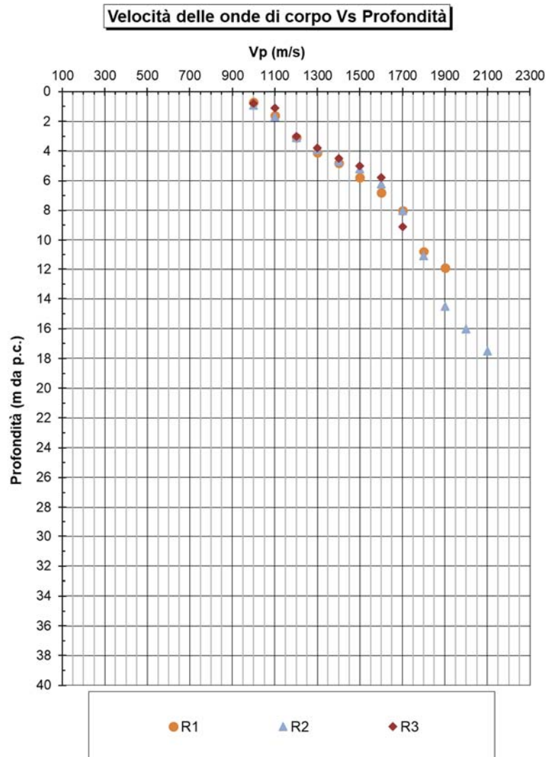
Figura 8-6 – Velocità delle onde di corpo V_p da prove sismiche a rifrazione
