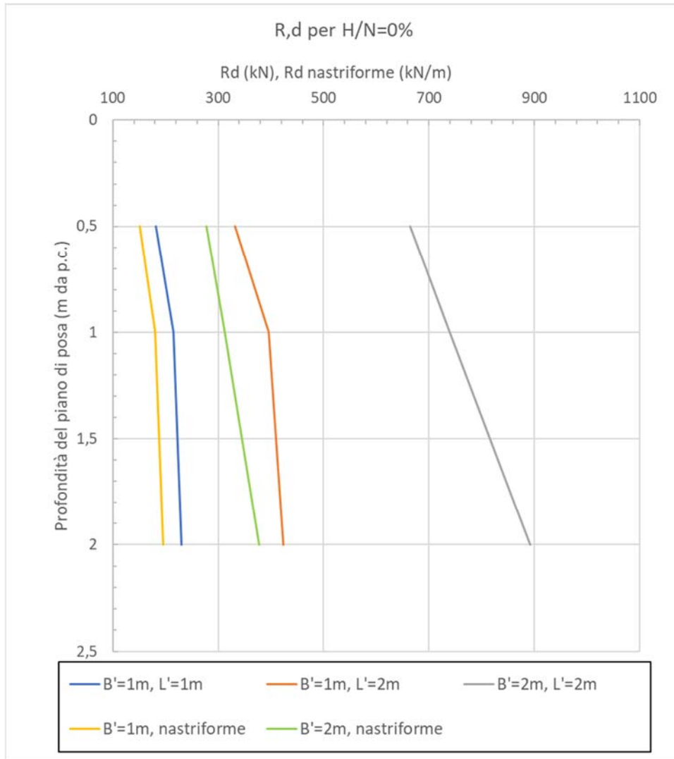
Figura 10-8 – Valori di R d ottenuti per H/N=0% - Condizioni non drenate
