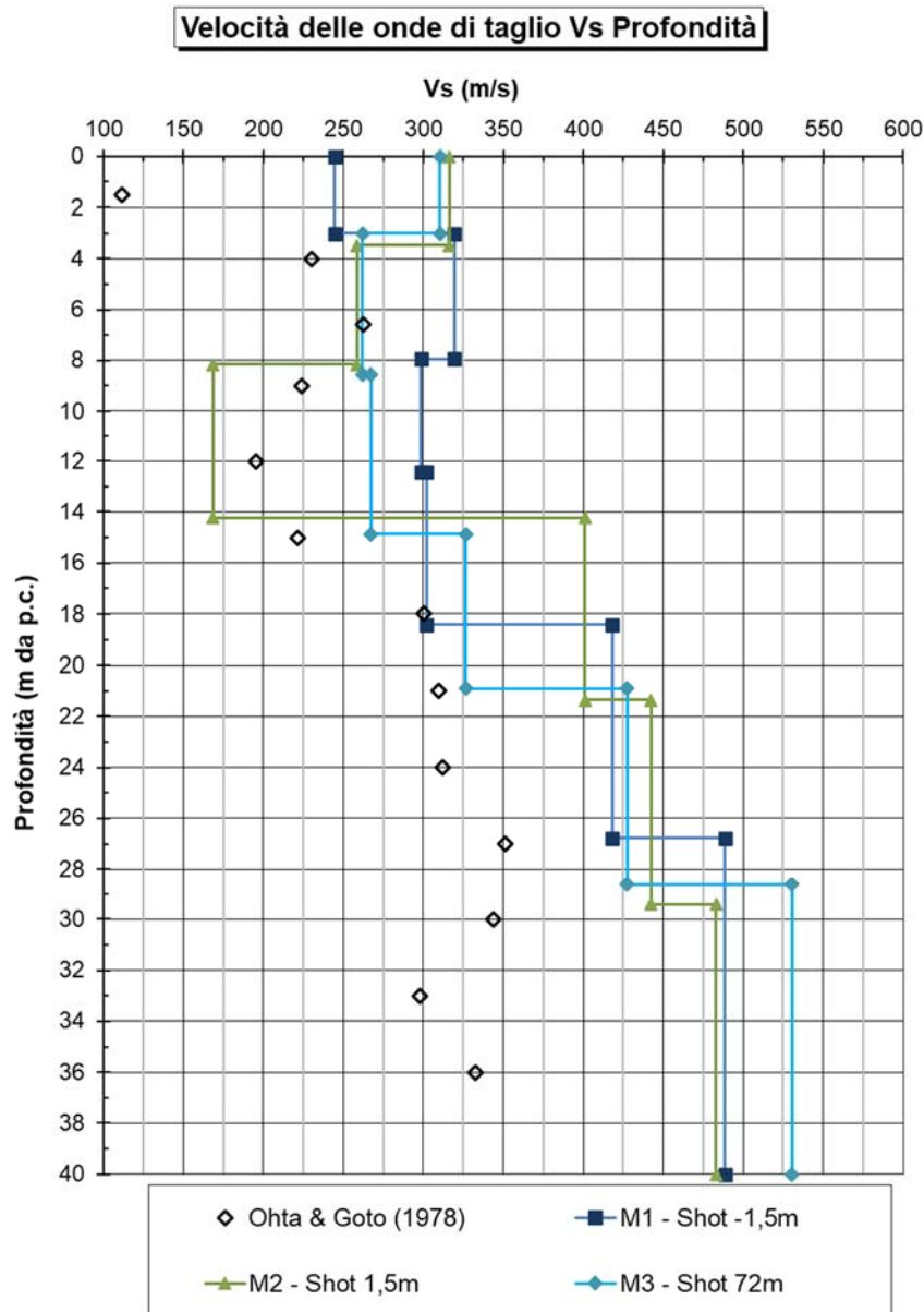
Figura 8-3 – Velocità delle onde di taglio V_s
