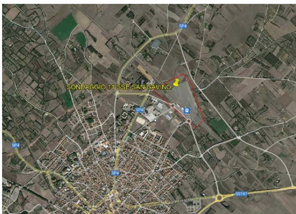
Figura 5-1 – Planimetria con ubicazione delle indagini
