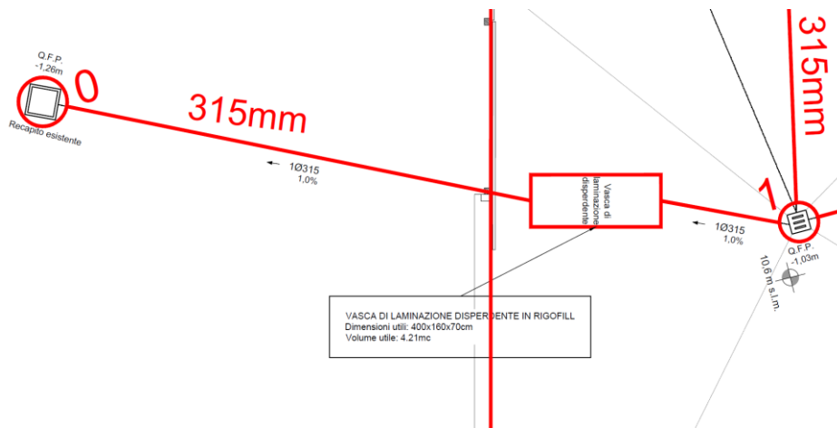
Figura 4-6 SSE Oristano – stralcio planimetrico della vasca disperdente, della condotta di by-pass e del pozzetto di recapito
