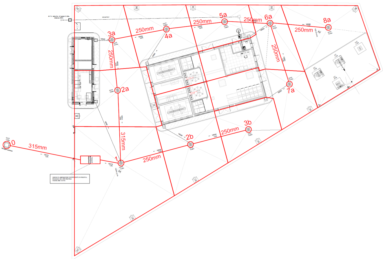
Figura 4-4 Stralcio planimetro della rete di drenaggio adottata per il piazzale.
