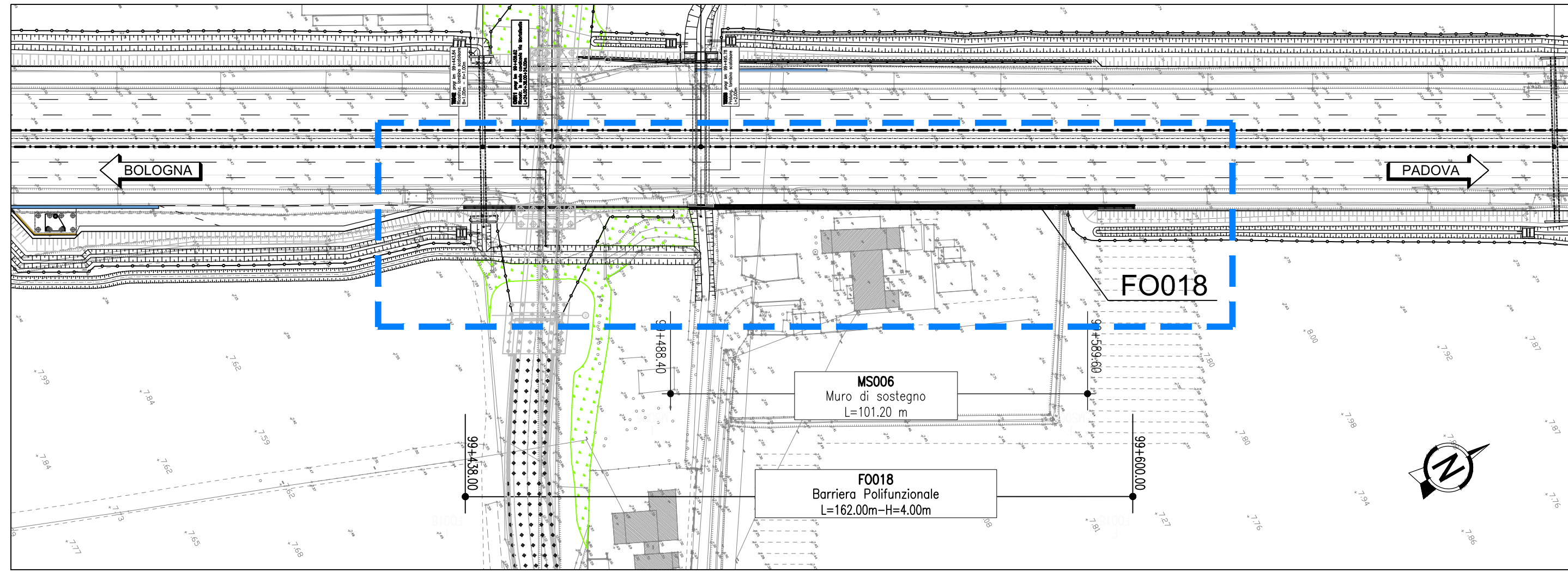
PLANIMETRIA DI PROGETTO 1:200
