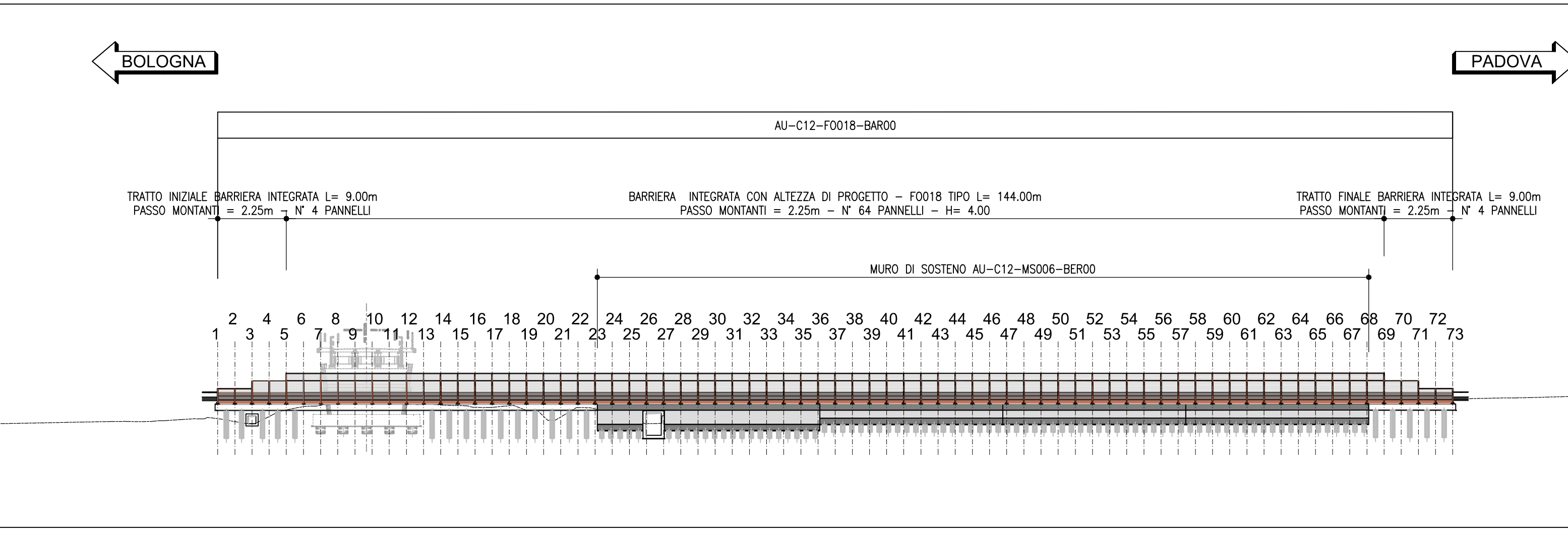
PROSPETTO D'ASSIEME 1:500
