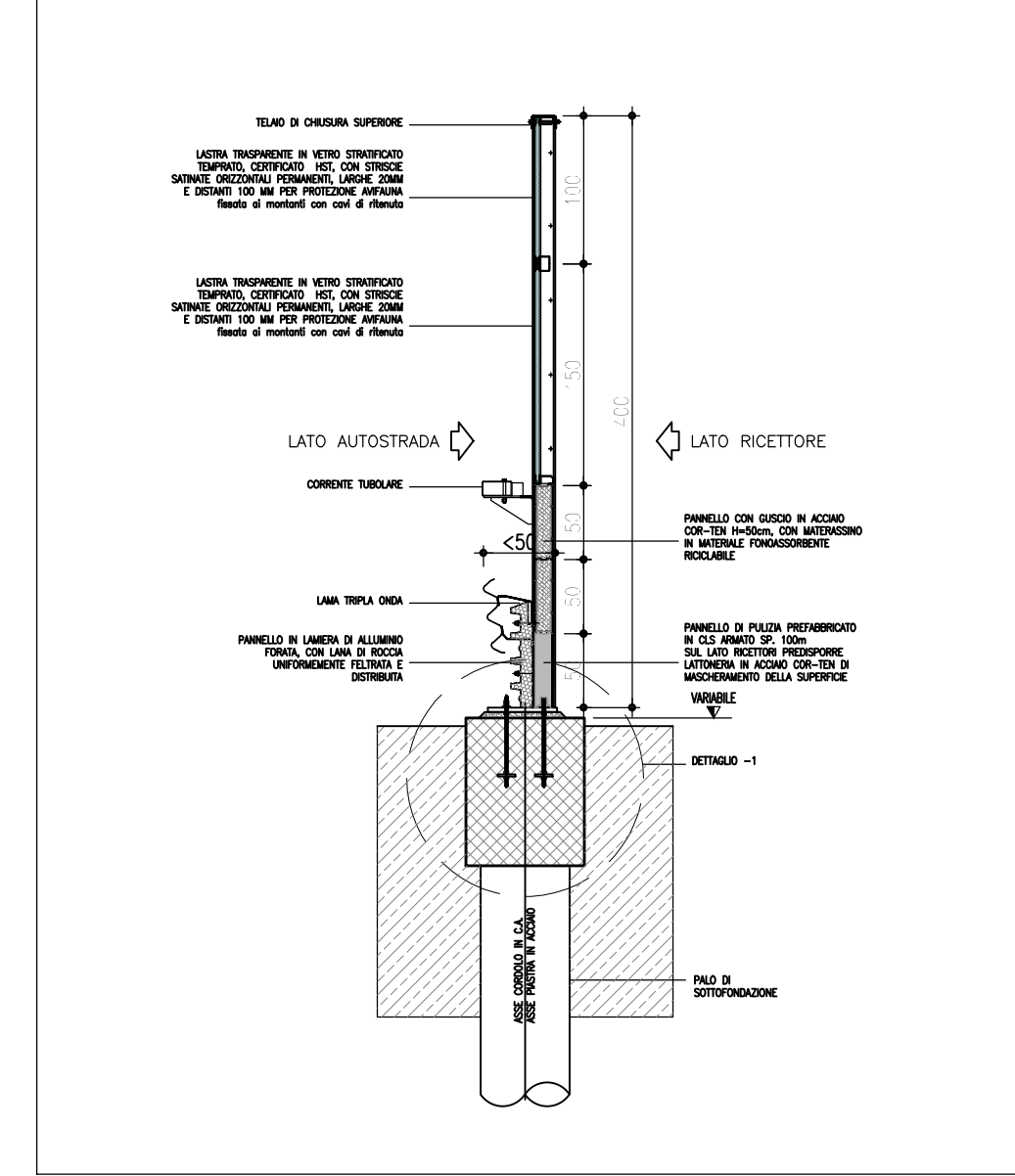
TRACCEMONTI BARRIERA
