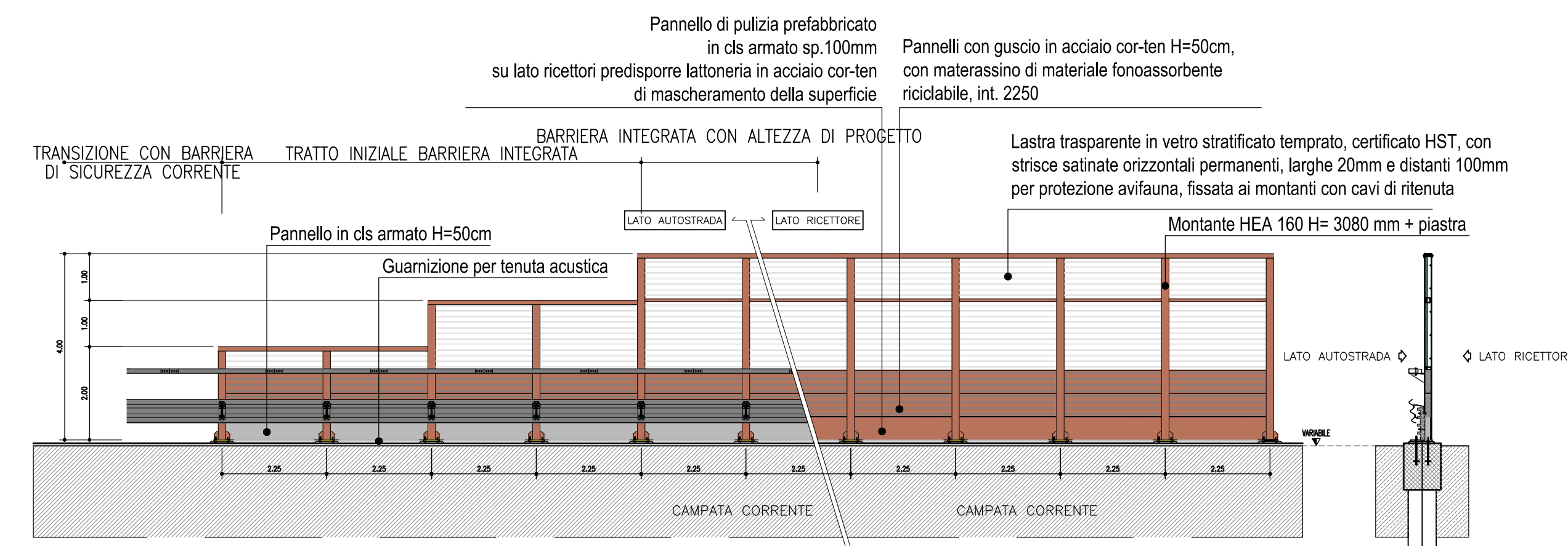
PROSPETTO BARRIERA "TIPO 1 P INTEGRATO H4 TRASPARENTE", LATO STRADA E LATO RICETTORE
