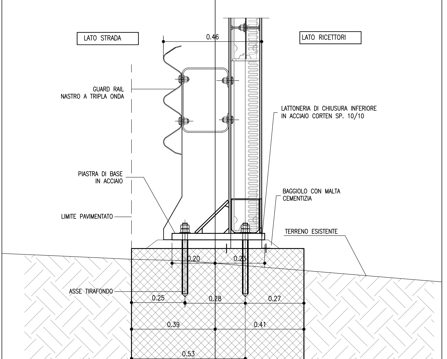
DETTAGLIO "1" 1:10
