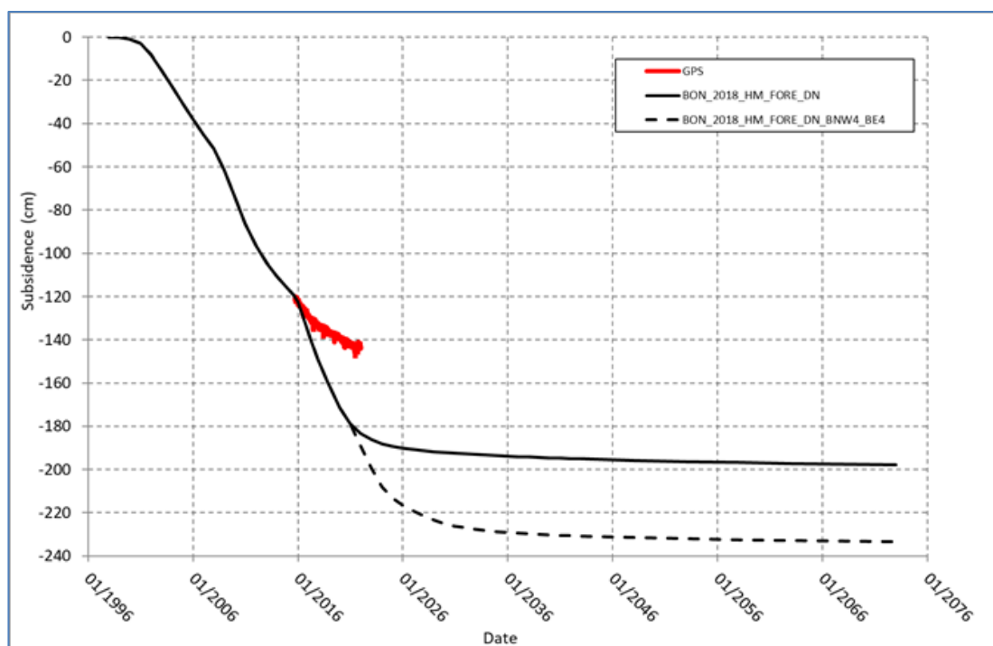
Figura 18 - Campo di Bonaccia: abbassamento misurato e calcolato in corrispondenza del CGPS della p.ma di Bonaccia NW
