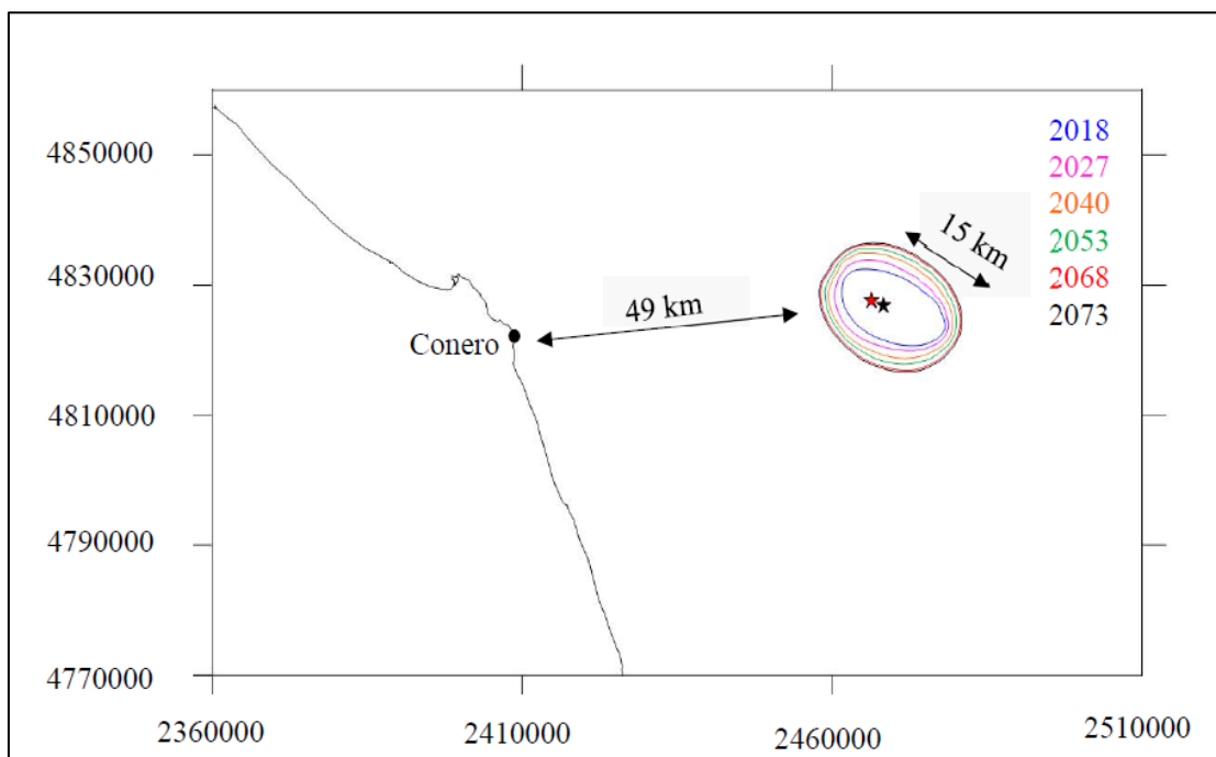
Figura 8 - Campo di Bonaccia: evoluzione temporale della linea di iso-subsidenza dei 2 cm
