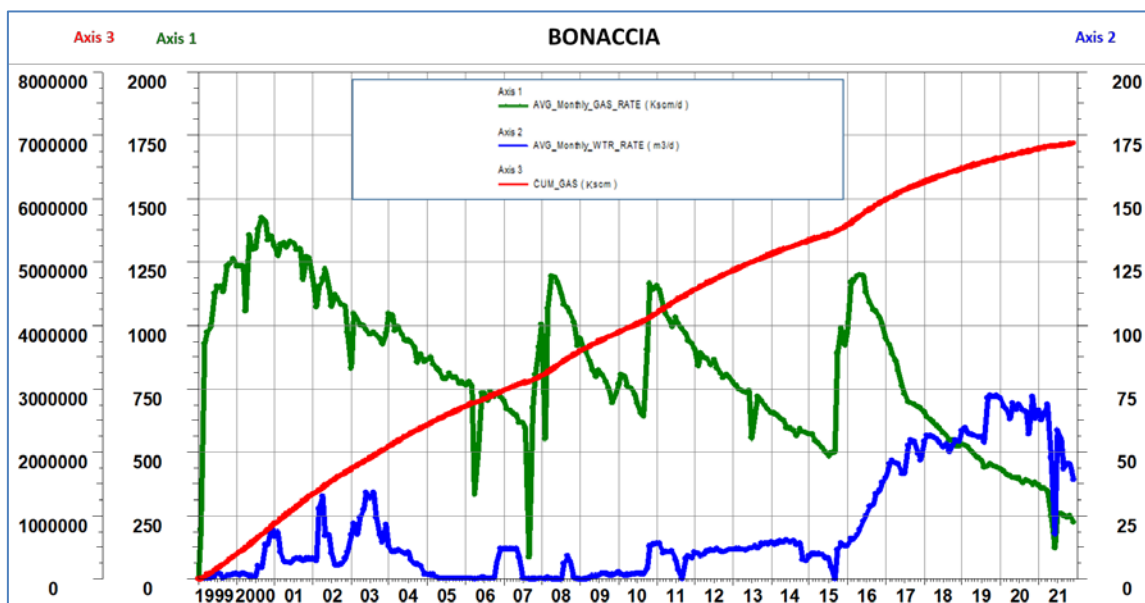
Figura 3 - Campo di Bonaccia: grafico della produzione storica
