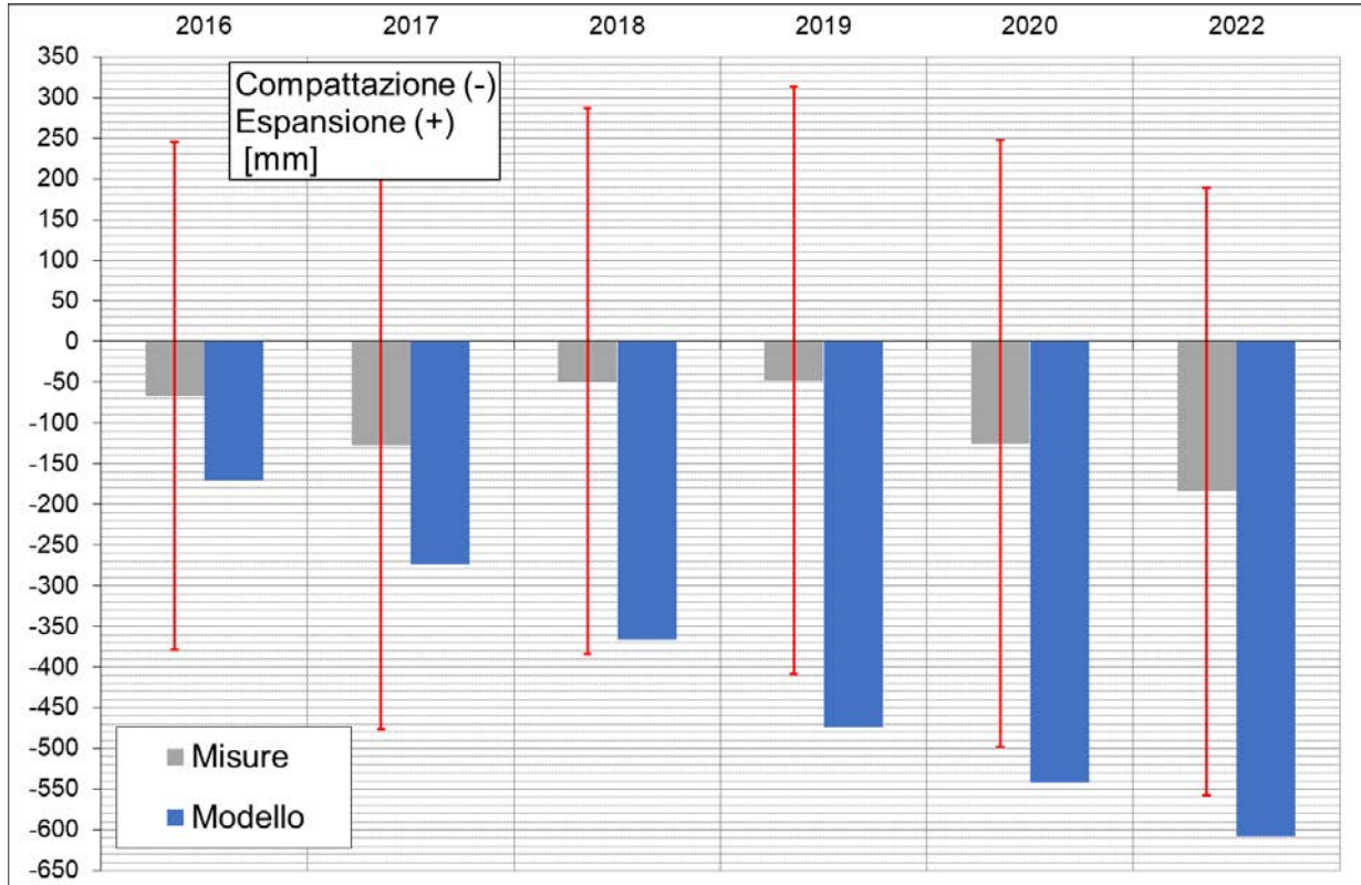
Figura 20 - Campo di Bonaccia: confronto tra le deformazioni verticali misurate e le corrispondenti stime del modello geomeccanico (pozzo Bonaccia NW 1dir). Indicato in rosso l'intervallo di confidenza delle misure pari a 3\sigma
