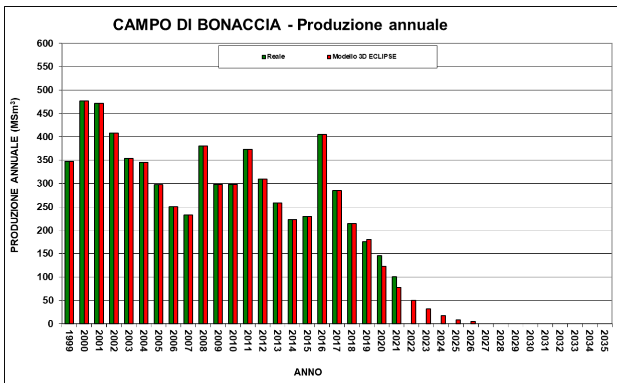
Figura 6 - Campo di Bonaccia: produzione e riserve da modello Eclipse 2018 (scenario DN)
