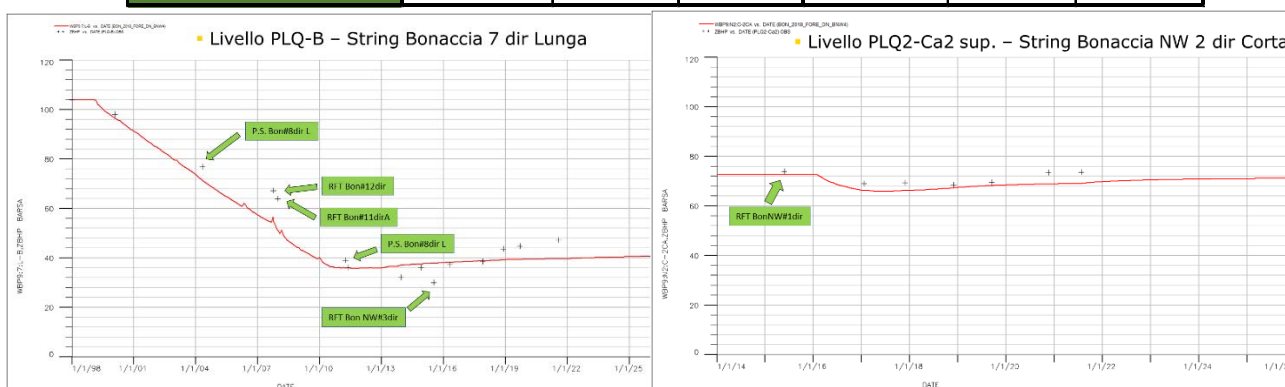
Figura 7 - Campo di Bonaccia: confronto tra i dati di pressione da profili statici e modello Eclipse 2018
