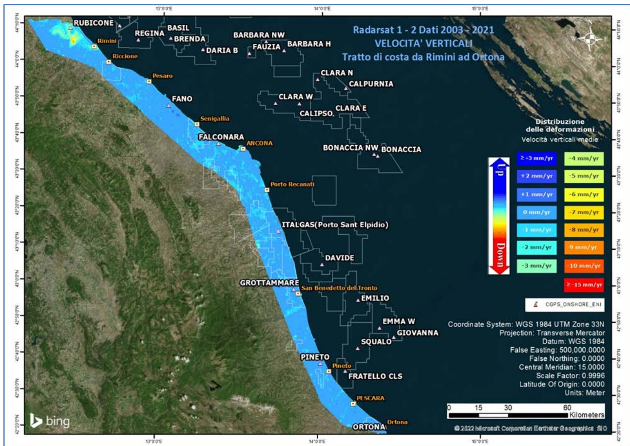
Figura 12 - Campo di Bonaccia: analisi dei dati SAR dal 2003 al 2021
