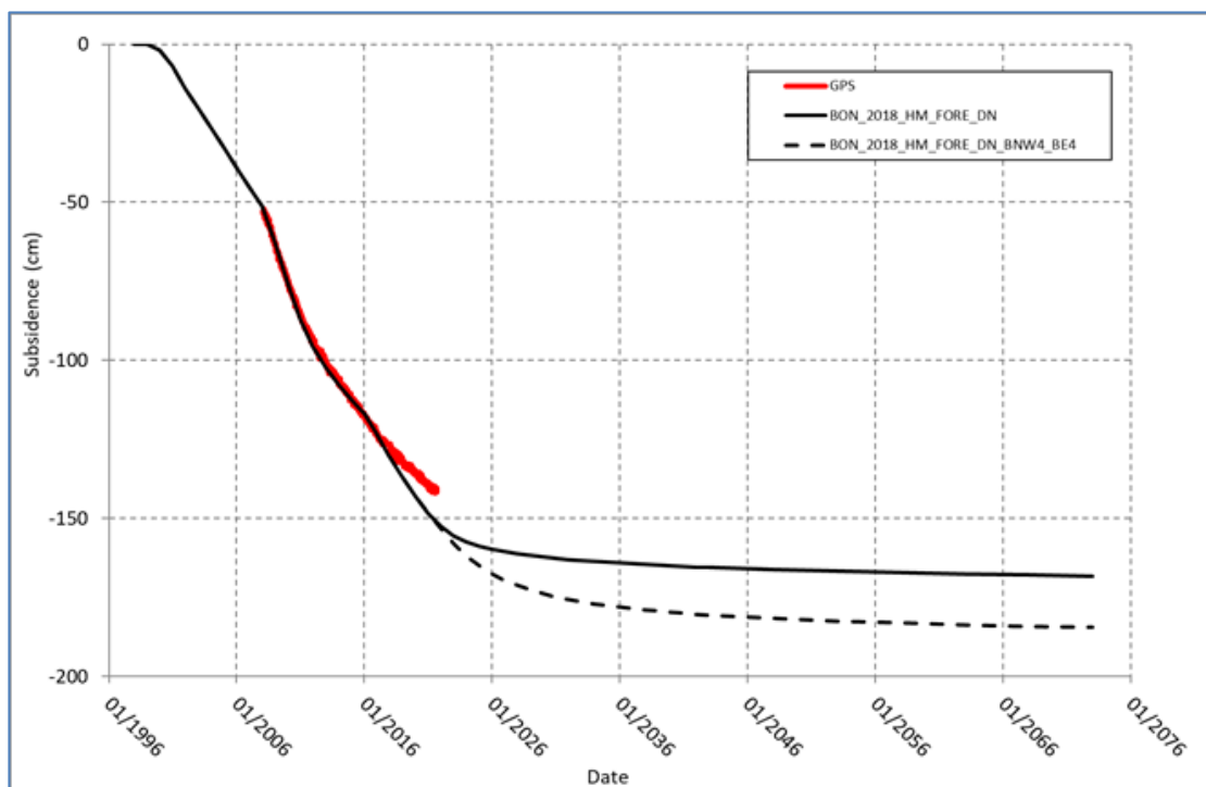
Figura 17 - Campo di Bonaccia: abbassamento misurato e calcolato in corrispondenza del CGPS della p.ma di Bonaccia
