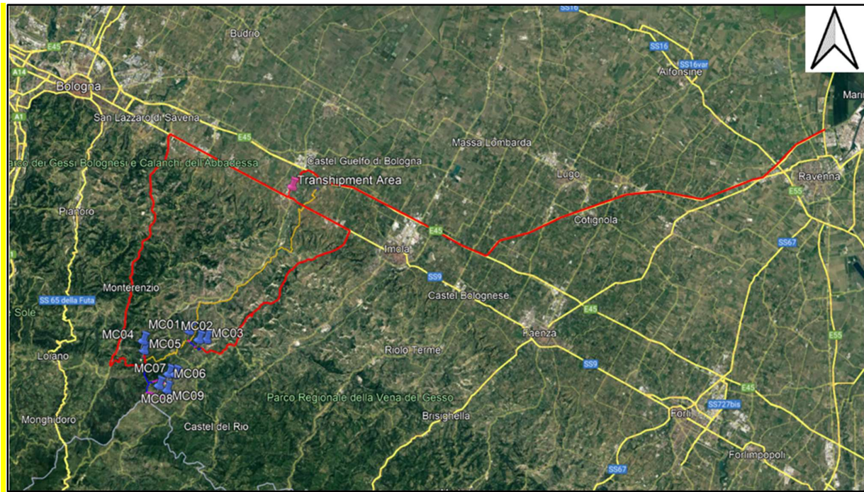
Figura 6.7: Layout d’impianto con viabilità di accesso dal Porto di Ravenna (linee rosse) su immagine satellitare
