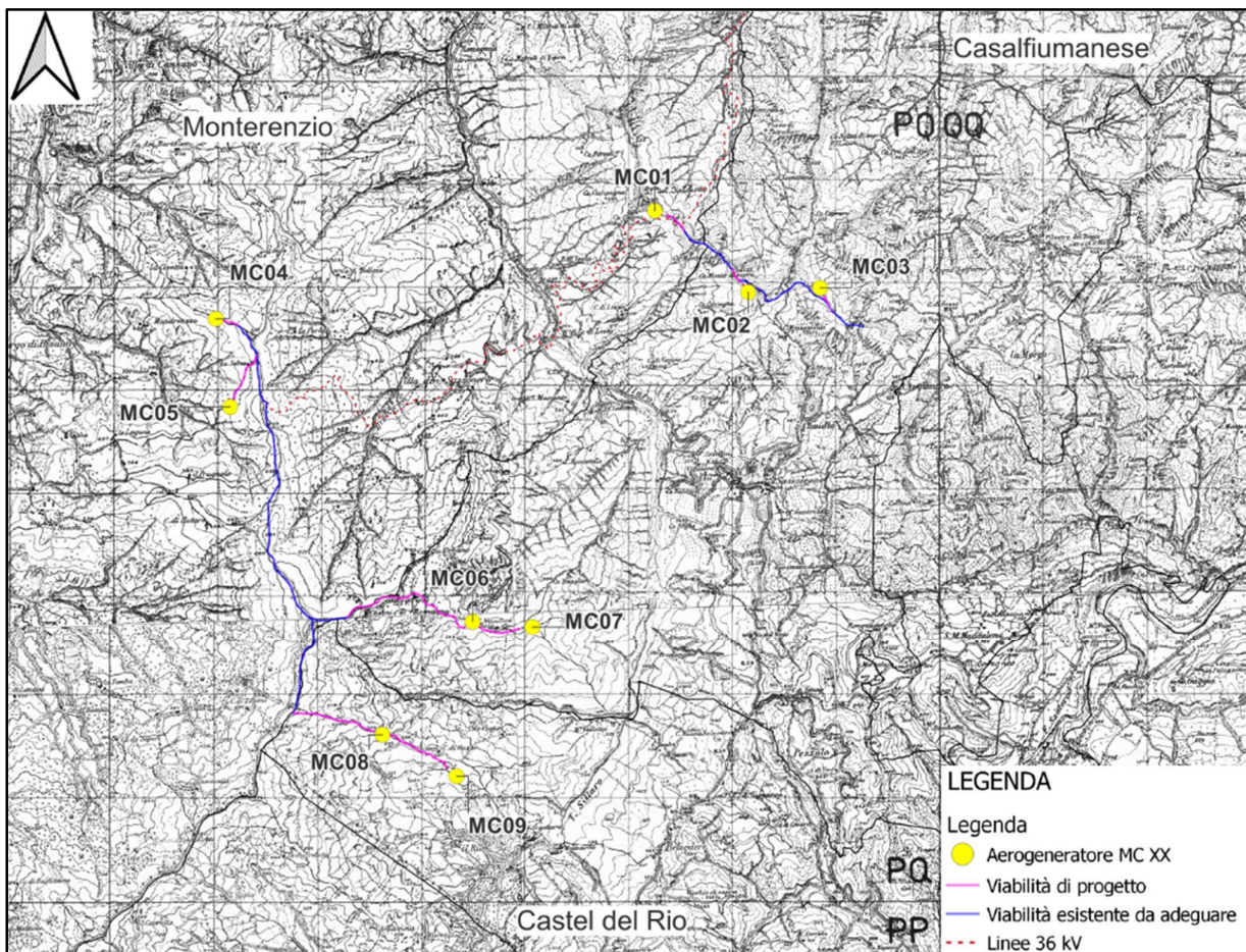
Figura 6.1: Layout d'impianto su carta IGM
