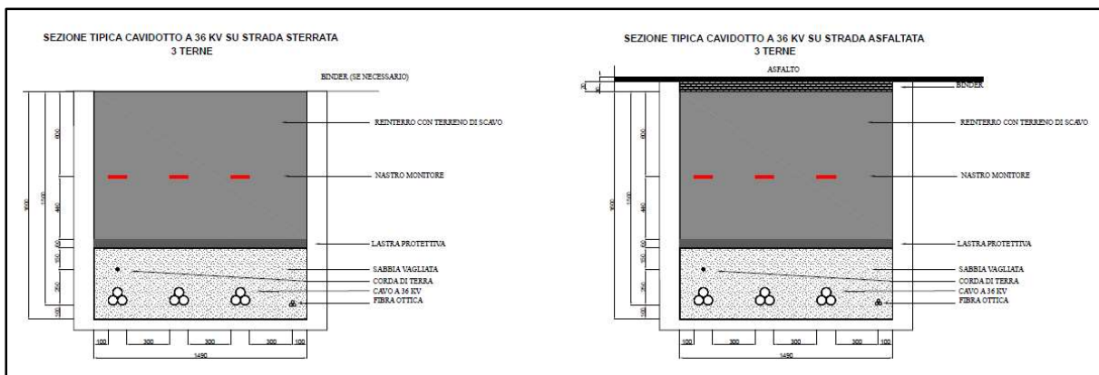
Figura 6.3.2.3: Sezioni tipiche delle trincee cavidotto per tre terne di cavi in parallelo
