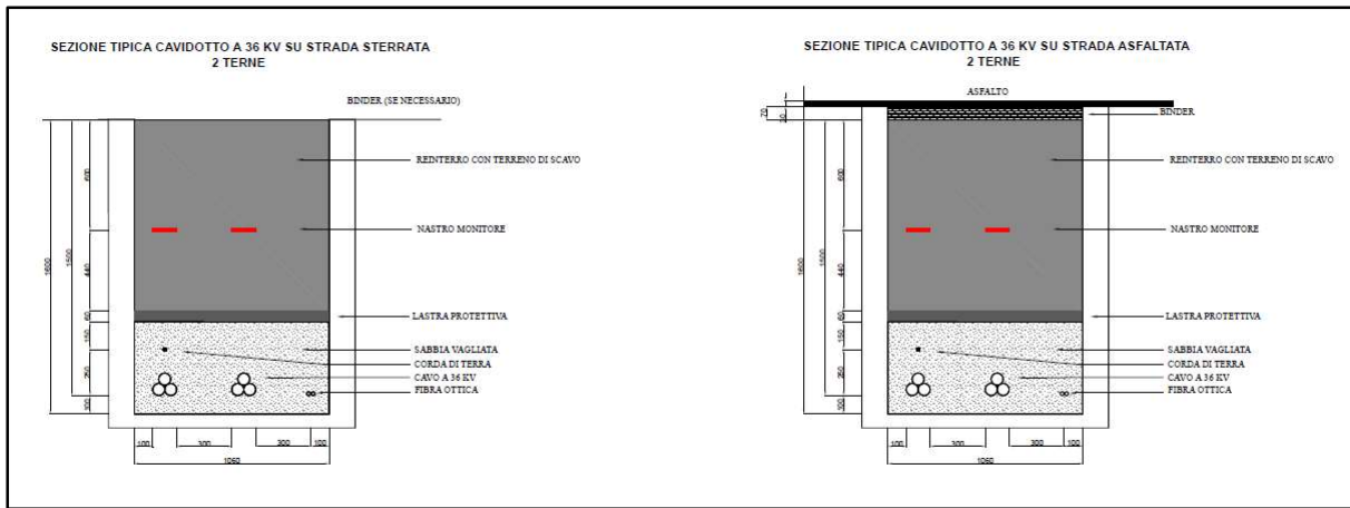
Figura 6.3.2.2: Sezioni tipiche delle trincee cavidotto per due terne di cavi in parallelo
