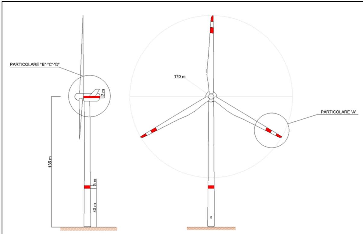
Figura 6.1.1: Profilo aerogeneratore SG170 – 6.0 MW
