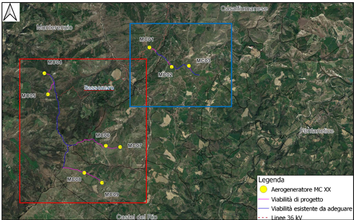
Figura 6.2: Layout d’impianto su ortofoto
