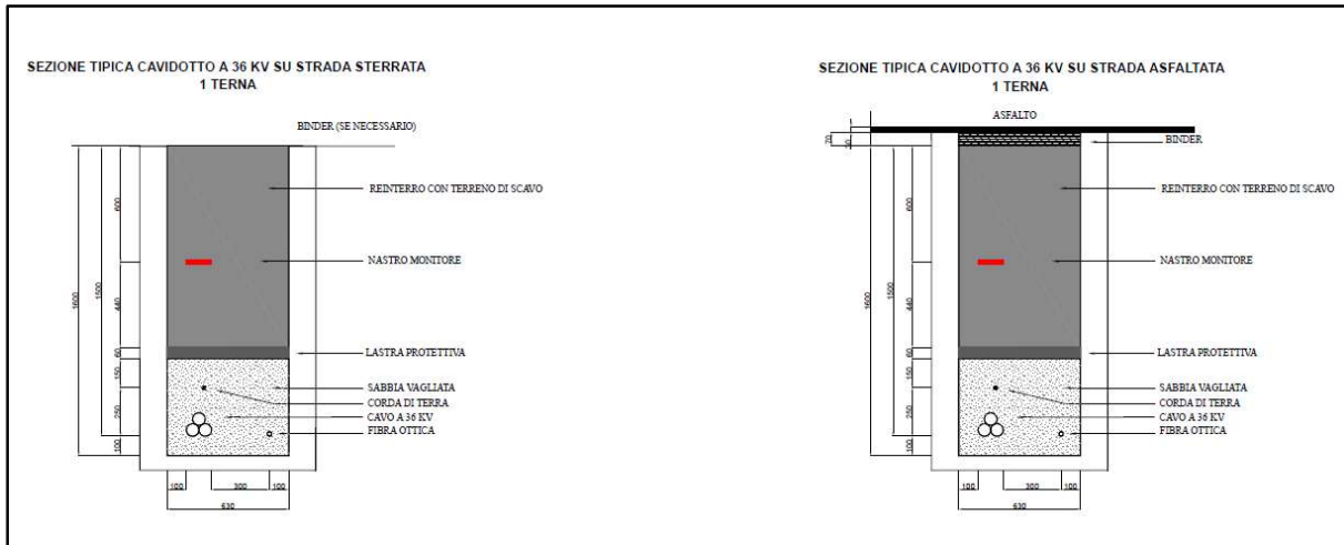
Figura 6.3.2.1: Sezioni tipiche delle trincee cavidotto per una terna di cavi in parallelo
