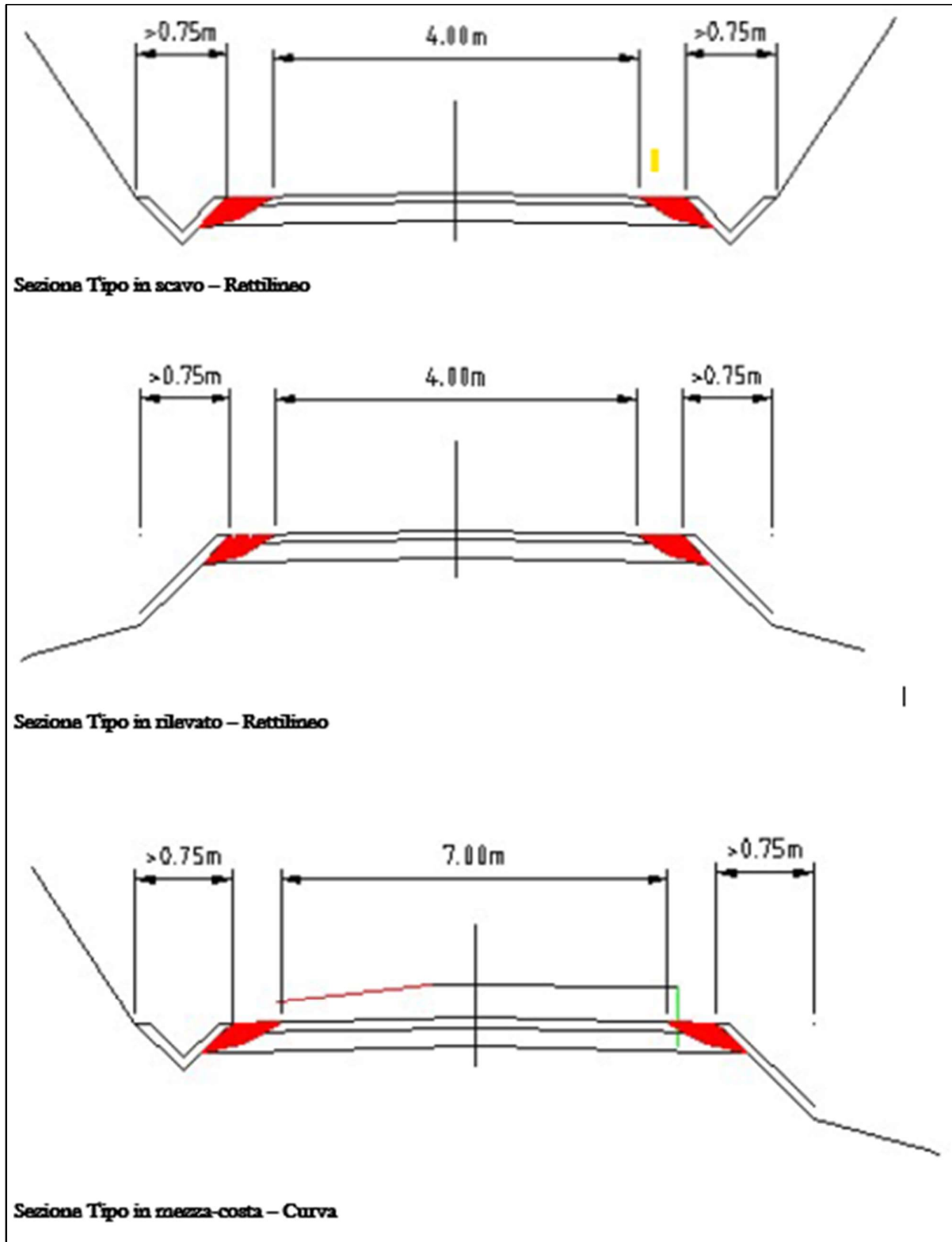
Figura 6.2.1: Sezioni tipo viabilità parco eolico
