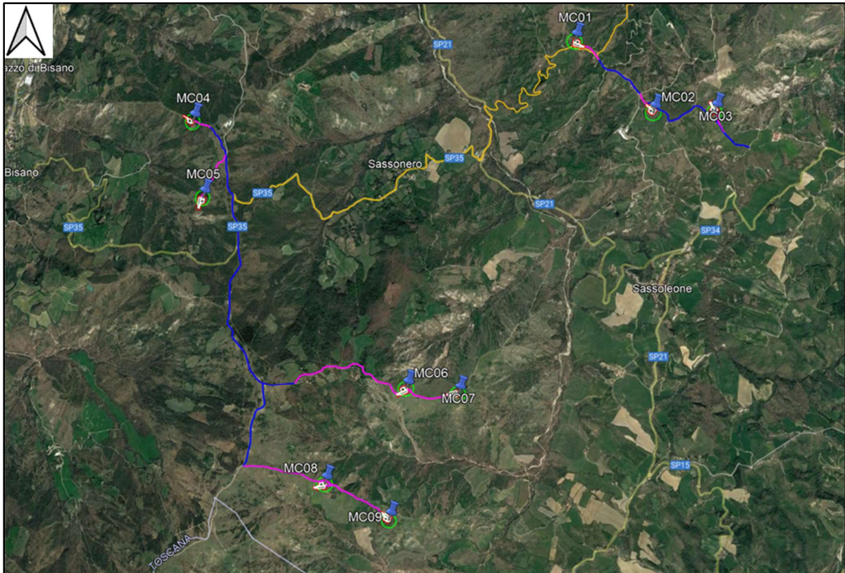
Figura 6.6: Layout d'impianto con sistema di viabilità esistente (linee blu) e di progetto (linee magenta) su immagine satellitare
