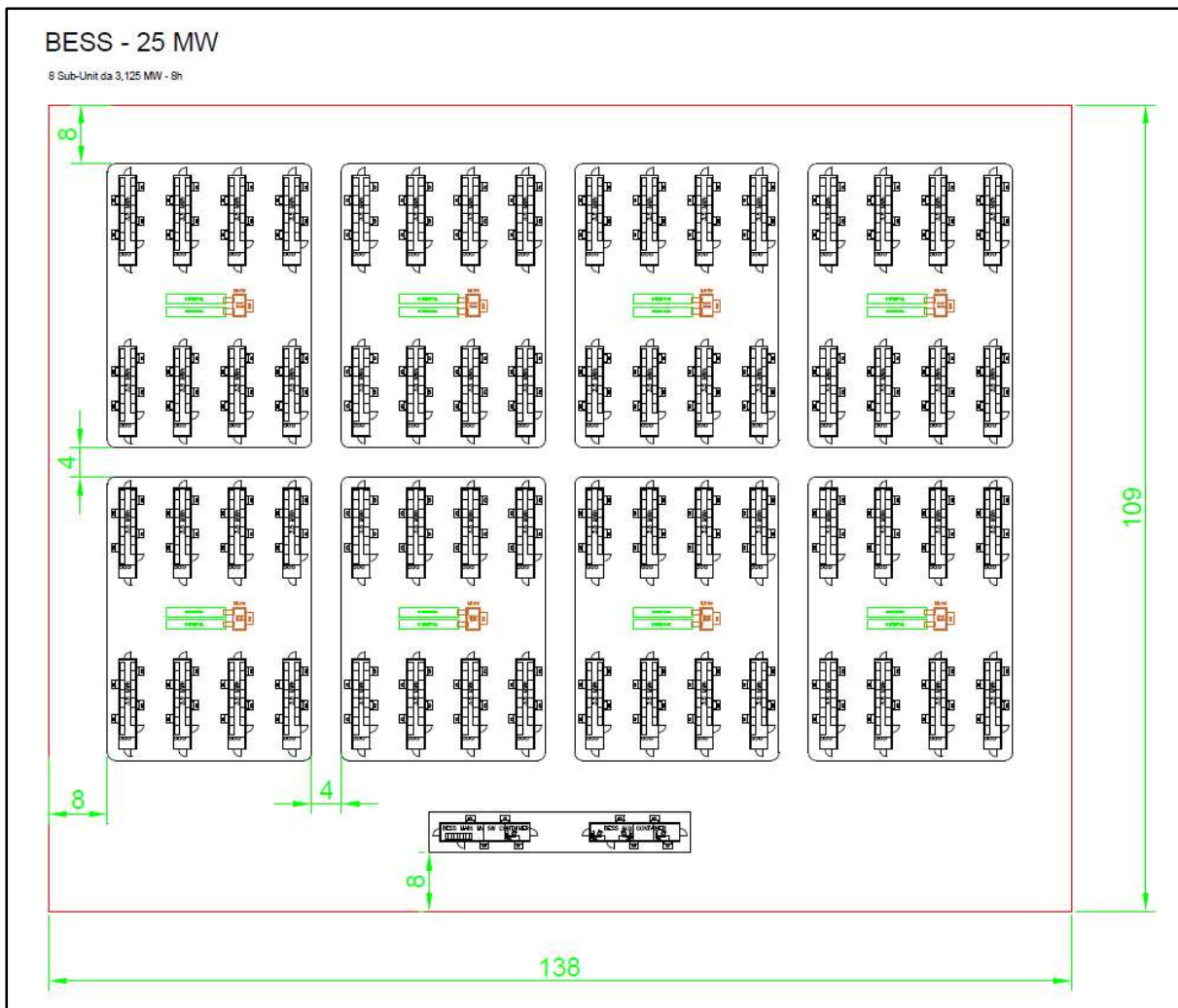
Figura 6.3.3.1: Configurazione BESS di potenza 25 MWp
