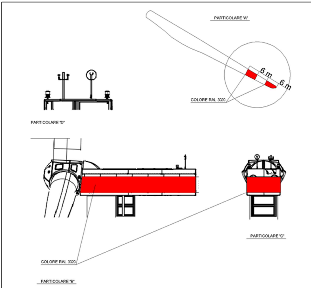
Figura 6.1.2: Particolari aerogeneratore SG170 – 6.0 MW di cui alla Figura 6.1.1
