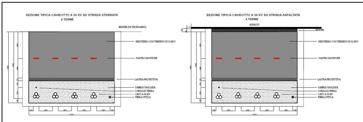
Figura 6.3.2.4: Sezioni tipiche delle trincee cavidotto per quattro terne di cavi in parallelo
