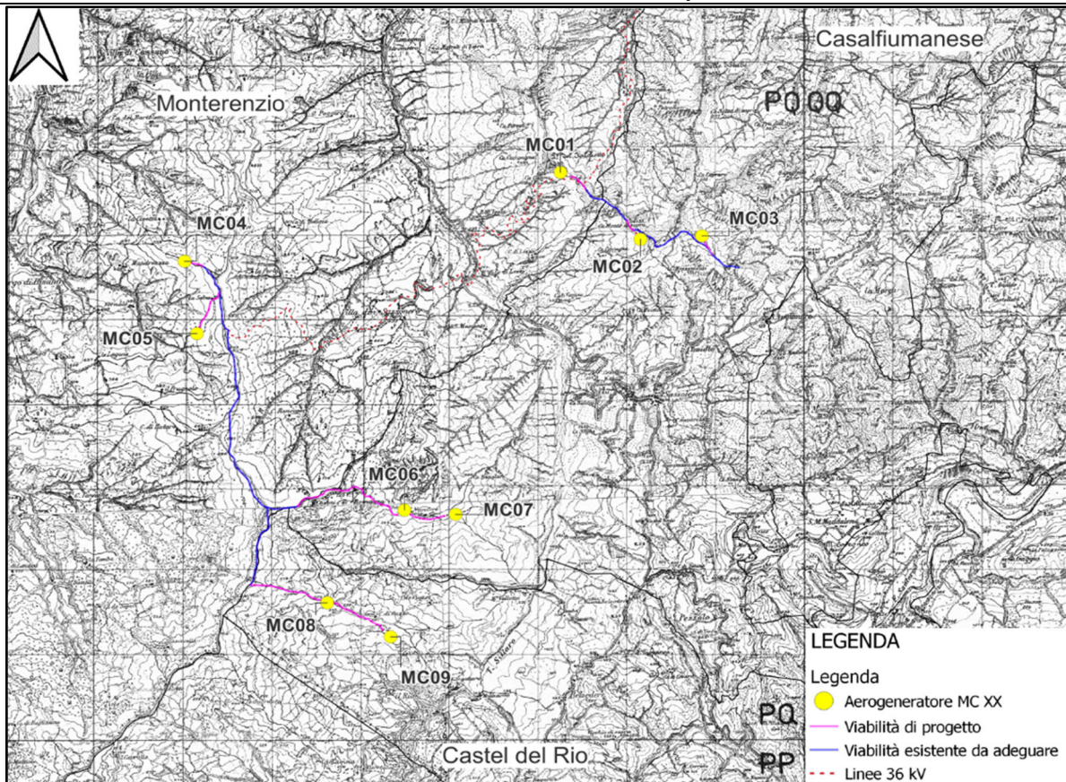
Figura 2.1: Layout d'impianto su carta IGM
