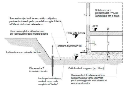
PARTICOLARI SCAVO E PLATEA FONDAZIONE
