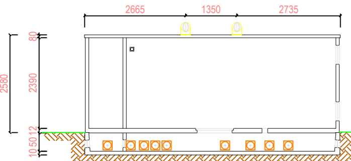
SEZIONE A-A
