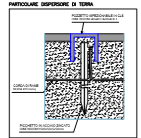
PARTICOLARE PICCHETTO DISPENSORE
