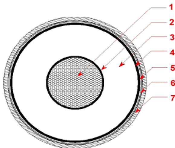
Figura 3 – Sezione del cavo
