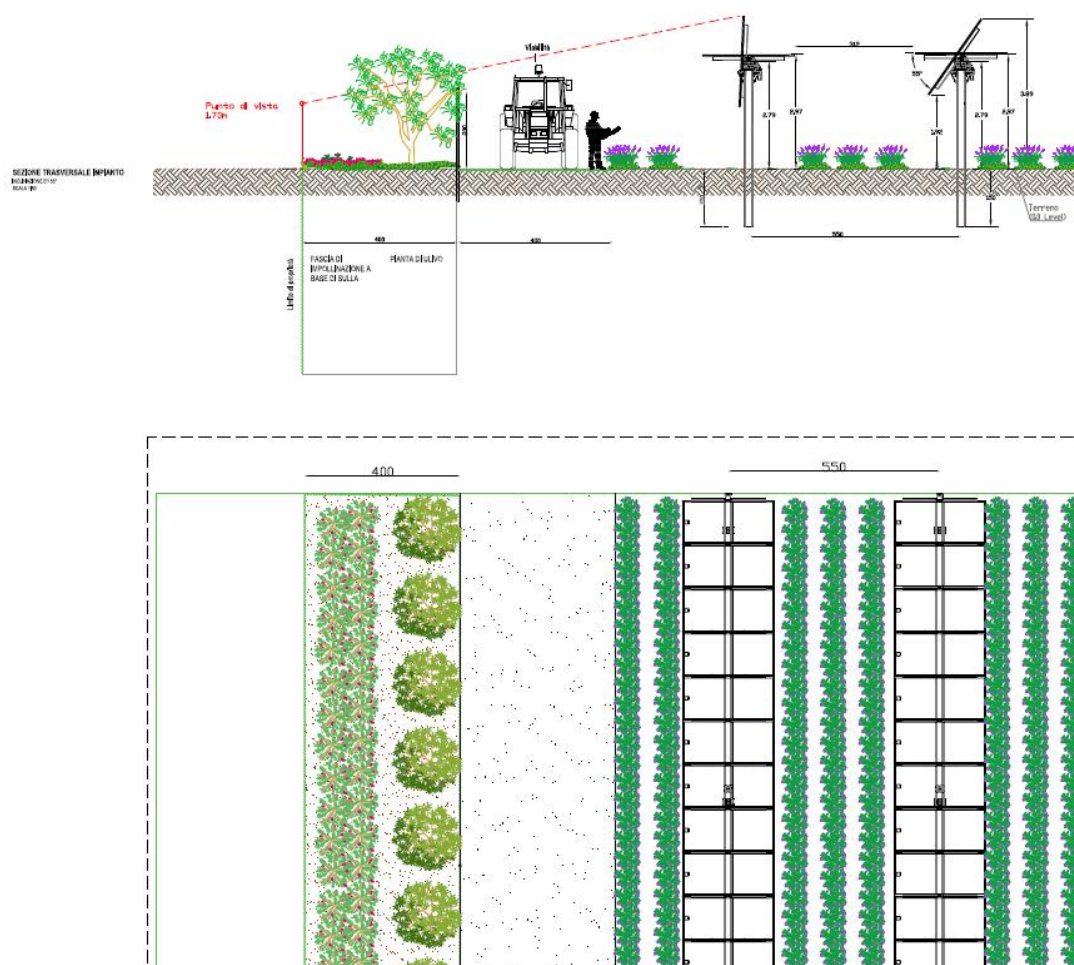
Figura 2 – Vista in sezione ed in pianta del campo agrofotovoltaico con la coltivazione di lavanda (VZYY142_ElaboratoGrafico_4.2.9_26). La soluzione adottata prevede un tracker alto (altezza in corrispondenza dell'asse di rotazione pari a 279 cm) ed interasse di 5,5 m
