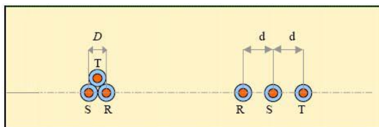
Figura 4 - Modalità di posa
