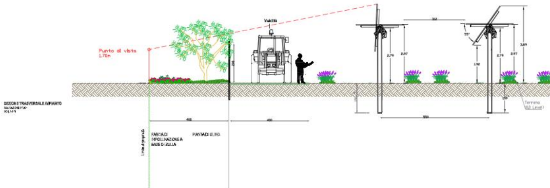
Figura 18 – Vista in sezione ed in pianta del campo agrovoltaco con la coltivazione di lavanda (VZYY142_ElaboratoGrafico_4.2.9_26).
