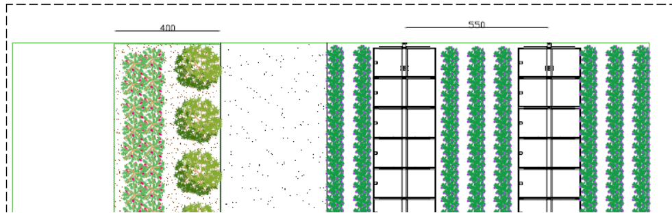
Figura 18 – Vista in sezione ed in pianta del campo agrovoltaco con la coltivazione di lavanda (VZYY142_ElaboratoGrafico_4.2.9_26).
