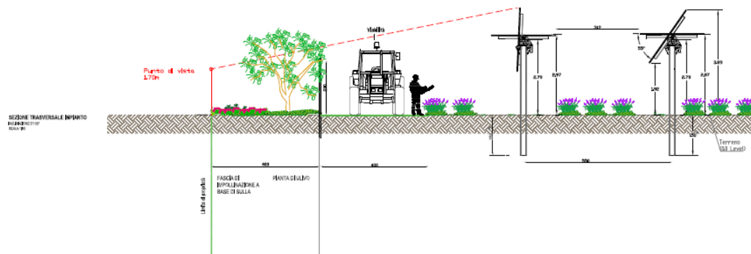
Figura 8 – Sezione tipo della soluzione adottata con tracker alto (altezza in corrispondenza dell'asse di rotazione pari a 279 cm) ed interasse di 5,5 m
