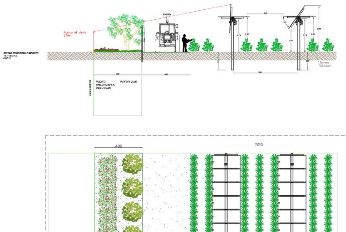
Figura 20 – Vista in sezione ed in pianta del campo agrovoltaico con la coltivazione di rosmarino (VZYY142_ElaboratoGrafico_4.2.9_26).
