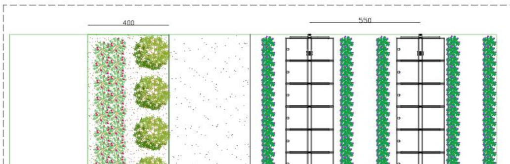
Figura 19 – Vista in sezione ed in pianta del campo agrovoltaco con la coltivazione di lavandino (VZYY142_ElaboratoGrafico_4.2.9_26).
