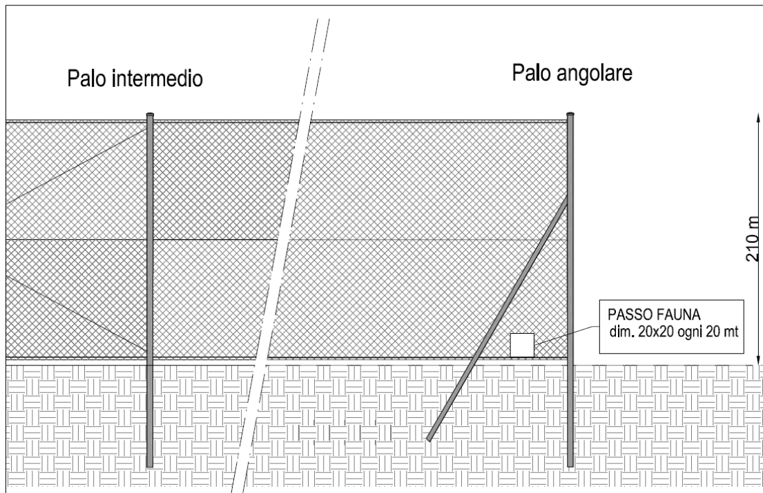
Figura 27 - Particolare costruttivo della recinzione perimetrale come da elaborato VZYY142_ElaboratoGrafico_4.2.9_10
