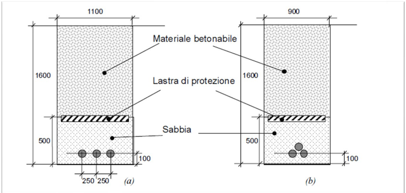
Figura 15: schermatura cavi elettrici interrati
