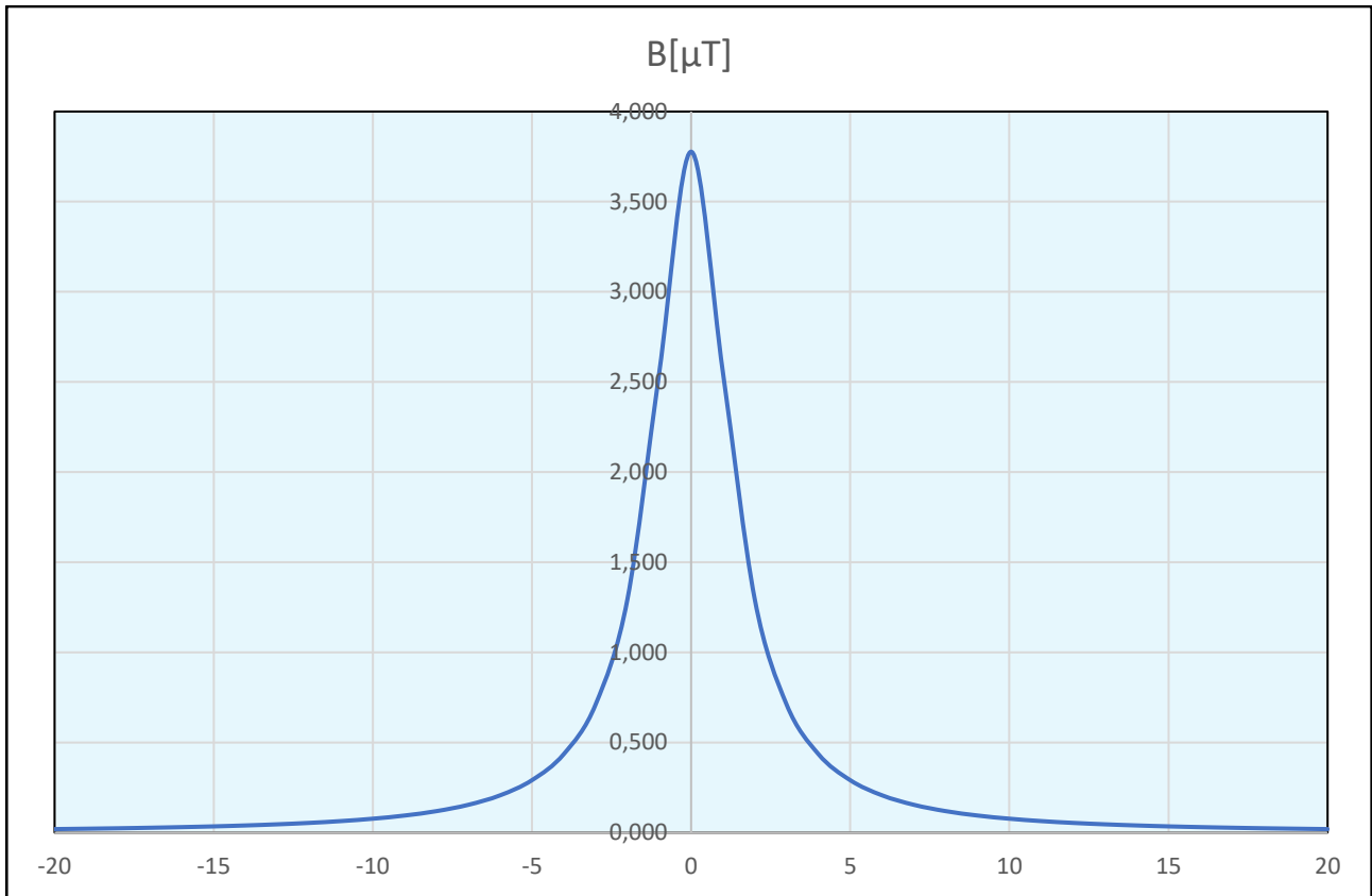
Figura 9: Induzione magnetica generata durante l'esercizio dalla dorsale 36 kV da 630 mm 2 di collegamento con la Stazione Elettrica di Trasformazione Terna; I = 425 A circa, profondità di posa 1,40 m
