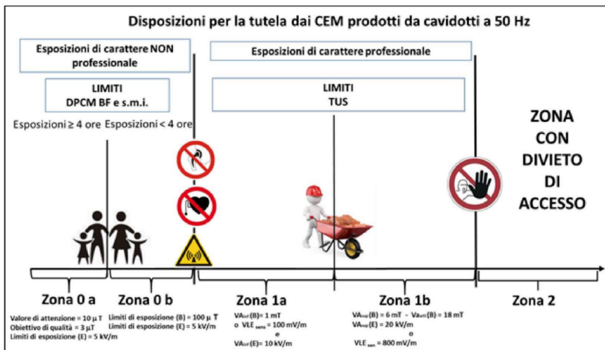
Figura 10: Misure di prevenzione e protezione per la tutela dai CEM prodotti da cavidotti a 50 Hz
