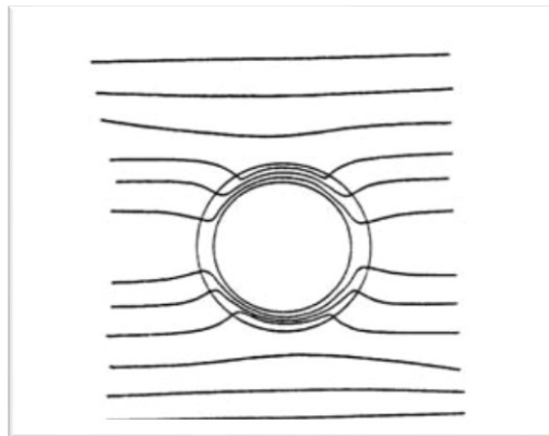
Figura 14: andamento qualitativo della deformazione delle linee di forza di un campo magnetico uniforme per effetto di un nucleo in materiale ferromagnetico
