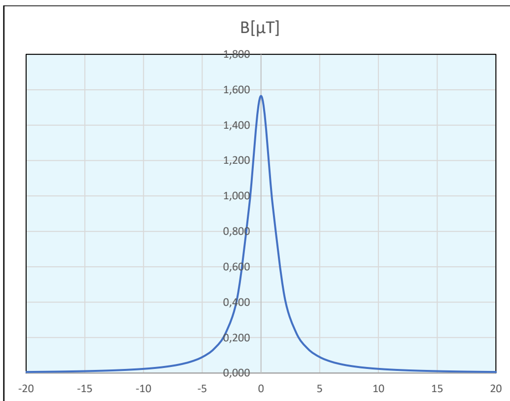
Figura 8: Induzione magnetica generata durante l'esercizio dalla linea a 36 kV n° 3 da 240 mm 2 valutata ai sensi della Norma CEI 211-4 – Guida ai metodi di calcolo dei campi elettrici e magnetici generati da linee elettriche. Fasi disposte a trifoglio, intensità di corrente I = 161 A, profondità di posa 1,20 m
