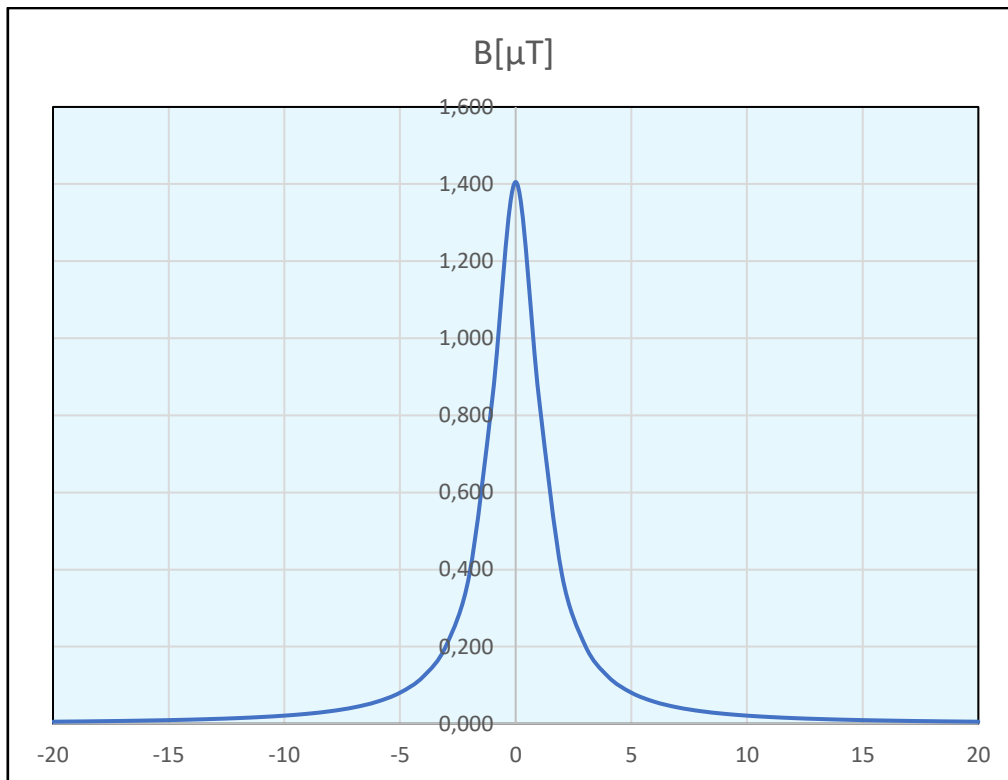
Figura 7: Induzione magnetica generata durante l'esercizio dalla linea a 36 kV n° 2 da 185 mm 2 valutata ai sensi della Norma CEI 211-4 – Guida ai metodi di calcolo dei campi elettrici e magnetici generati da linee elettriche. Fasi disposte a trifoglio, intensità di corrente I = 152 A, profondità di posa 1,20 m
