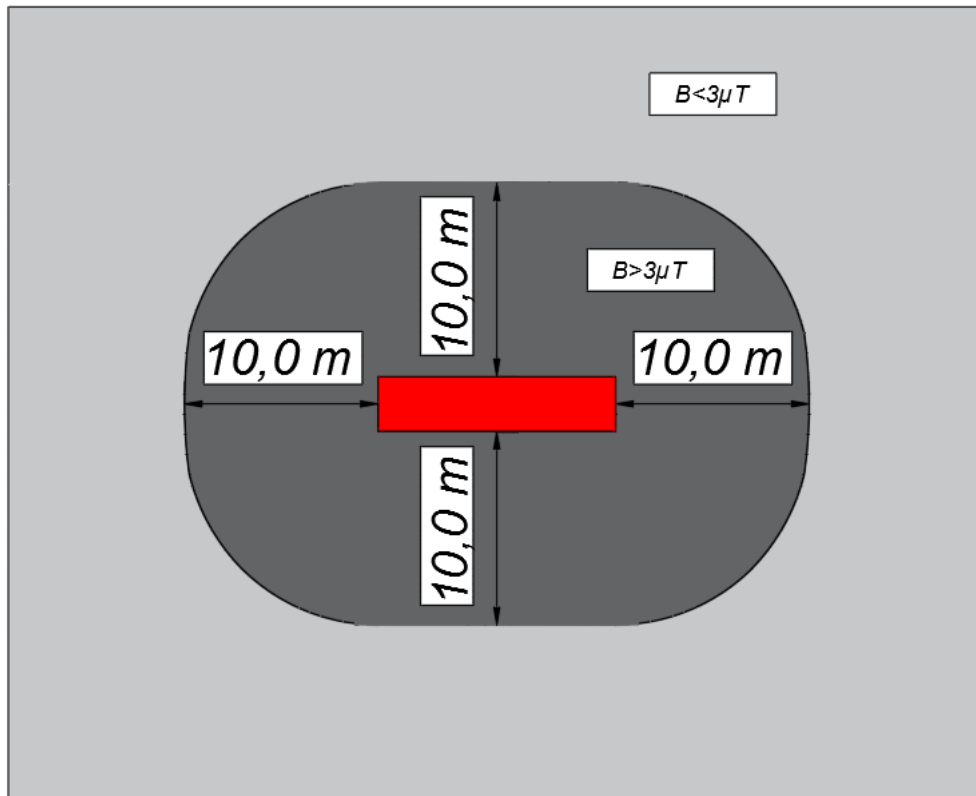
Figura 4: Distanza di prima approssimazione cabina elettrica equipaggiata con trasformatori da 5000 kVA
