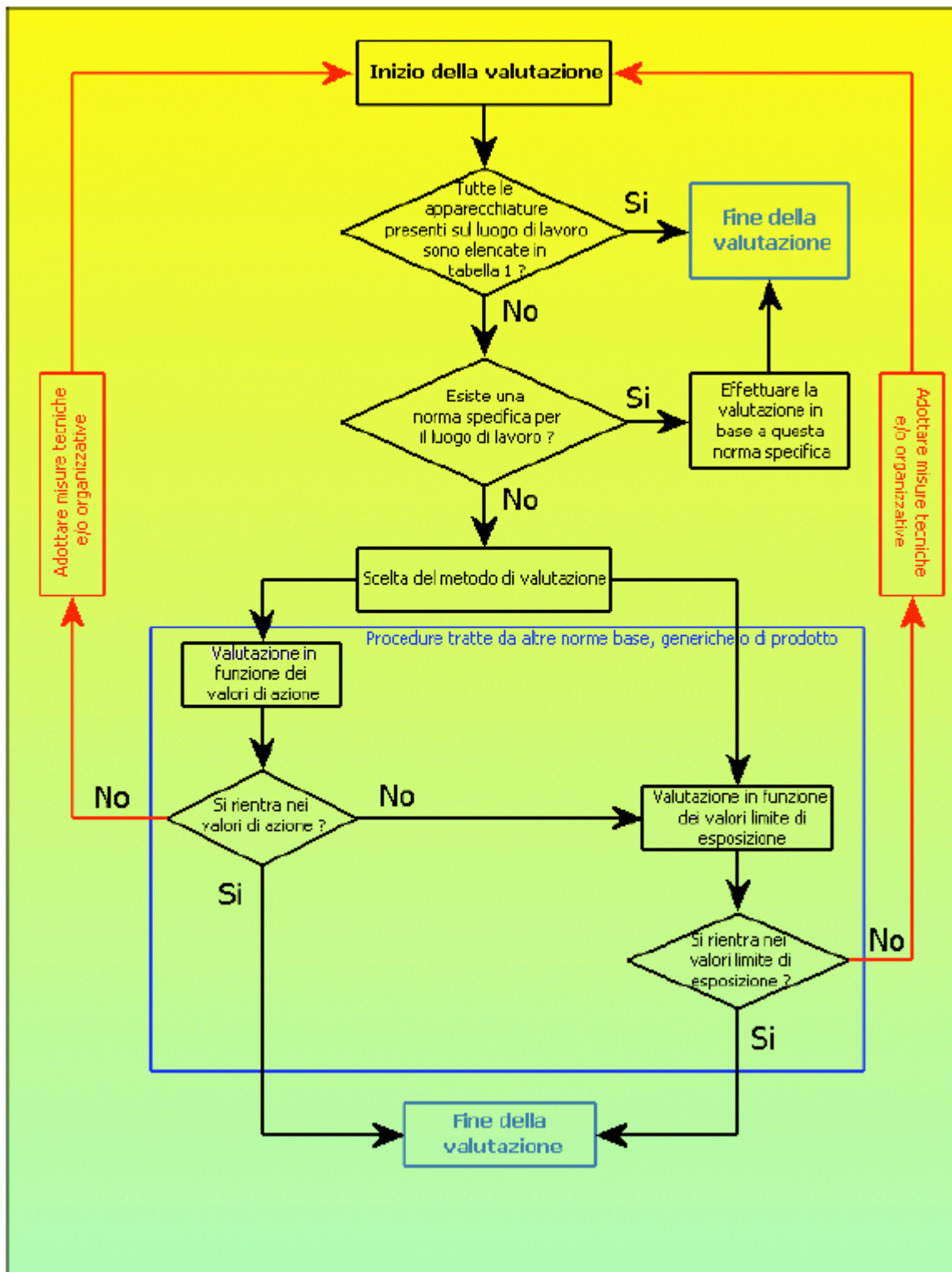
Figura 11: Diagramma di flusso del processo di valutazione del rischio elettromagnetico (CEI EN 50499)
