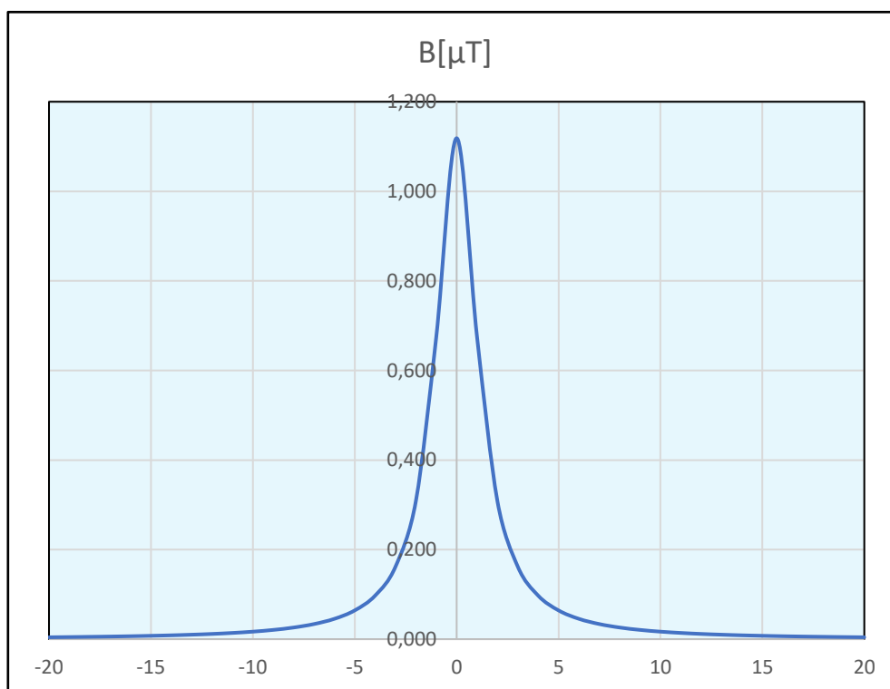
Figura 6: Induzione magnetica generata durante l'esercizio dalla linea a 36 kV n° 1 da 185 mm 2 valutata ai sensi della Norma CEI 211-4 – Guida ai metodi di calcolo dei campi elettrici e magnetici generati da linee elettriche. Fasi disposte a trifoglio, intensità di corrente I = 121 A, profondità di posa 1,20 m
