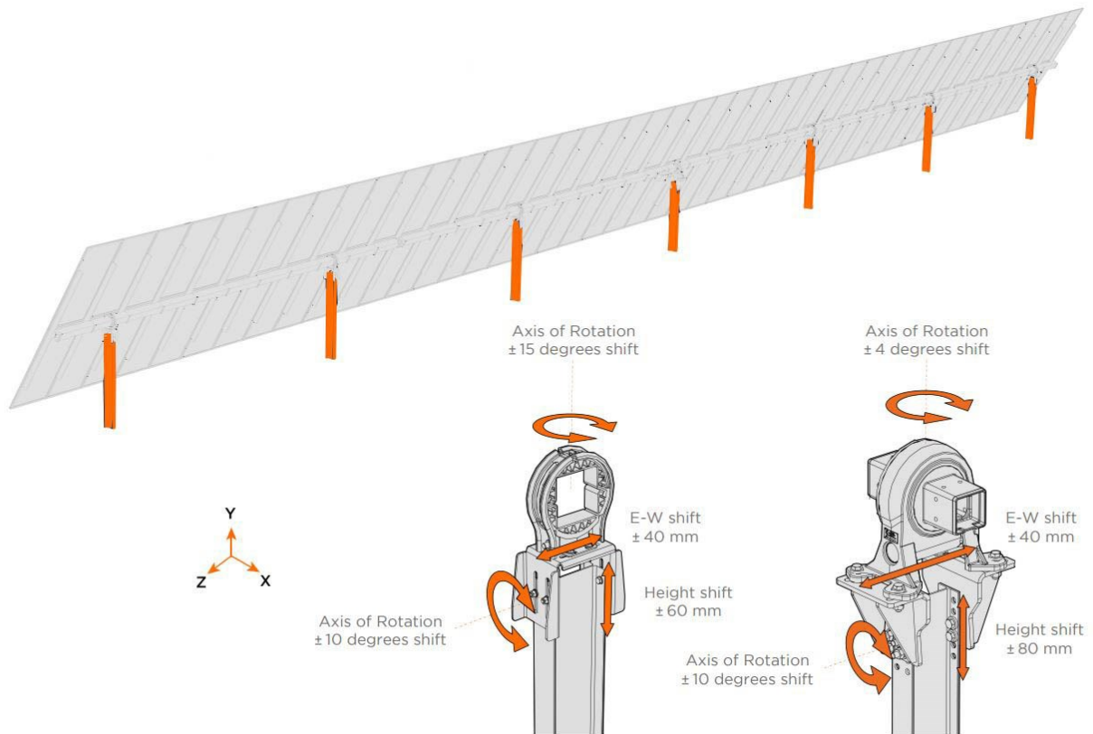
Figura 2 - Montaggio strutture tracker
