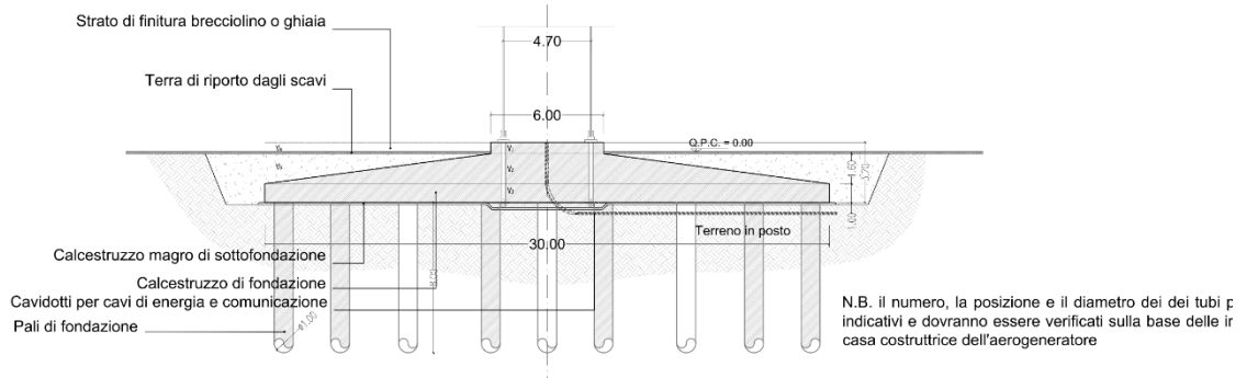
Figura 1 - Pianta e vista della fondazione dell'aerogeneratore nella configurazione provvista di pali
