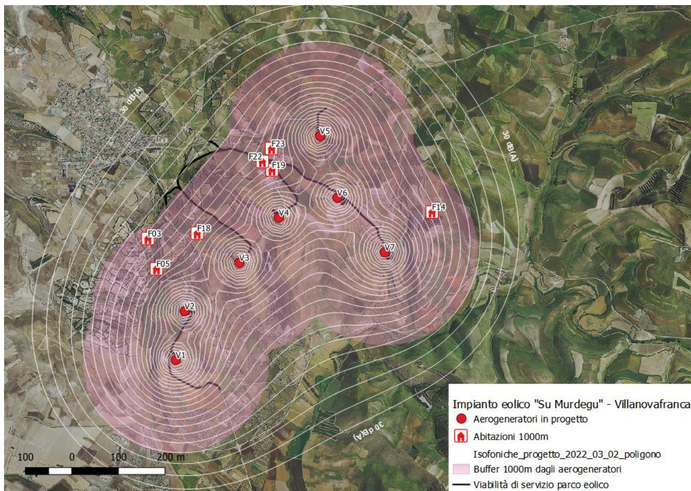
Figura 2.5 – Campo sonoro generato dall'impianto. Si noti come l'isofonica dei 30 dBA sia attestata ad una distanza indicativa di 1.200 m dalle postazioni eoliche in progetto
