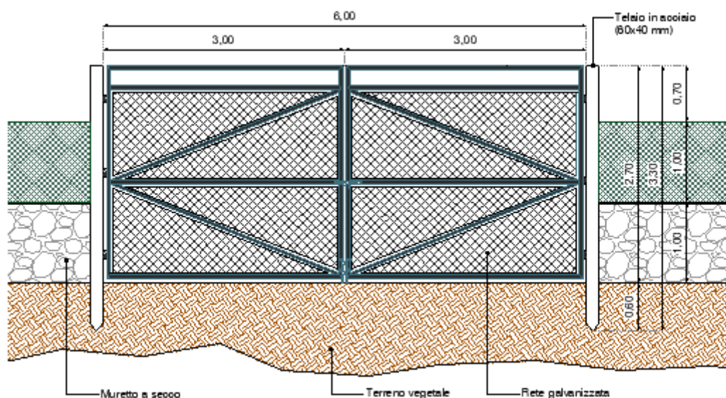
Figura 2 - Cannello d'ingresso
