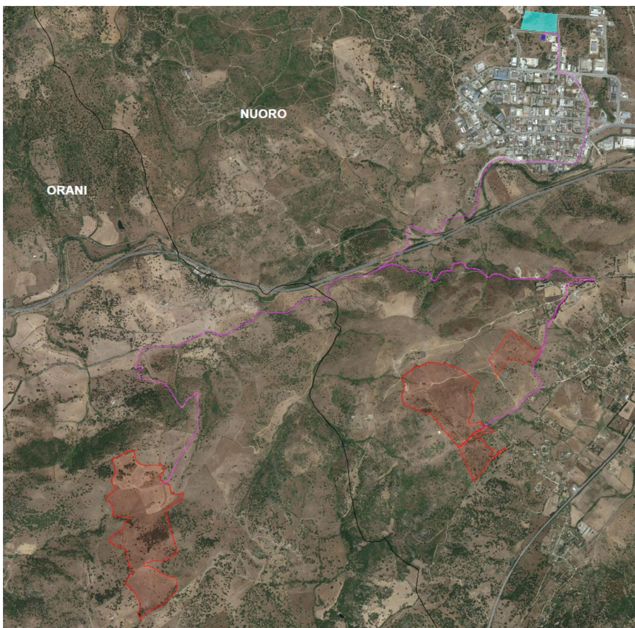
Figura 4 - Area impianto FV evidenziata in rosso, stazione elettrica RTN in ciano
