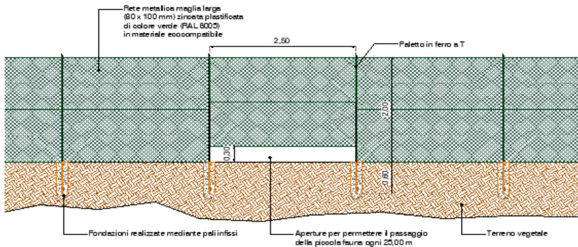
Figura 1 - Prospetto recinzione
