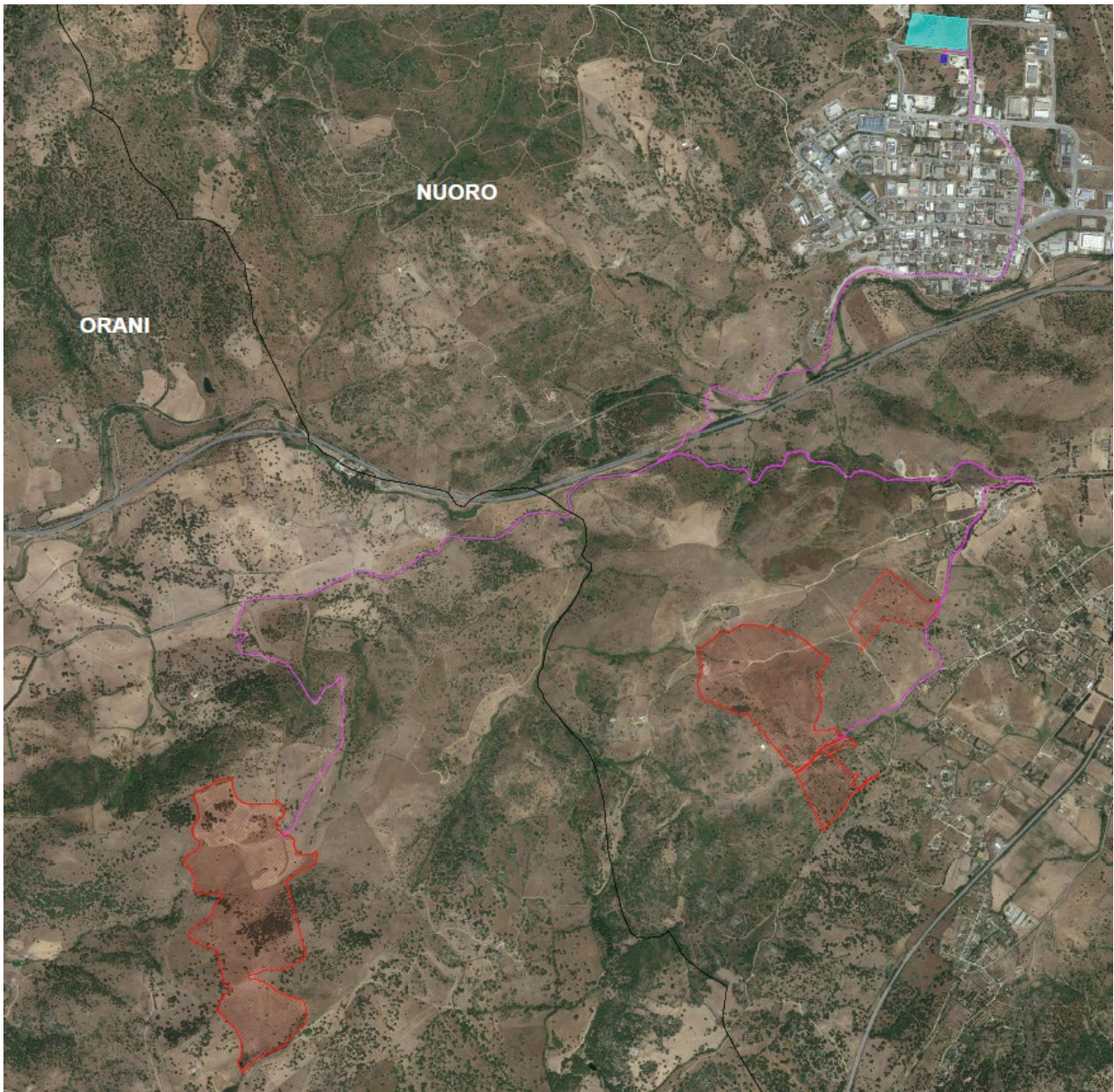
Figura 1 - Impianto FV in rosso
