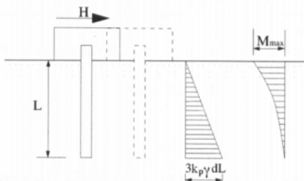
Figura 17 - Resistenza limite del terreno di un palo impedito di ruotare a testa
