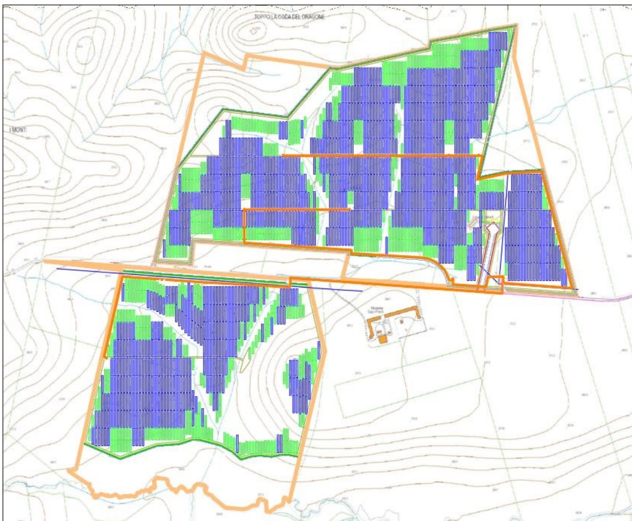
Figura 3 - Layout impianto
