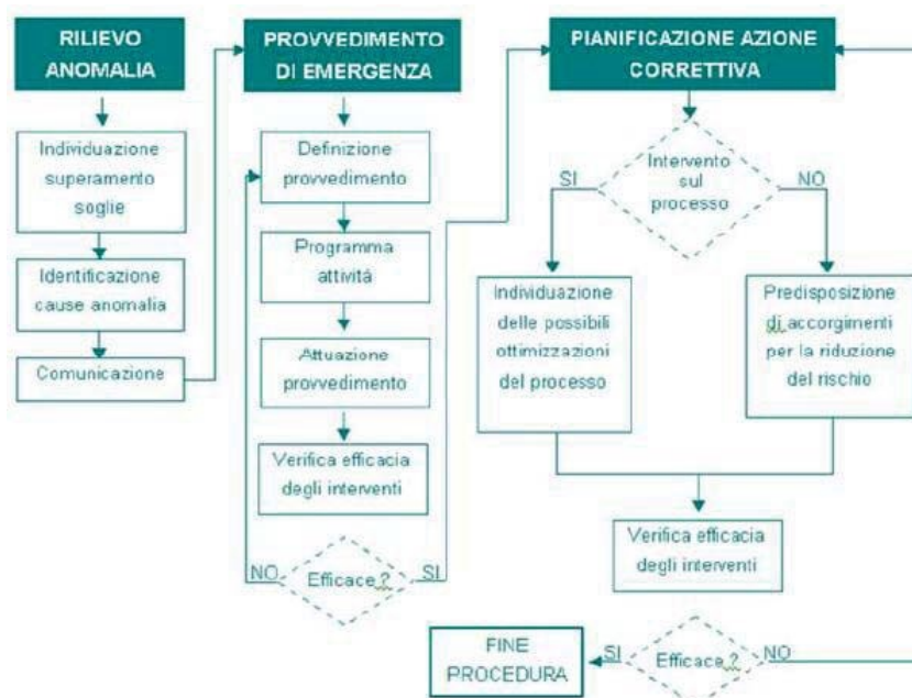
Figura 4: Processo di gestione delle anomalie.
