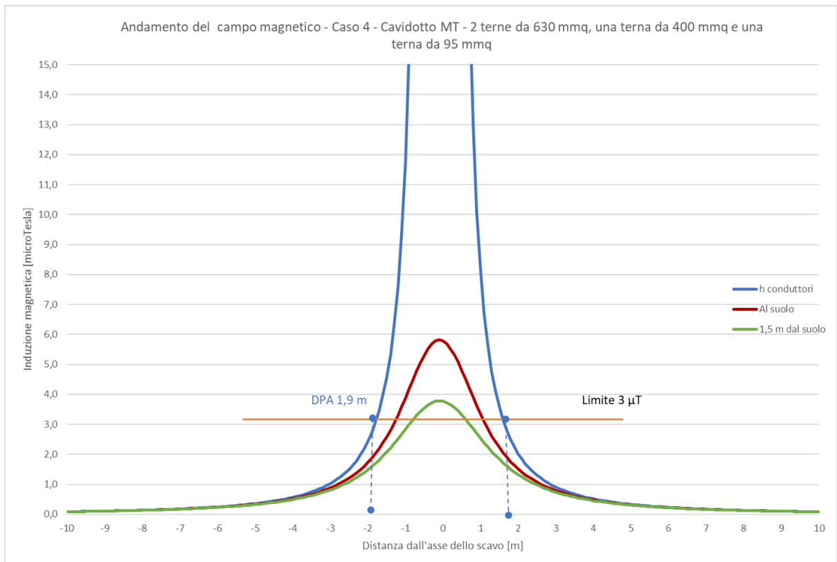
Figura 4: Andamento del campo magnetico in funzione della distanza dall'asse dei conduttori in forma grafica relativa CASO 4.
