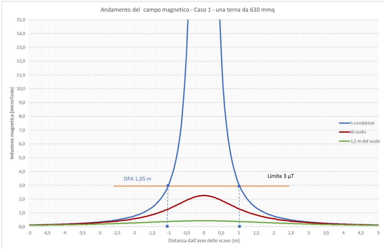
Figura 1: Andamento del campo magnetico in funzione della distanza dall'asse dei conduttori in forma grafica relativa CASO 1.
