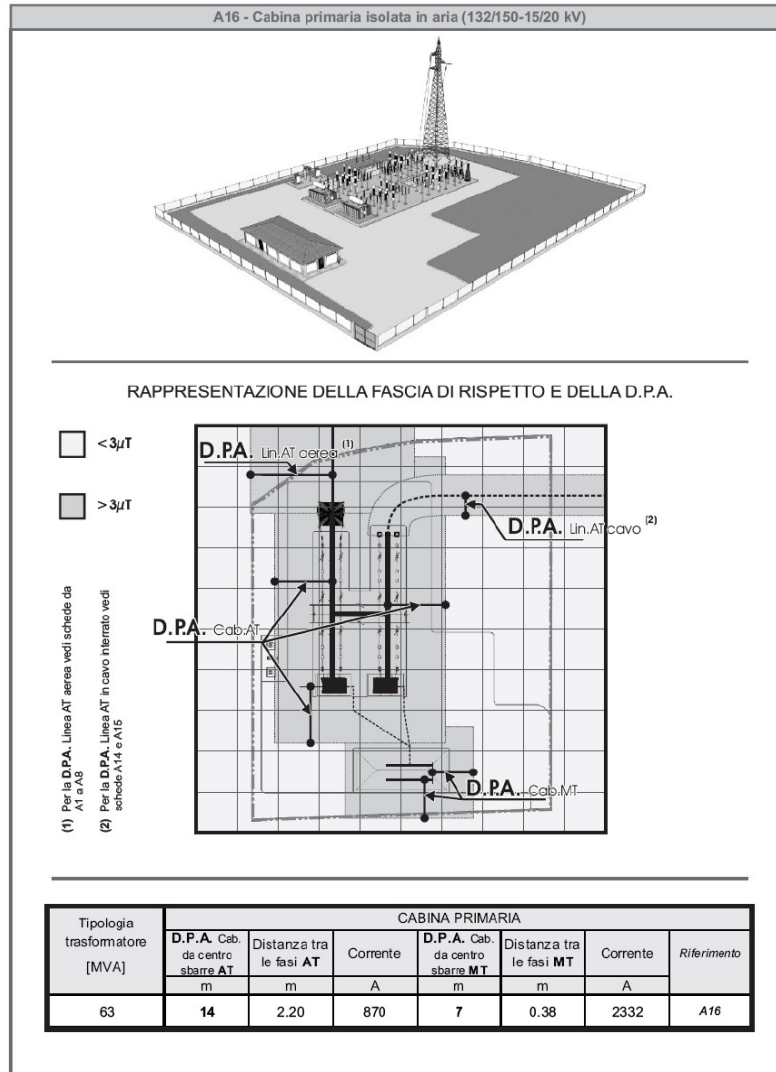
Figura 5: Esempio di fasce di rispetto relative ad una cabina primaria
