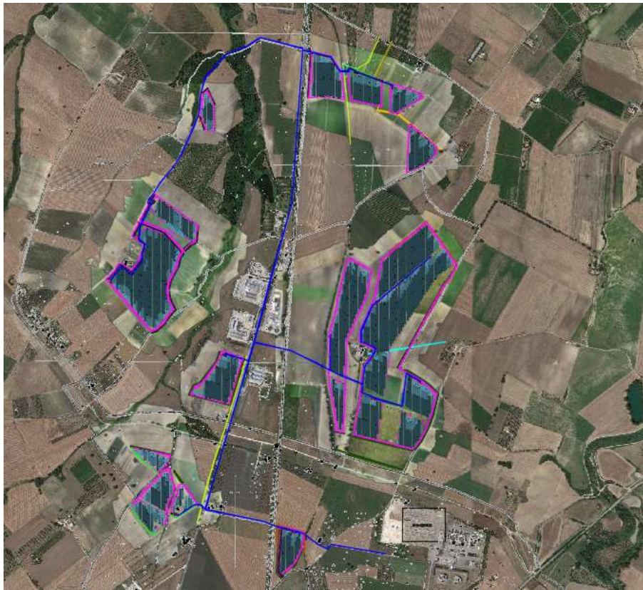
4- Layout di progetto
