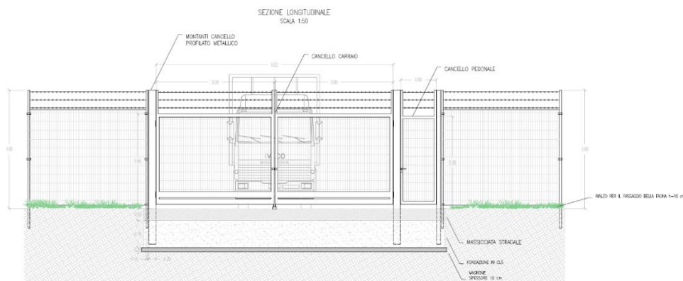
Figura 2.7: Particolare accesso
