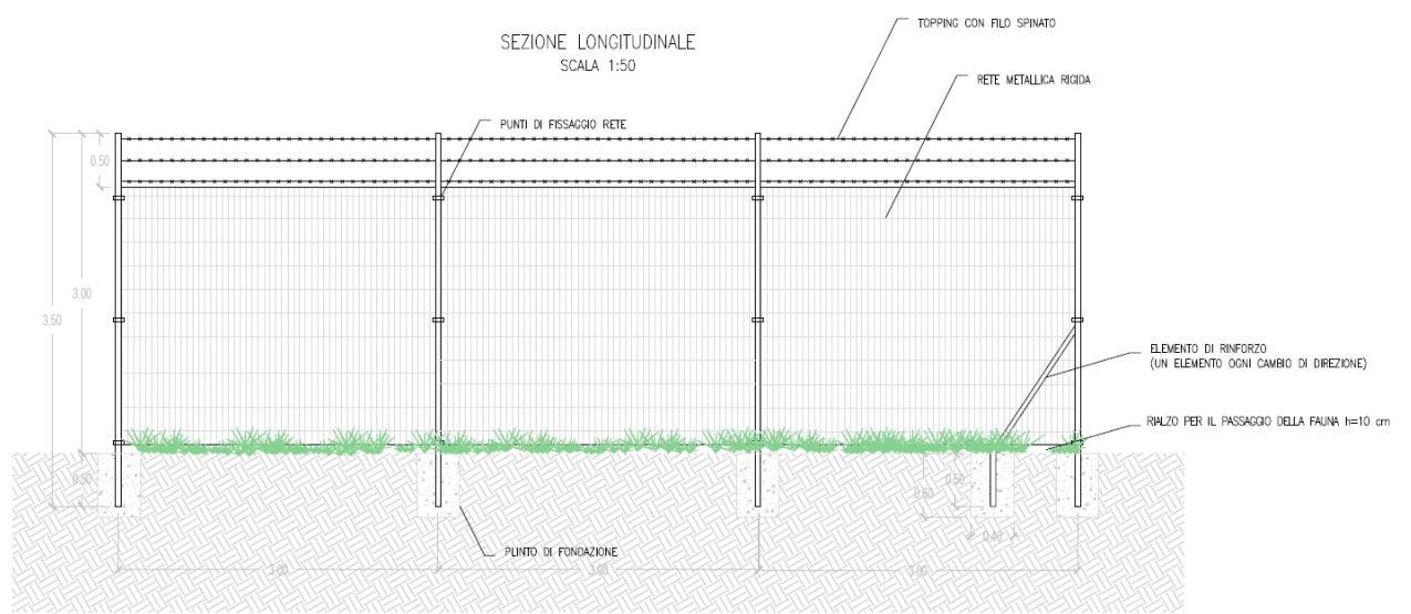
Figura 2.6: Particolare recinzione
