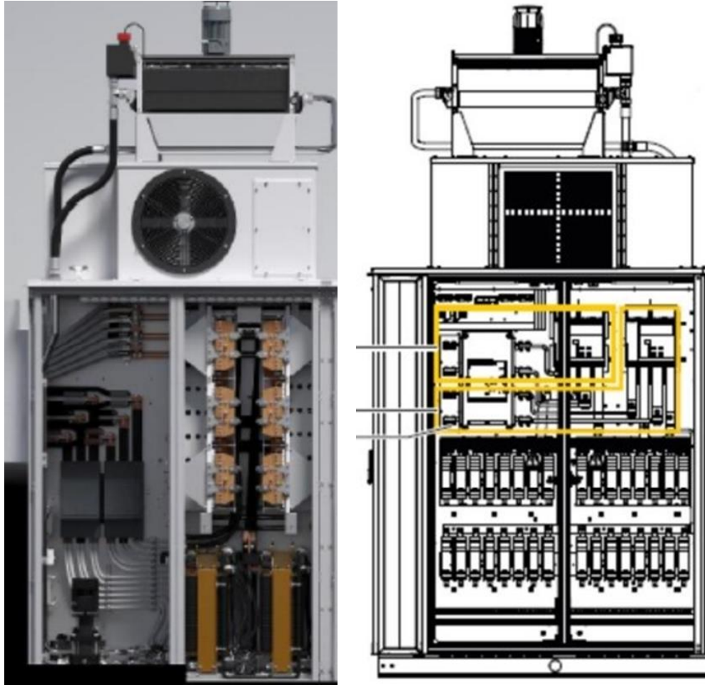
Figura 2.3: Datasheet inverter centralizzato
