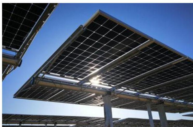
Figura 2.5: Particolare strutture di sostegno moduli
