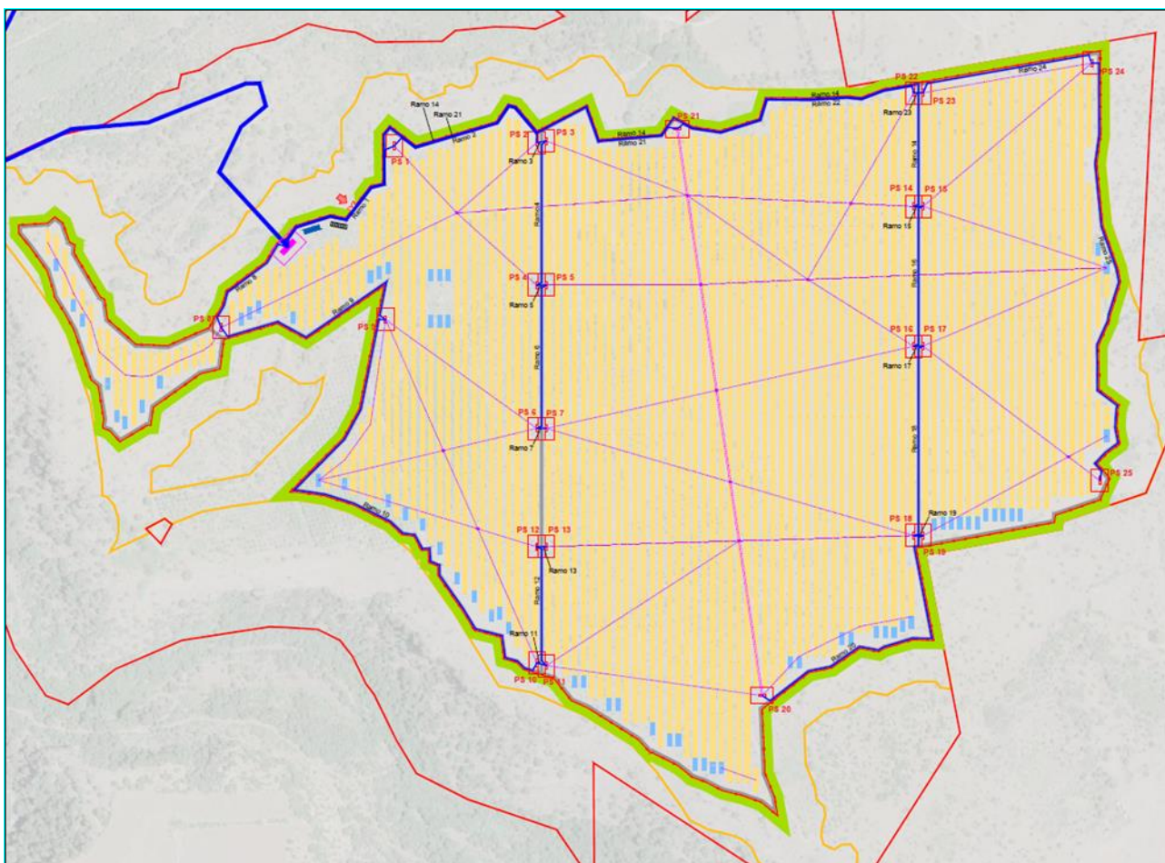
Figura 2.10: Stato di progetto dell'area dell'impianto
