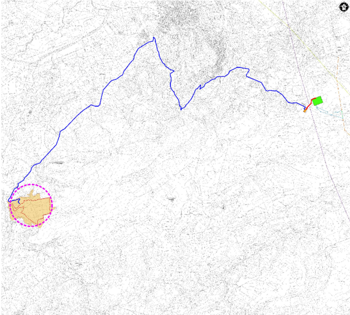
Figura 5.1: Collegamento MT alla Stazione di utenza
