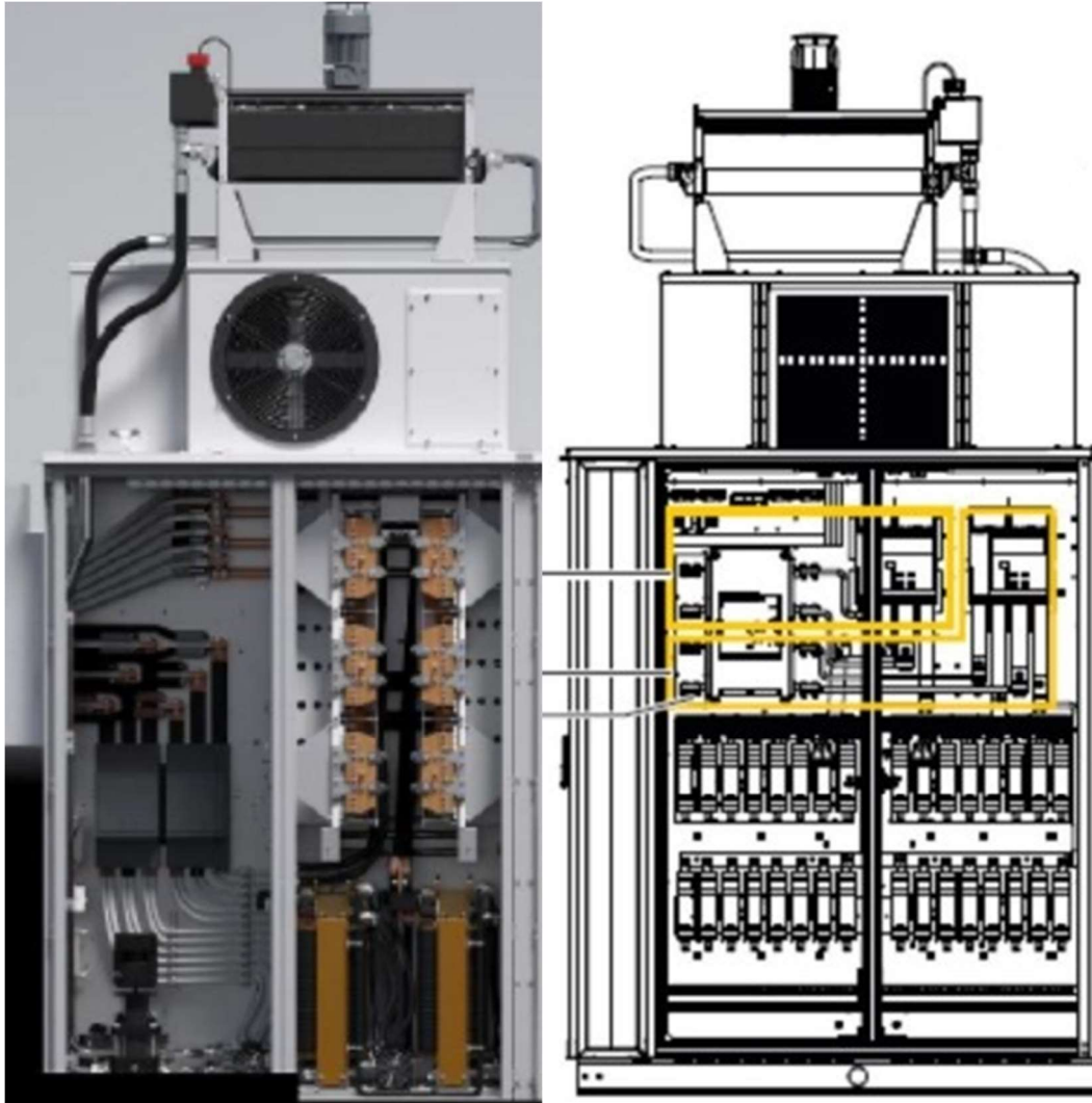
Figura 4.6 – Modulo inverter centralizzato tipo SUNWAY TG 1800 1500V TE.
