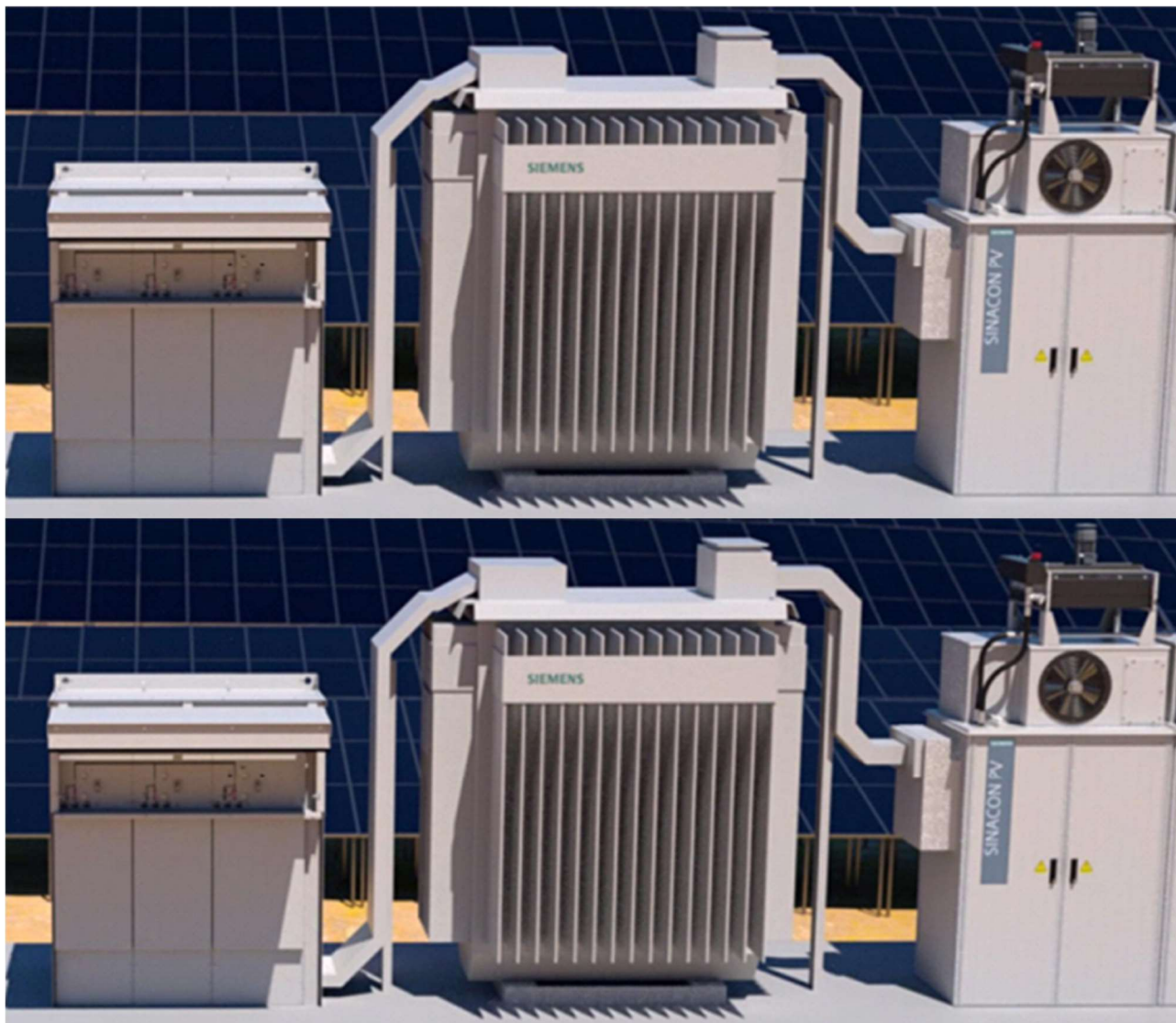
Figura 4.8 – Power Station tipo: SIEMENS DANACON 2000 PV con inverter centralizzato.
