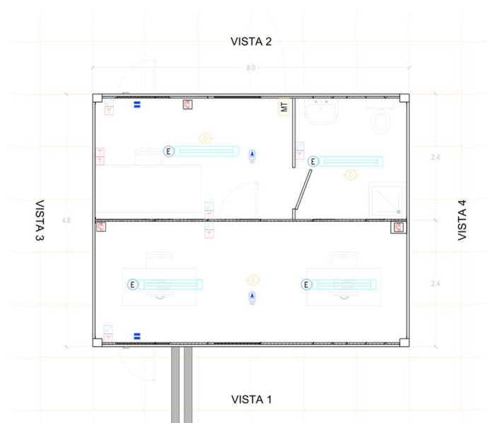
Figura 4.3 - Posizionamento plafoniere Cabina Uffici.
