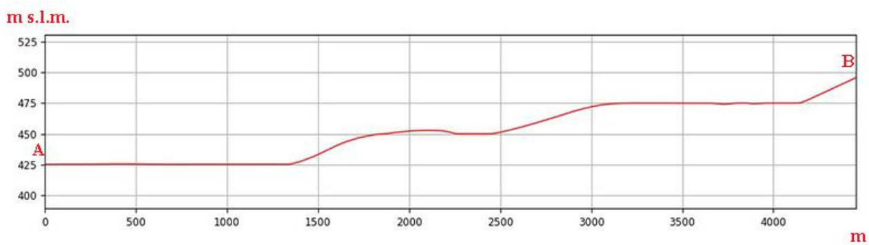
Sezione morfologica del terreno- Punto di presa n°14
