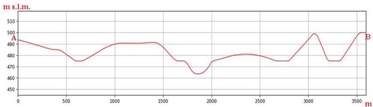
Sezione morfologica del terreno- Punto di presa n°10
