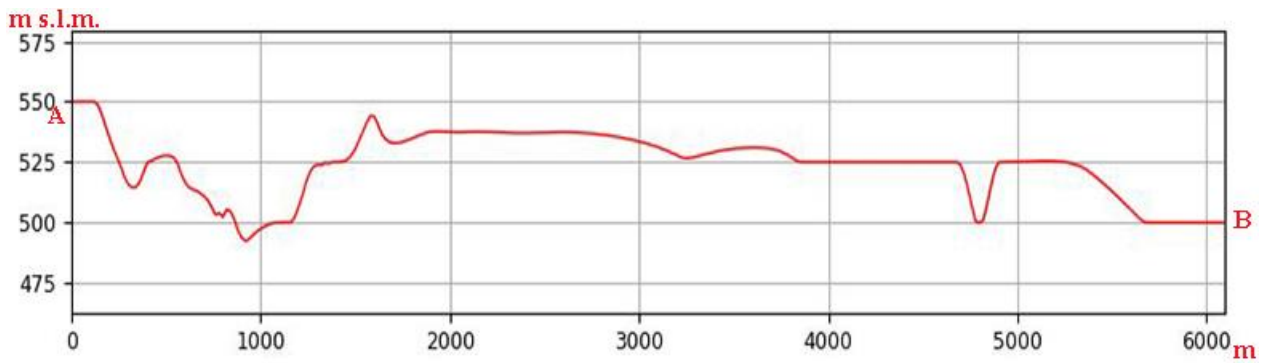
Sezione morfologica del terreno- Punto di presa n°5
