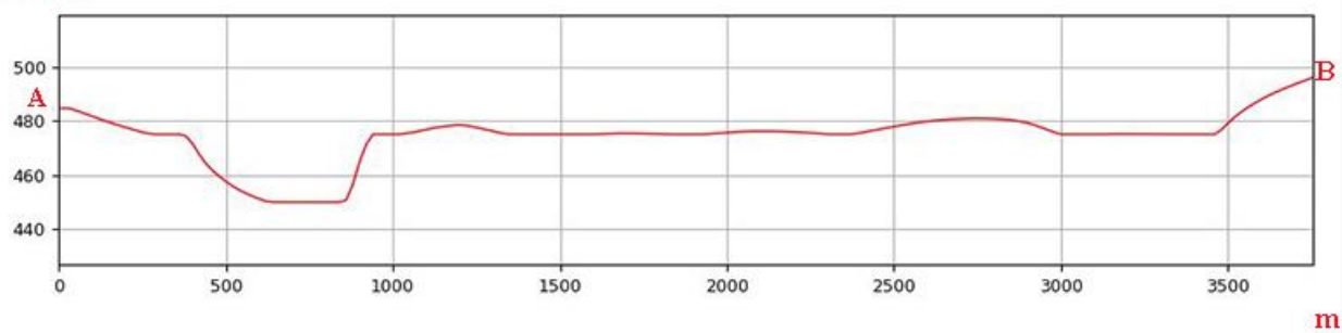
Sezione morfologica del terreno- Punto di presa n°13
