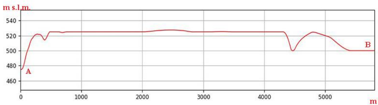
Sezione morfologica del terreno- Punto di presa n°4
