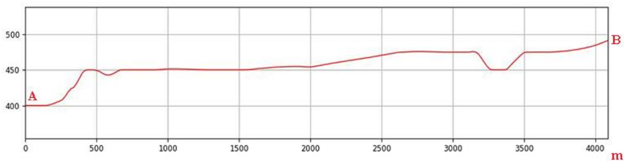
Sezione morfologica del terreno- Punto di presa n°8
