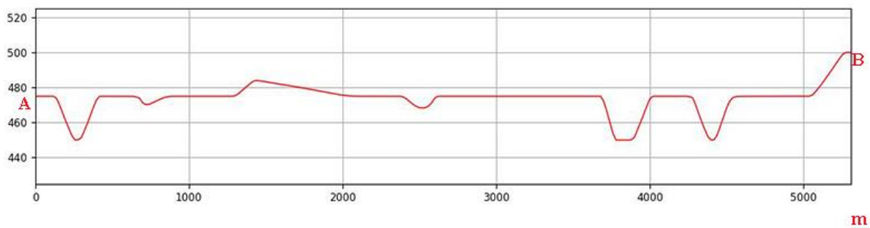
Sezione morfologica del terreno- Punto di presa n°12
