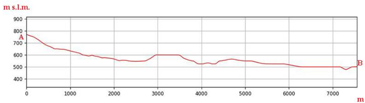
Sezione morfologica del terreno- Punto di presa n°16
