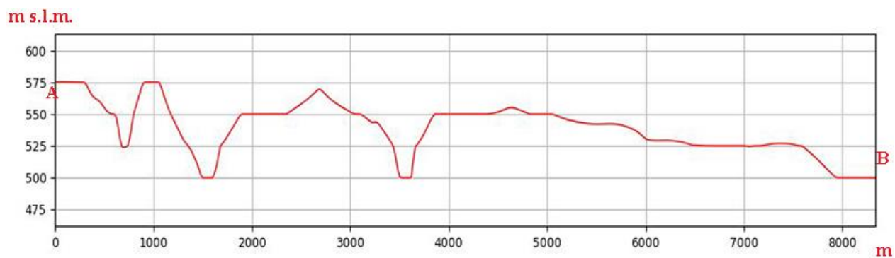
Sezione morfologica del terreno- Punto di presa n°6
