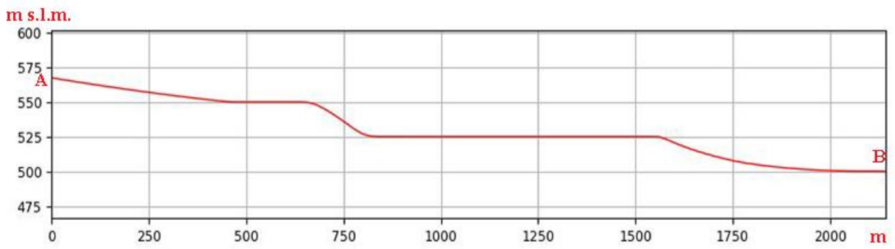
Sezione morfologica del terreno- Punto di presa n°2
