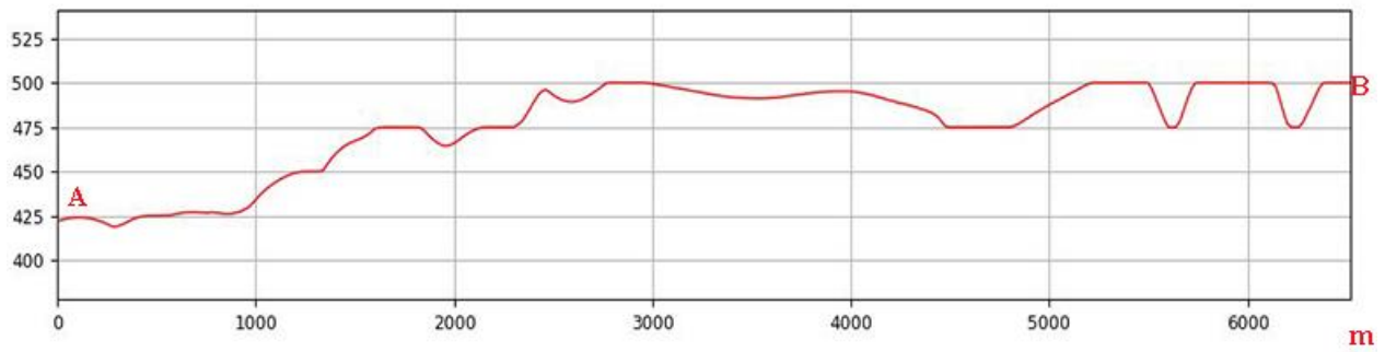
Sezione morfologica del terreno- Punto di presa n°11
