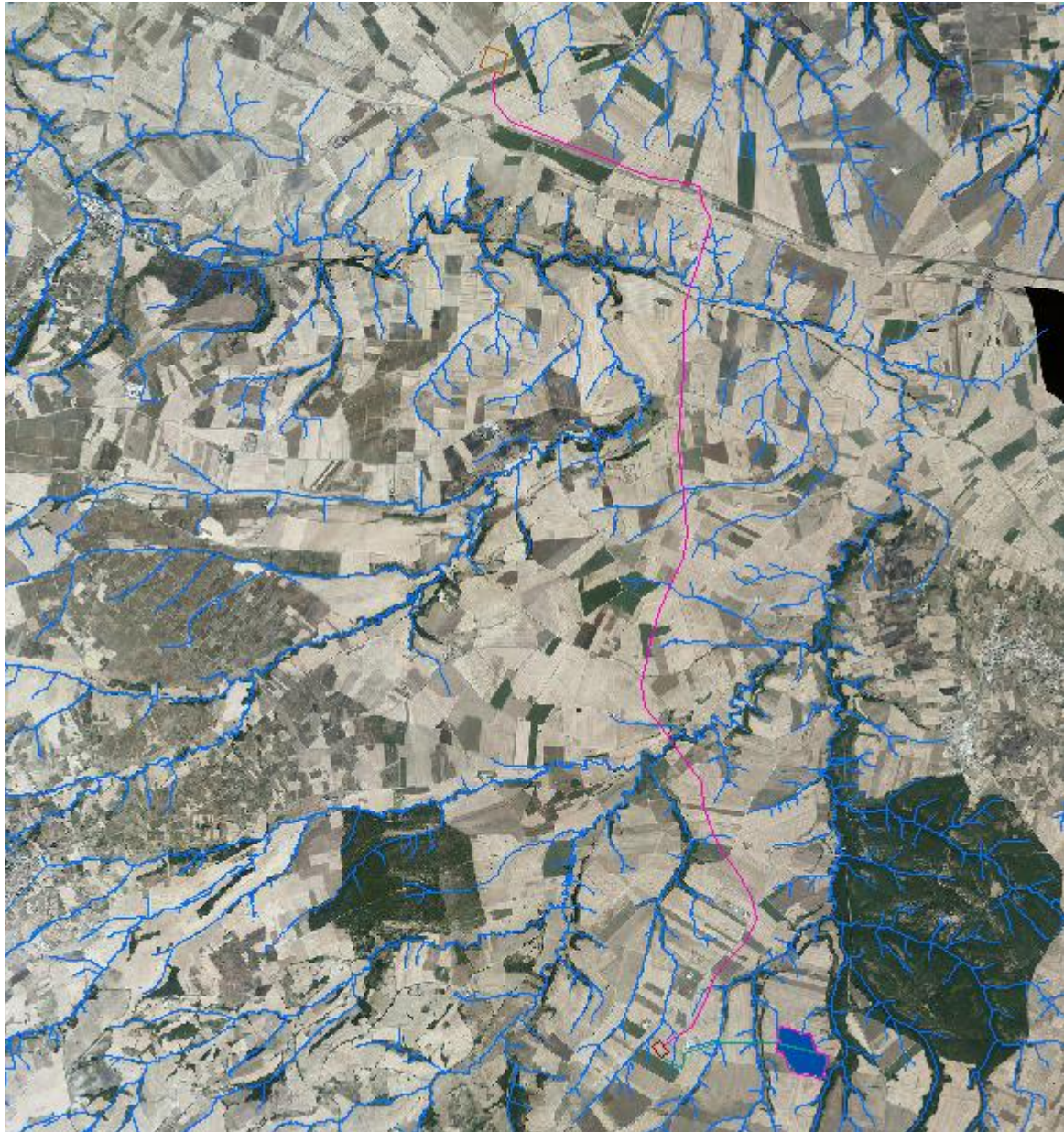
Figura 8.13. – Idrografia dell'area
