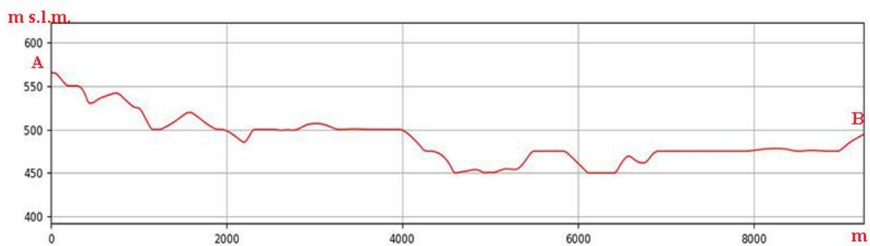
Sezione morfologica del terreno- Punto di presa n°15
