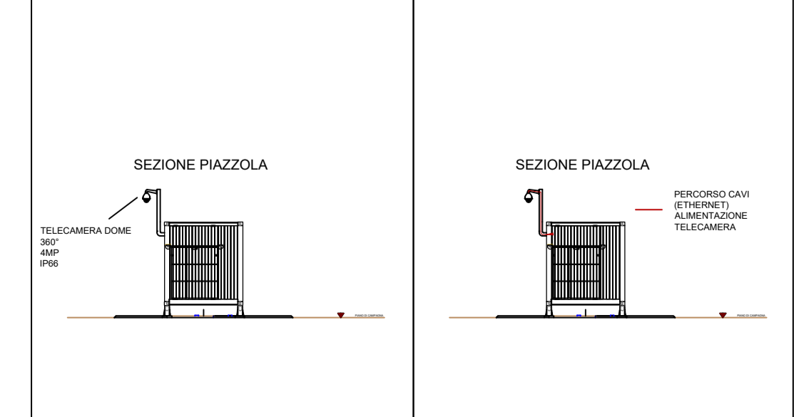
Particolare telecamera dome cabine di campo
