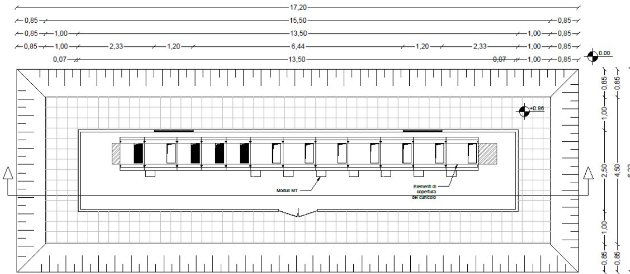
Cabina di raccolta lotto B
