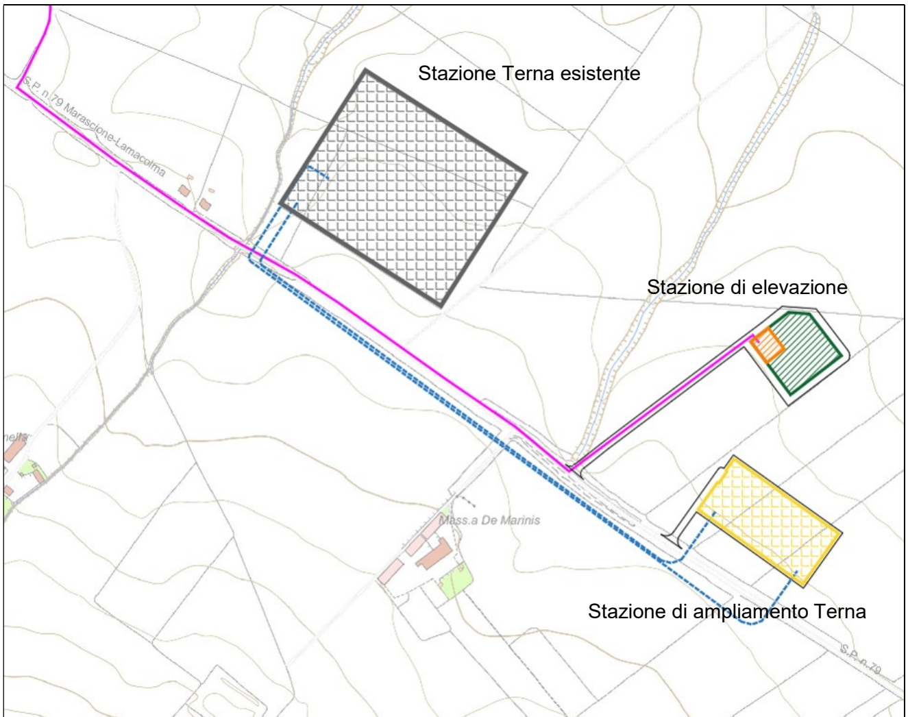
Stazione di elevazione MT/AT
