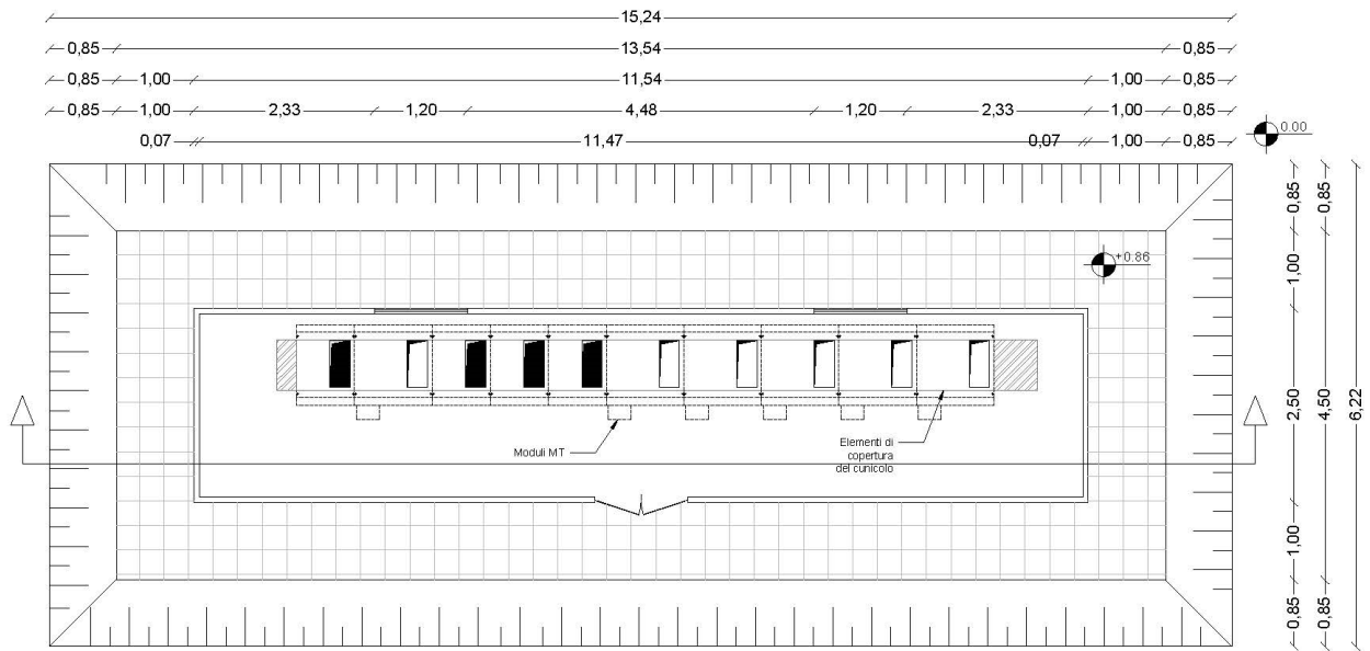
Cabina di raccolta LOTTO A
