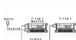
Estensione ingressi: unità MASTER/SLAVE via cavo
