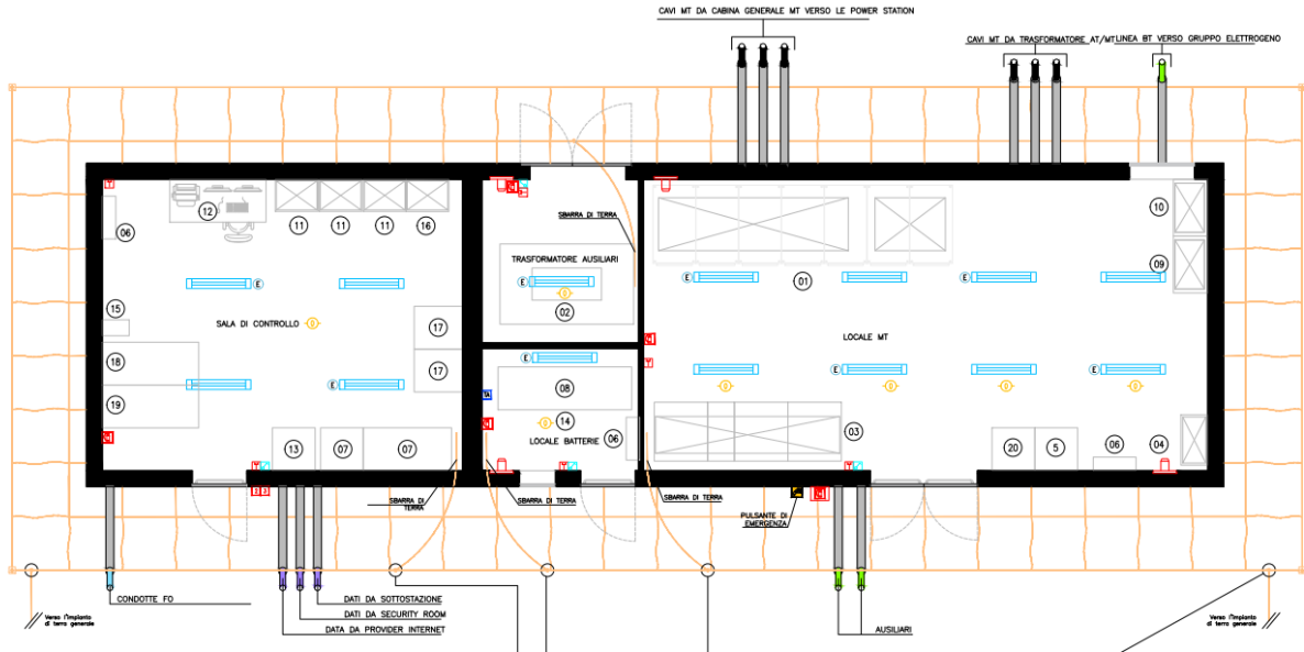
Figura 4.4 - Posizionamento plafoniere nella cabina MT.
