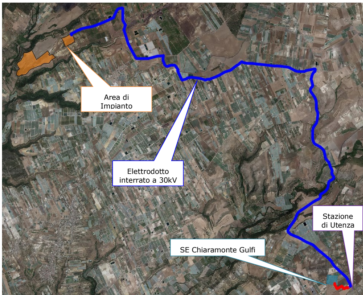
Figura 1: Tracciato degli elettrodotti MT e AT
