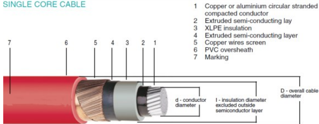
Figura 2: Caratteristiche cavi MT
