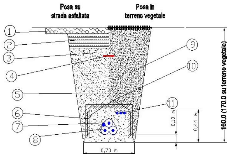
Figura 4: Tipici di posa cavi MT con n°2 linee su viabilità asfaltata
