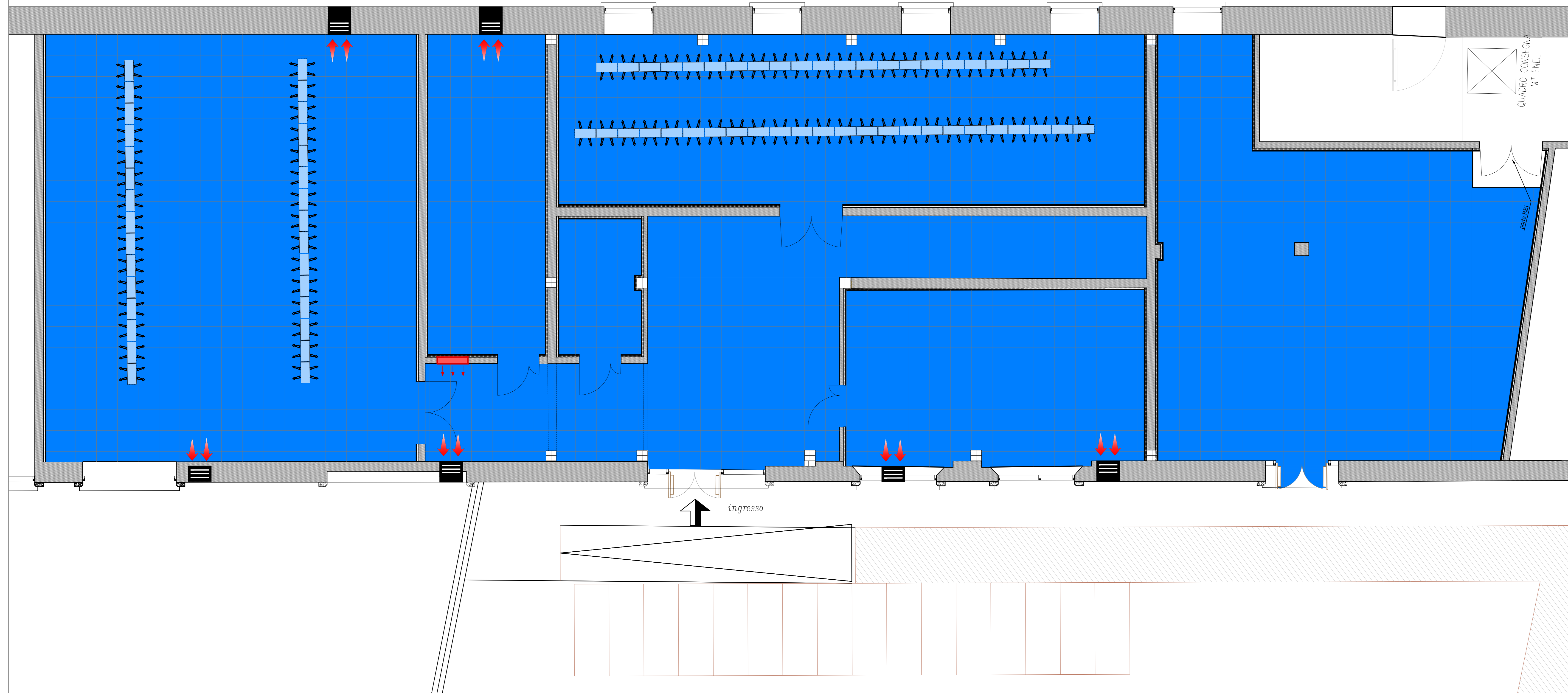
PLANIMETRIA PAVIMENTAZIONE FLOTTANTE Scala 1:50 N.B. Vedi tavola di dettaglio
