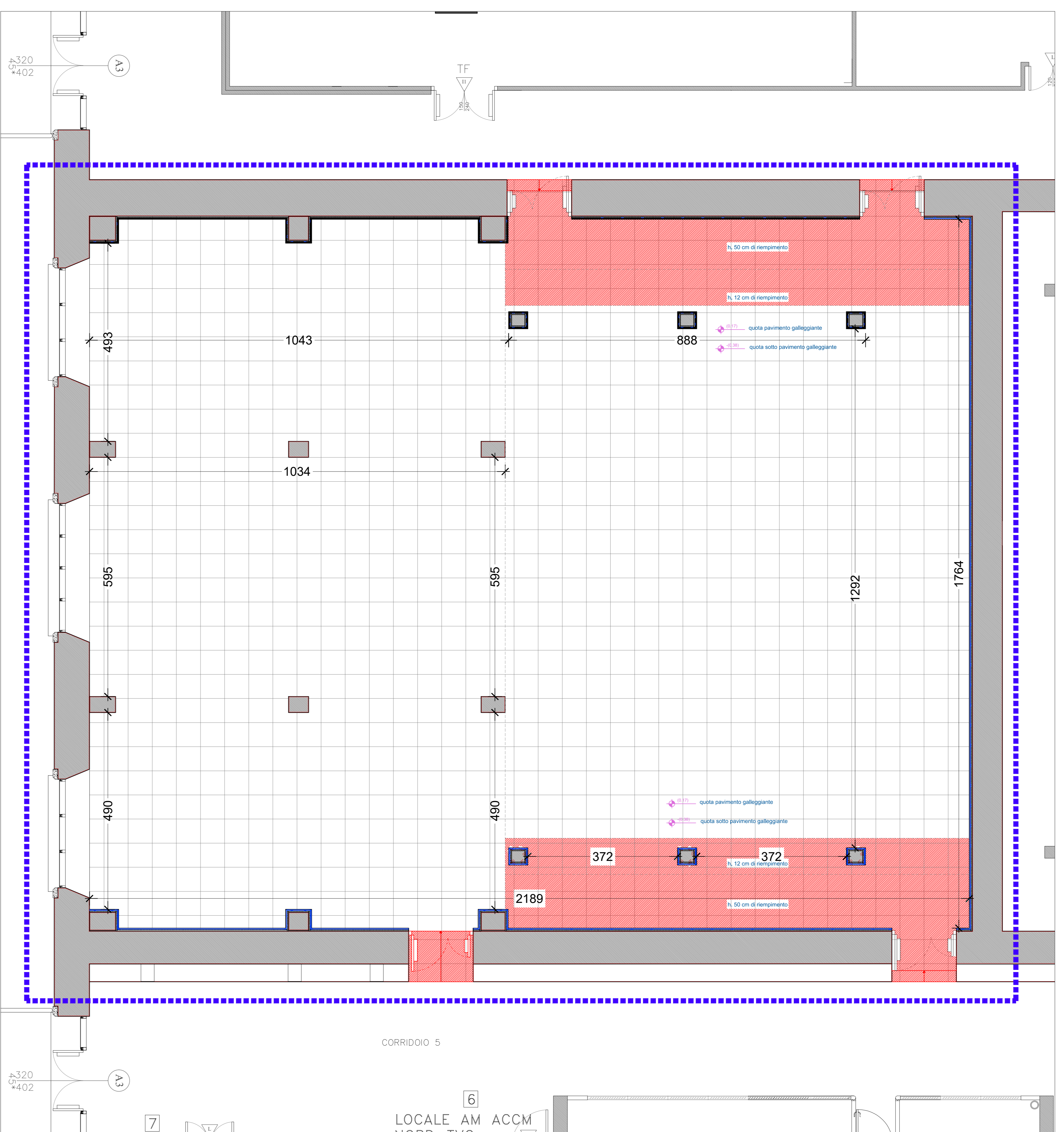
PLANIMETRIA - NUOVA SALA SERVER TVG Scala 1:50 - - - - - area oggetto di intervento - - - - - nuove costruzioni
