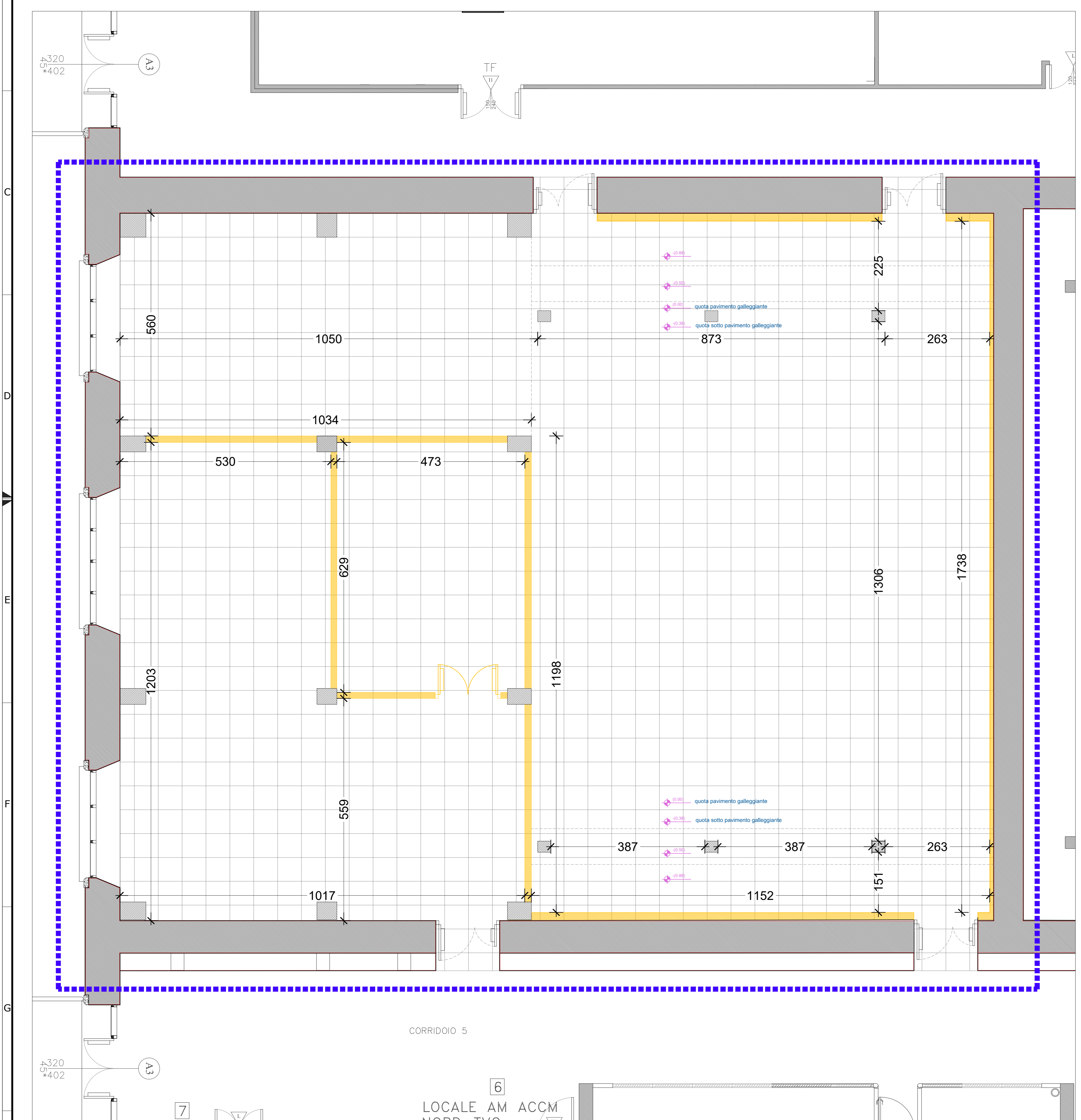
PLANIMETRIA - NUOVA SALA SERVER TVG Scala 1:50 - - - - - area oggetto di intervento - - - - - demolizioni
