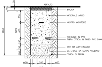
TRINCEA SU STRADA ASFALTATA TIPO "2C" - 2 CIRCUITI
