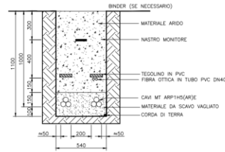
TRINCEA SU STRADA STERRATA TIPO "2C" - 2 CIRCUITI
