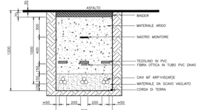
TRINCEA SU STRADA ASFALTATA TIPO "3C" - 3 CIRCUITI
