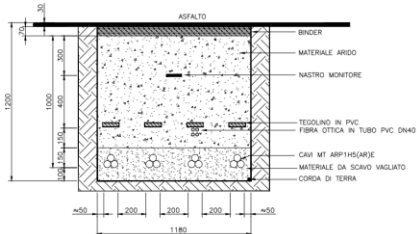
TRINCEA SU STRADA ASFALTATA TIPO "4C" - 4 CIRCUITI
