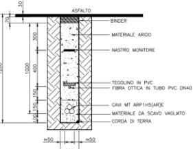
TRINCEA SU STRADA ASFALTATA TIPO "1C" - 1 CIRCUITO
