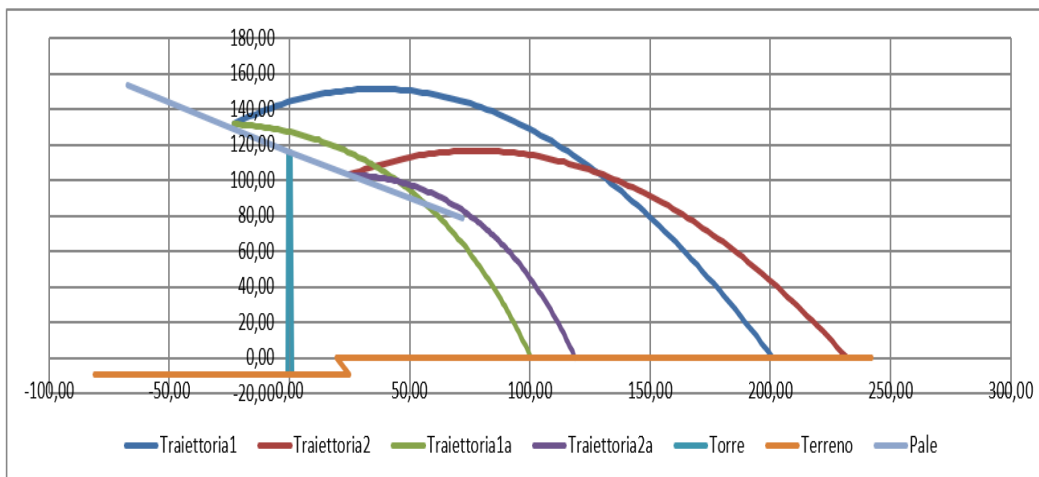
Figura 10 Calcolo della gittata mediante interpolazione dei diversi valori assunti dall'angolo di lancio \alpha in REAL CASE considerando un dislivello in posizione sottomessa del ricevitore rispetto all'aerogeneratore e la presenza di attrito viscoso dovuto all'aria
