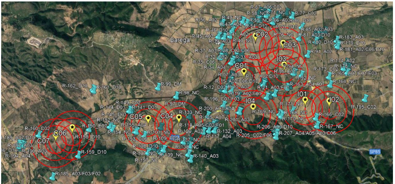
Figura 7 Disposizione dei ricettori (tabella 2) rispetto le Turbine con relativi buffer di 300, 500 e 700 metri
