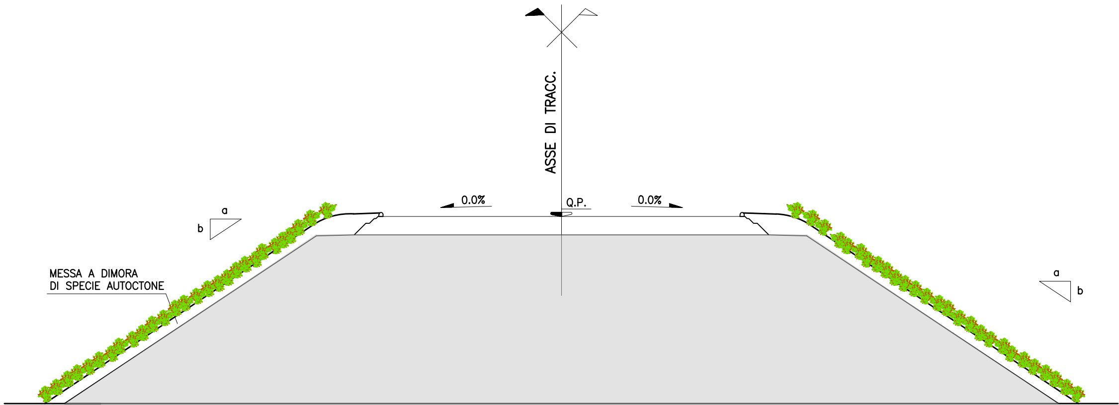
SISTEMAZIONE A VERDE SEZIONE TIPO IN RILEVATO
