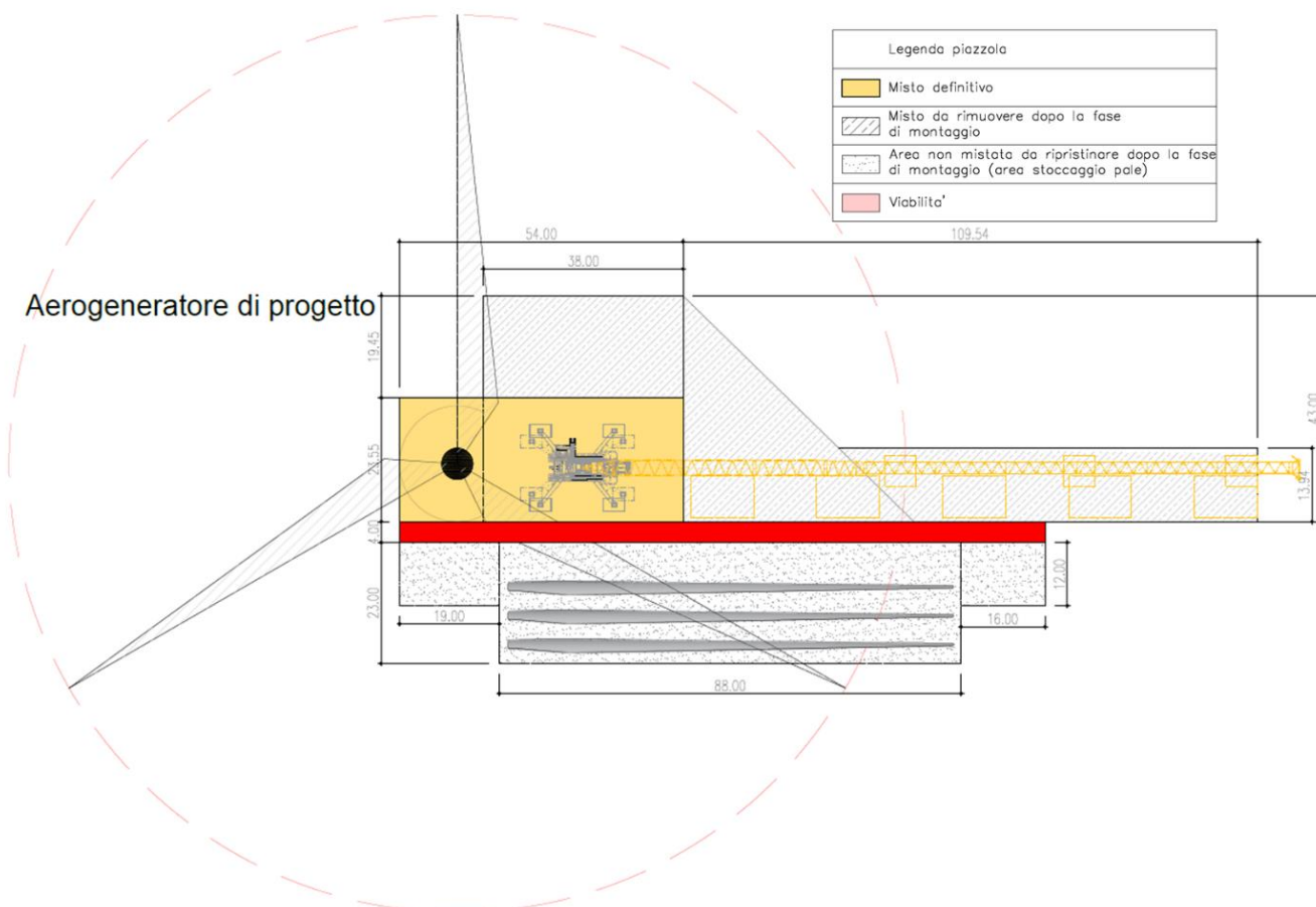
Figura 2: Configurazione piazzole degli aerogeneratori di progetto
