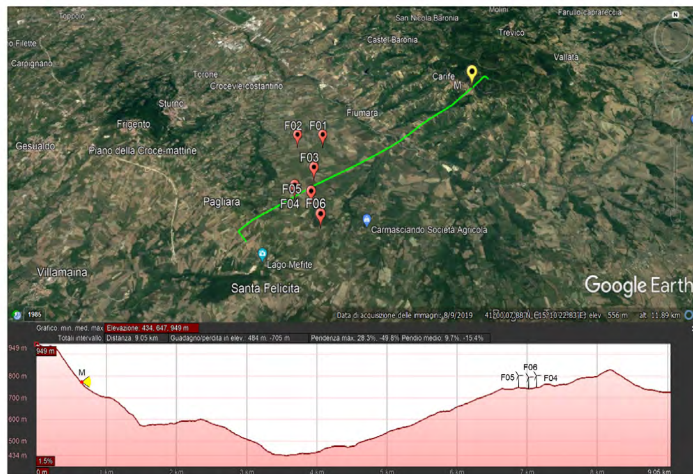
Sezione illustrativa della morfologia del terreno
