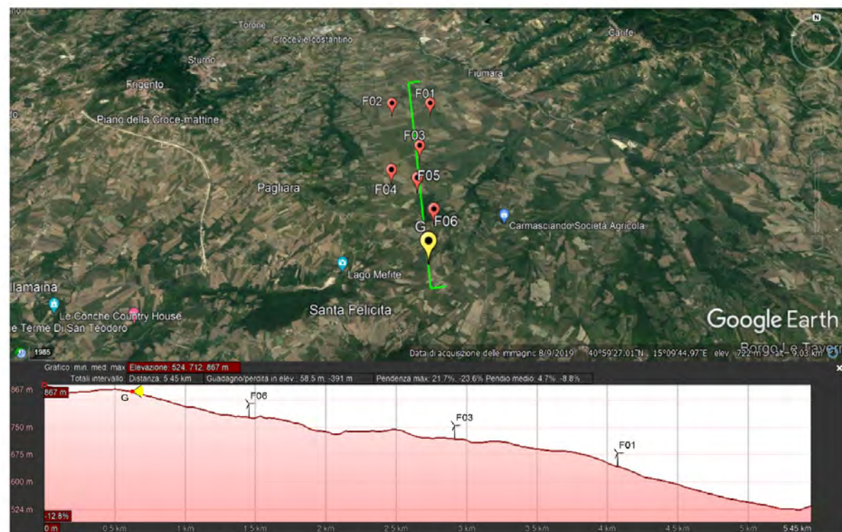
Sezione illustrativa della morfologia del terreno
