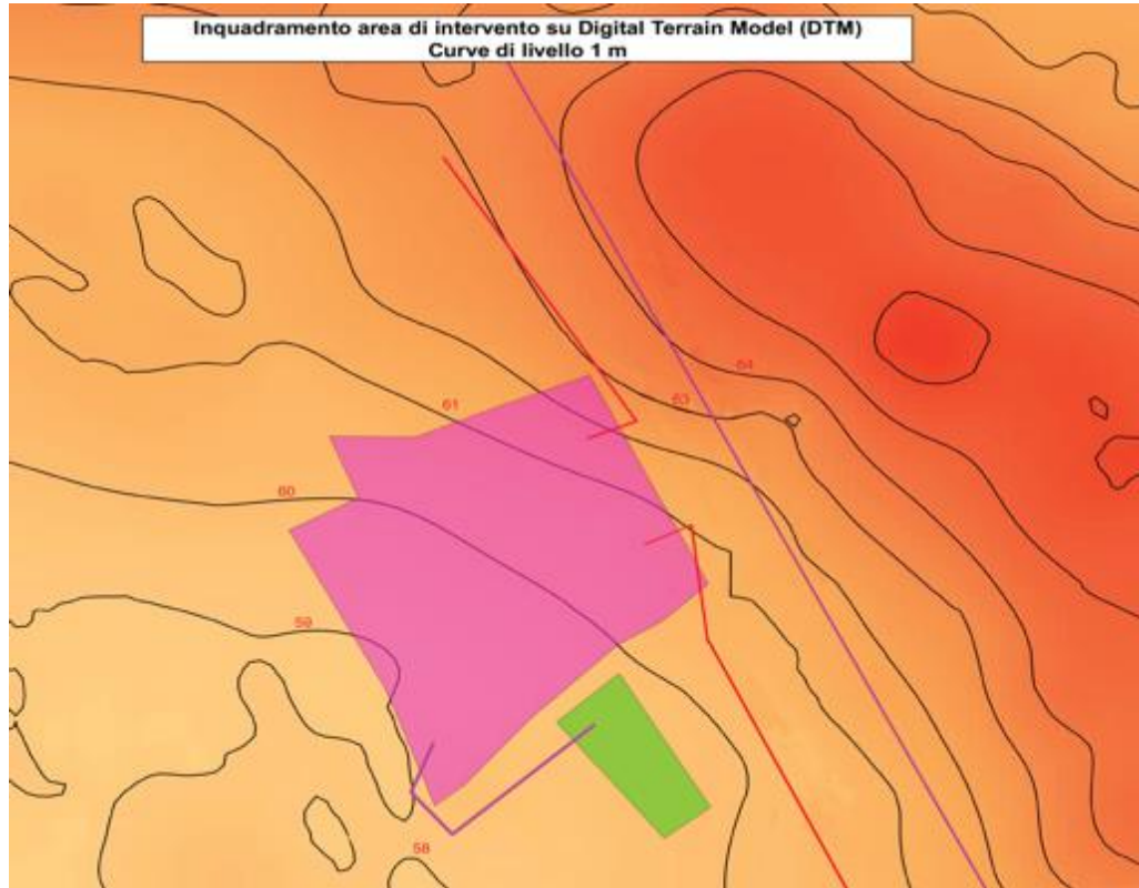
Tavola n. 11: Inquadramento con "digital terrain model" (DTM)
