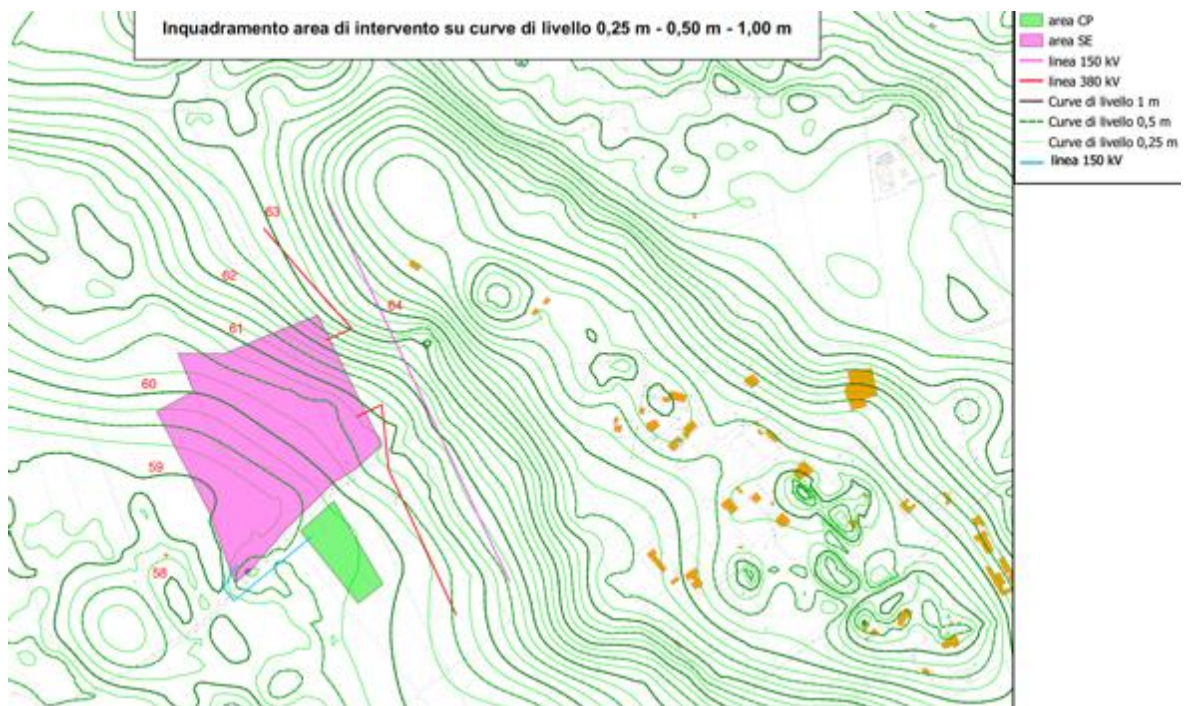
Tavola n. 10: Rilievo topografico con isoipse dell'ordine di 0,25 m., 0,50 m. e 1 m.
