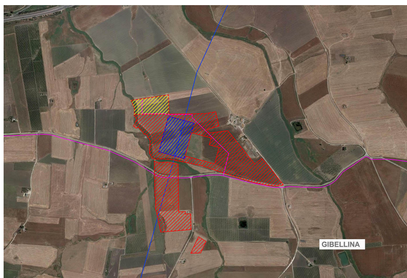
Figura 2 – Ubicazione area impianto e stazione di consegna (Google Earth)
