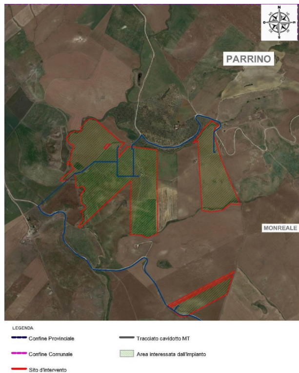
Figura 3 E - Ortofoto dell'area di impianto ricadente in Contrada Parrino (Monreale-PA) e cavidotto di connessione
