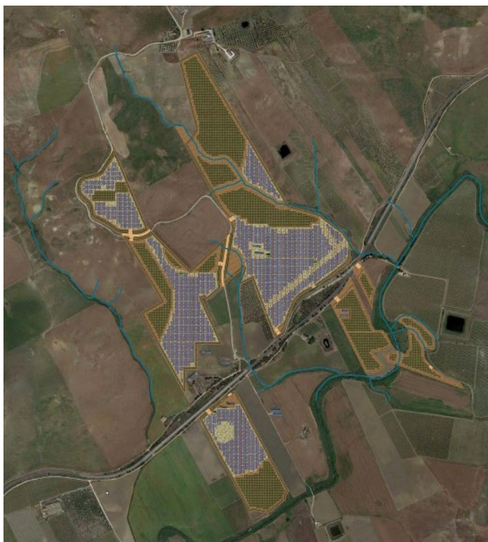
Figura 9 D – Ortofoto con render dell'area d'impianto con pannelli ricadente in Contrada Torretta
