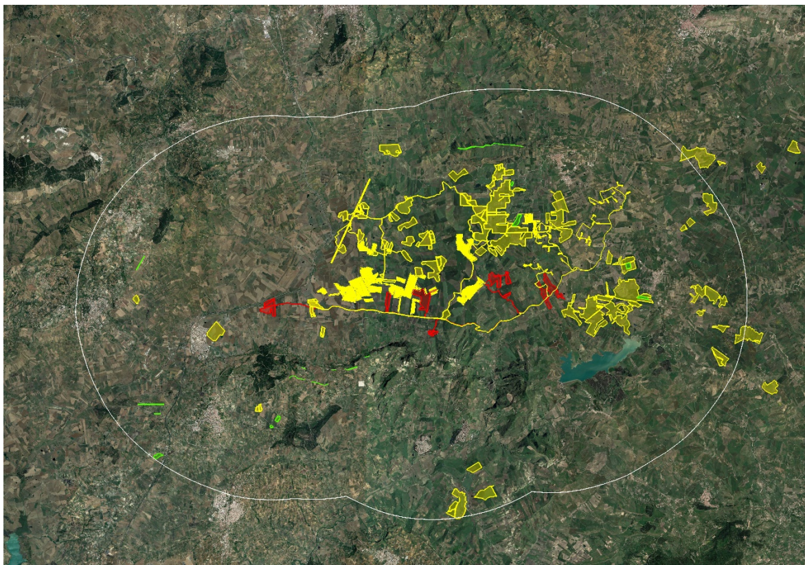
Fig 11 – Tutti gli impianti compresi nel buffer di 10 km dall'impianto S&P 9
