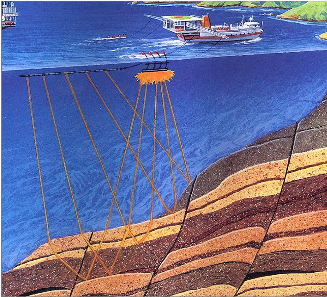
Figura 3.35 - Esempio di stendimento e linea di acquisizione sismica in mare (fonte: AAPG)
