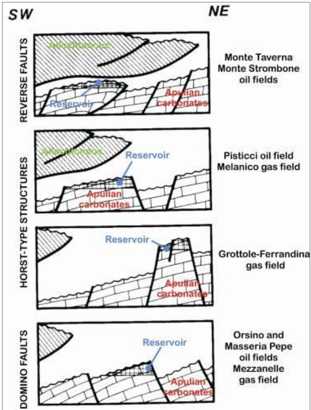
Figura 3.31 - Schemi delle varie tipologie di trappole (e relativi campi) impostatesi sul substrato carbonatico pre-pliocenico e trappole in substrato plio-pleistocenico (fonte: Sella et al., 1988, modificato)
