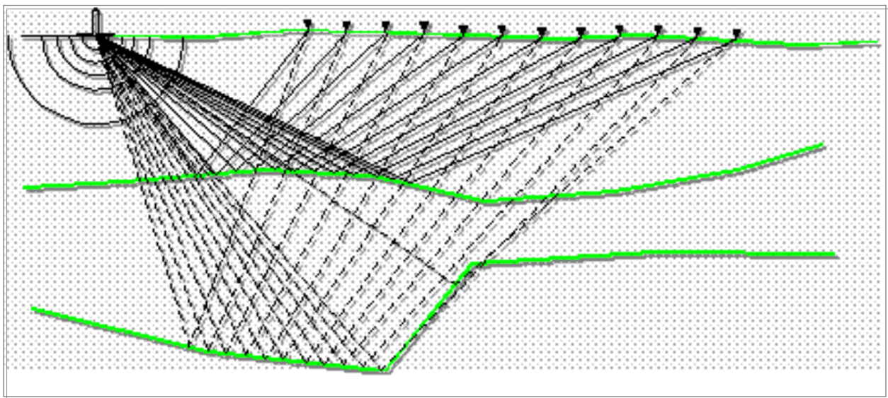
Figura 3.33 - Concetti di sismica a riflessione e percorso delle onde sismiche captate dai ricevitori (fonte: www.retegeofisica.it )
