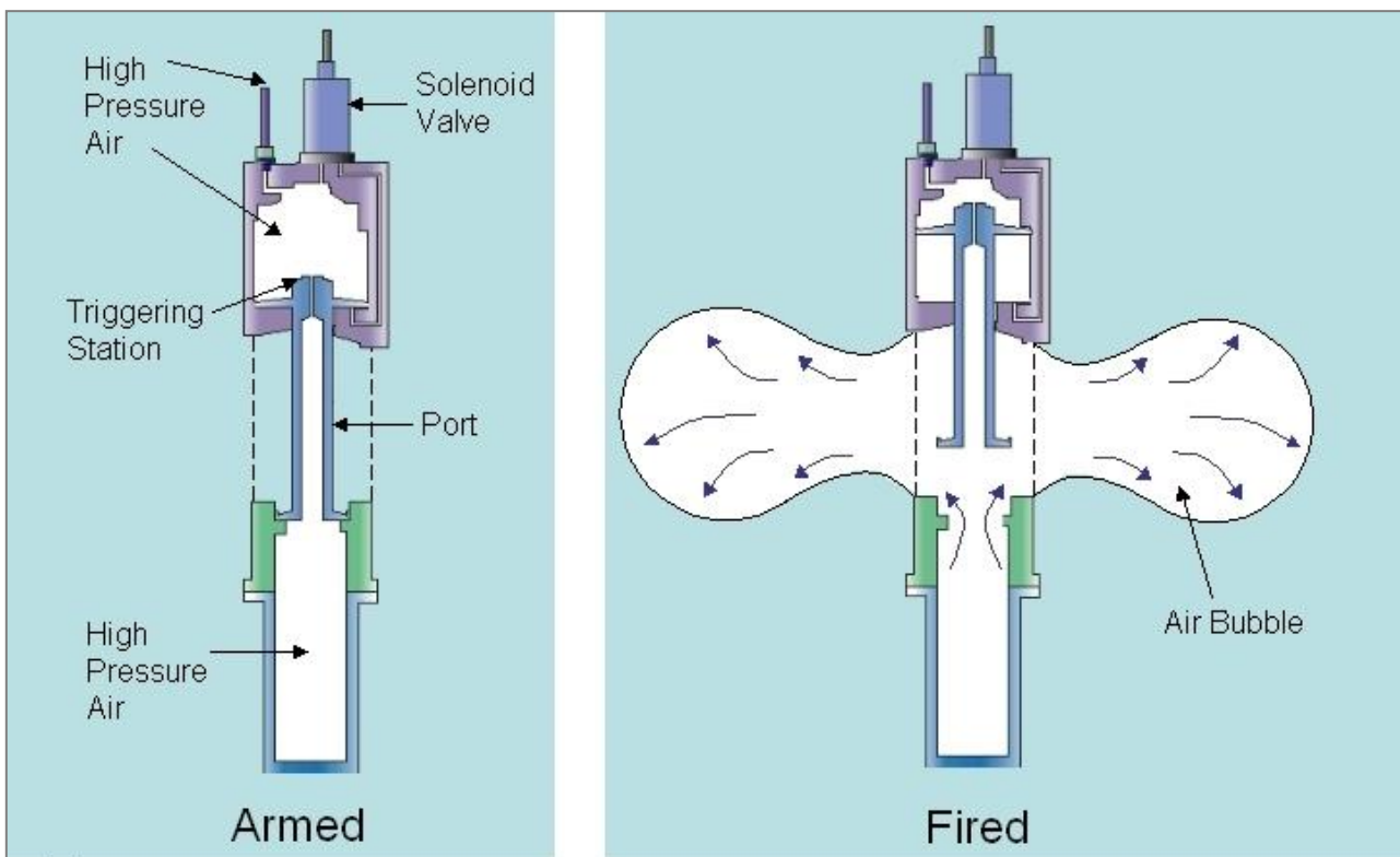
Figura 3.37 - Esempio di caricamento di un airgun e rilascio dell'aria compressa verso l'esterno (fonte: www.petroleumgeophysics.com )
