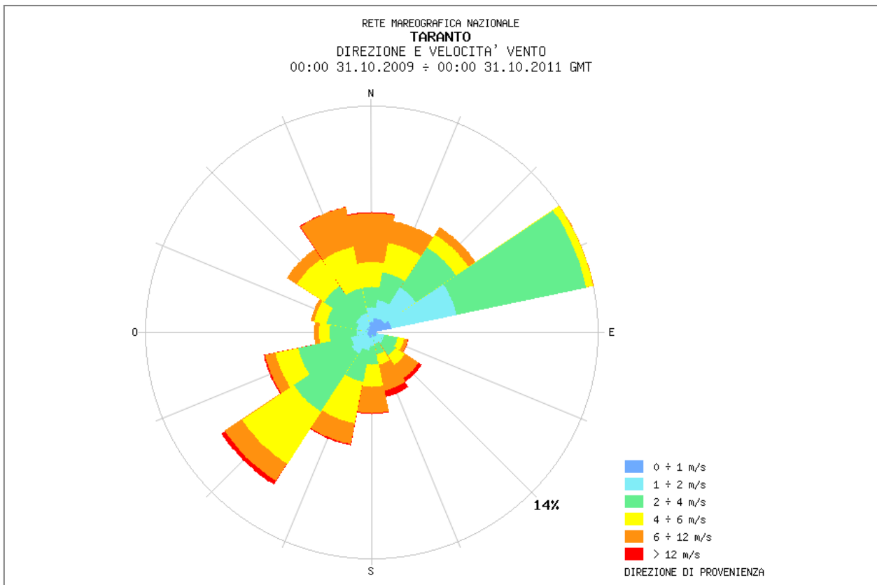
Figura 4.26 - Rosa dei venti illustrante il regime anemometrico medio nel periodo 31/10/2009-31/10/2011 a Taranto (fonte: www.mareografico.it)
