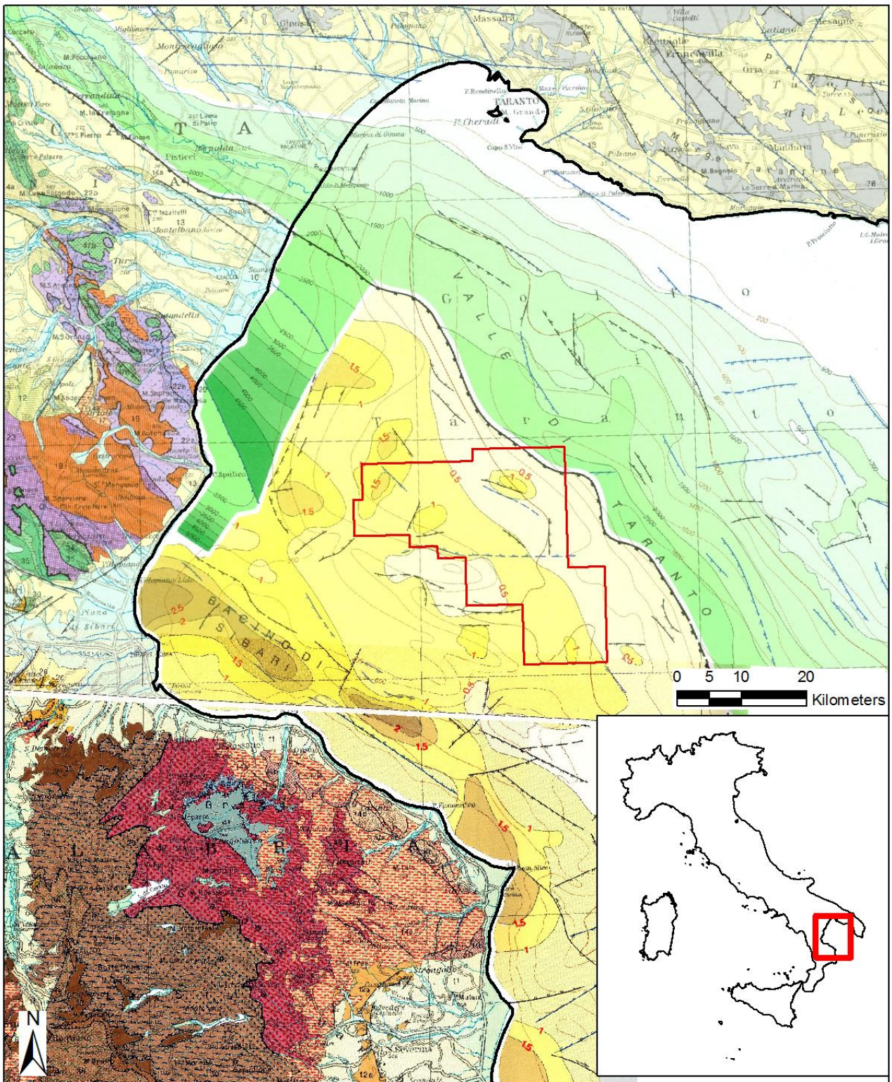
Figura 3.3 - Stralcio della carta geologica del settore della parte settentrionale del Mar Ionio (Golfo) e delle aree limitrofe
