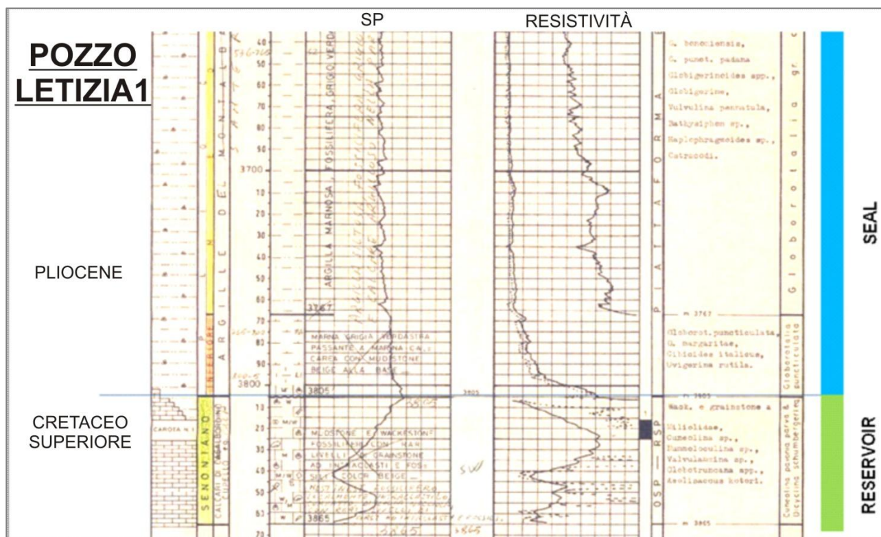
Figura 3.29 - Esempio di roccia di copertura Pliocenica sopra il Cretaceo nel pozzo Letizia 1
