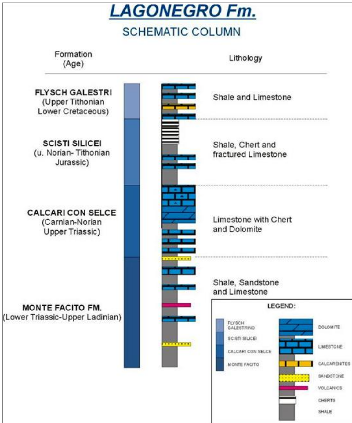
Figura 3.10 - Relazioni crono-stratigrafiche tra le varie formazioni costituenti la Formazione di Lagonegro
