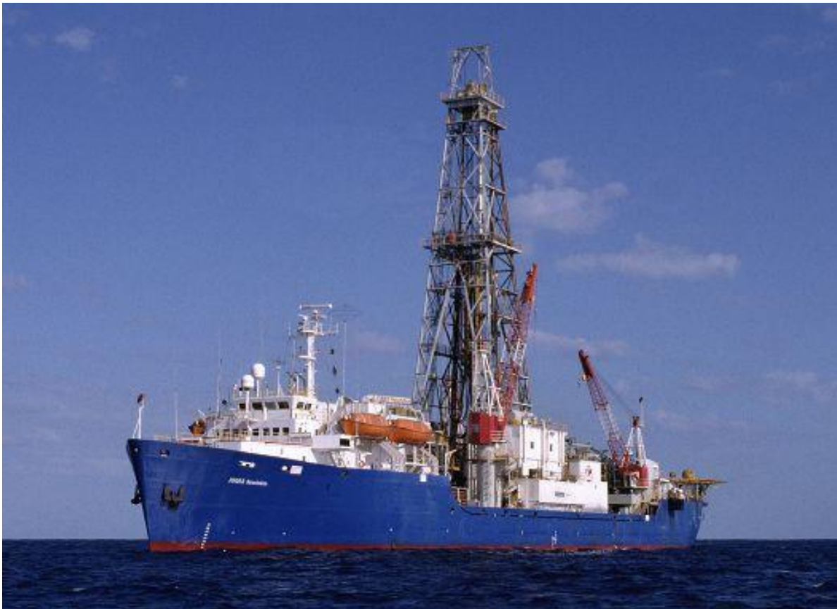
Figura 3.46 - Esempio di drilling ship (fonte: www-odp.tamu.edu )
