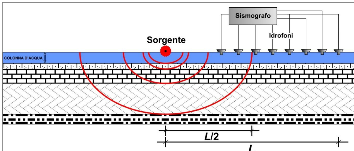
Figura 3.34 – Schema esemplificativo di uno stendimento sismico in mare energizzato da una fonte distante L dall'ultimo idrofono
