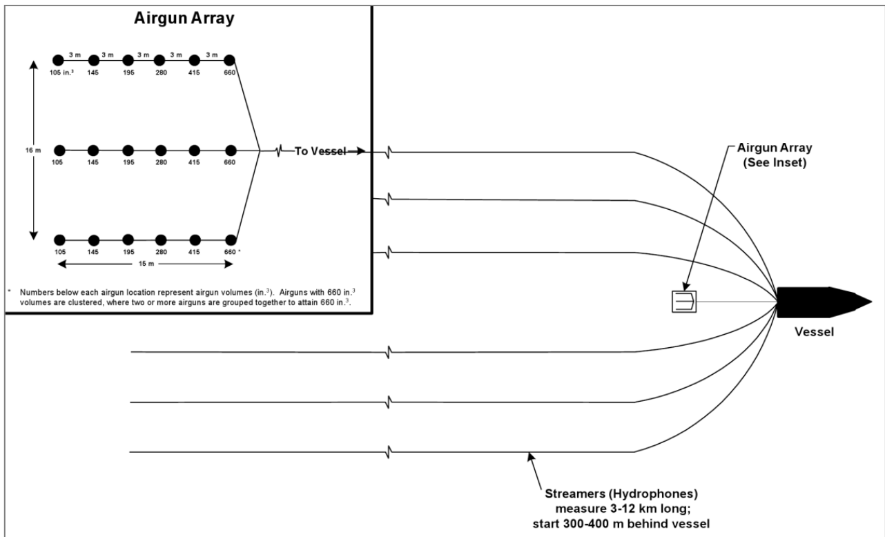
Figura 3.38 – Esempio di possibile configurazione di un array (fonte: OCS EIS/EA MMS 2004-054)
