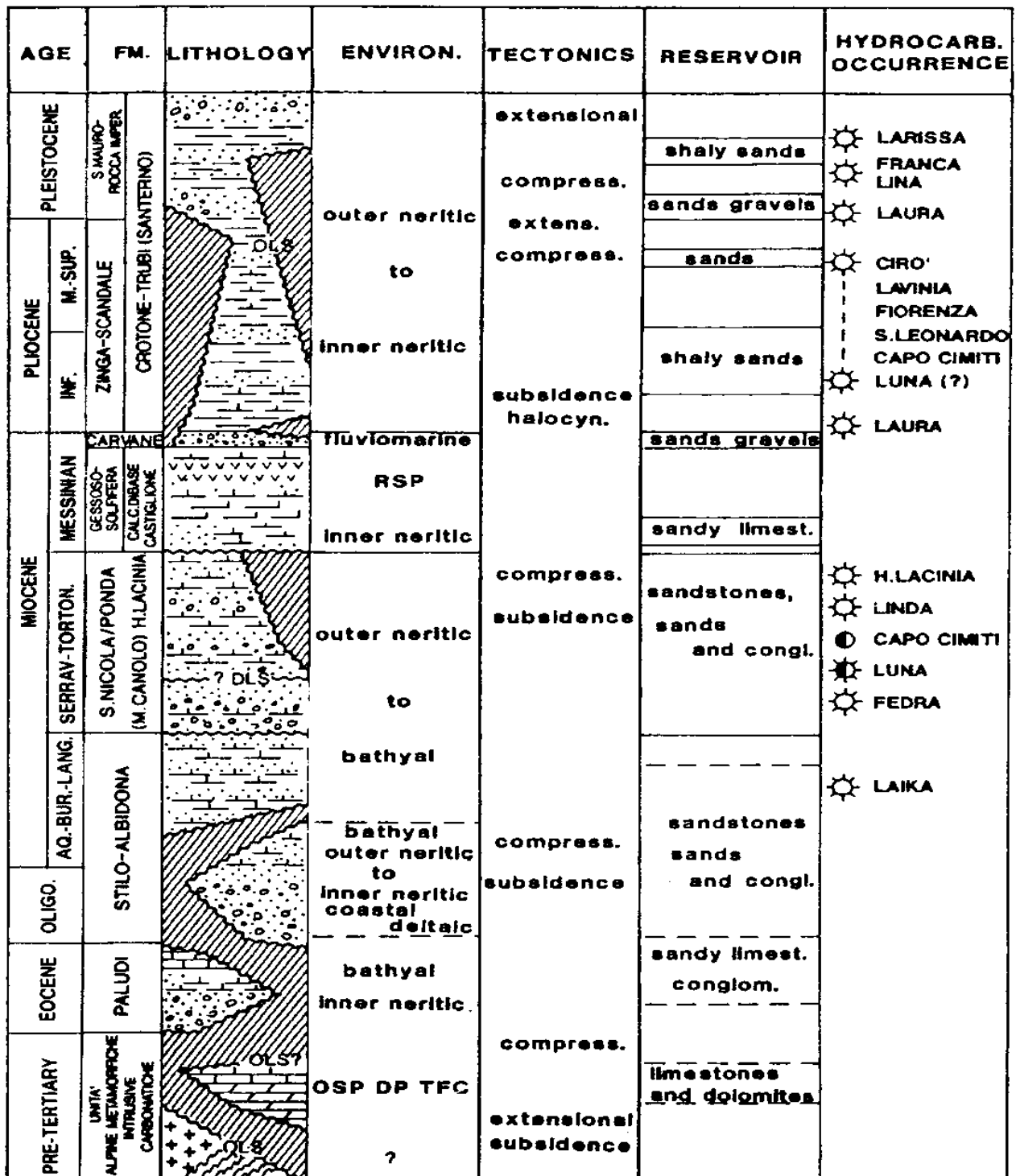
Figura 3.20 - Schema geologico della zona a mare dell'Arco Calabro con la distribuzione delle principali fasi tettoniche e delle rocce serbatoio
