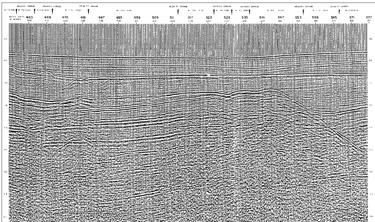
Figura 3.36 - Esempio di sezione sismica non interpretata risultante da coperture multiple
