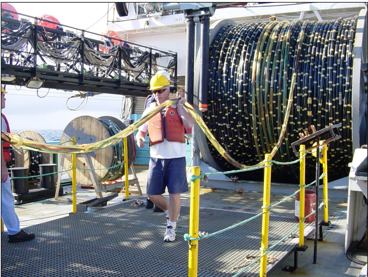
Figura 3.41 – Esempio di cavo per l'acquisizione sismica in mare (fonte: www.ig.utexas.edu )
