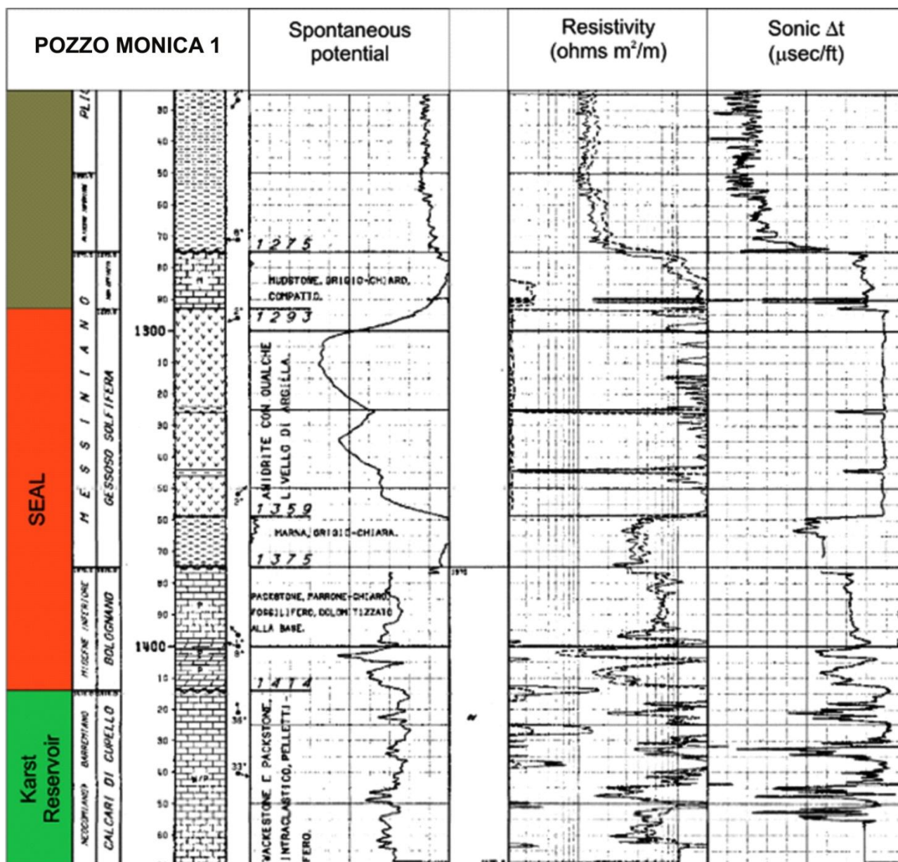
Figura 3.28 - Composite log dal pozzo Monica 1
