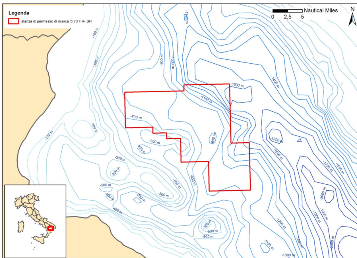
Figura 2.1 – Ubicazione con relativo perimetro dell'area in istanza di permesso di ricerca con indicazione della batimetria
