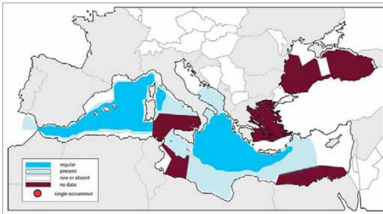
Figura 4.47 - Presenza di capodogli nel mar Mediterraneo (fonte: Notarbartolo di Sciara & Birkun, 2010)
