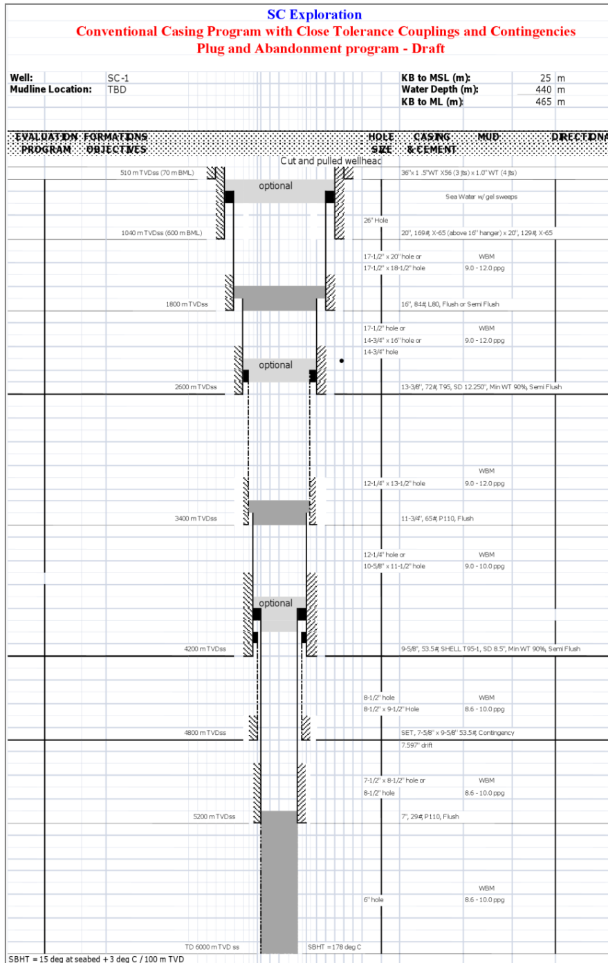
Figura 3.49 - Schema di eventuale abbandono del pozzo secondo le procedure standard di Shell Italia E&P S.p.A.
