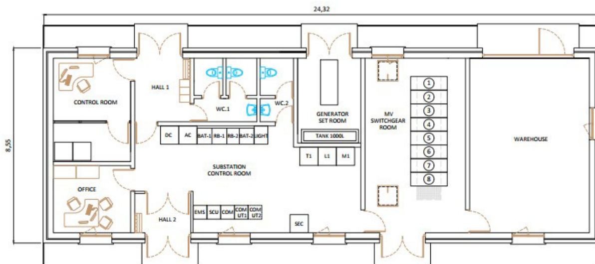
Layout edificio consegna
