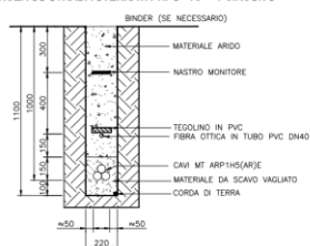
TRINCEA SU STRADA STERRATA TIPO "1C" - 1 CIRCUITO
