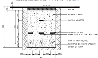
TRINCEA SU STRADA ASFALTATA TIPO "3C" - 3 CIRCUITI
