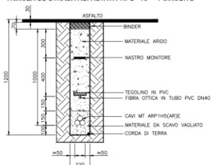
TRINCEA SU STRADA ASFALTATA TIPO "1C" - 1 CIRCUITO
