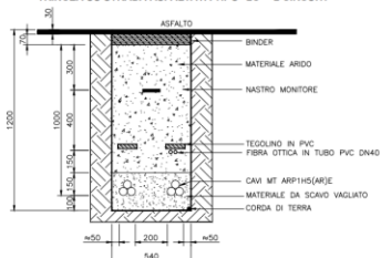
TRINCEA SU STRADA ASFALTATA TIPO "2C" - 2 CIRCUITI
