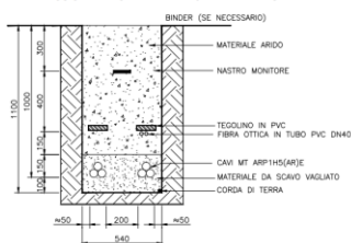
TRINCEA SU STRADA STERRATA TIPO "2C" - 2 CIRCUITI
