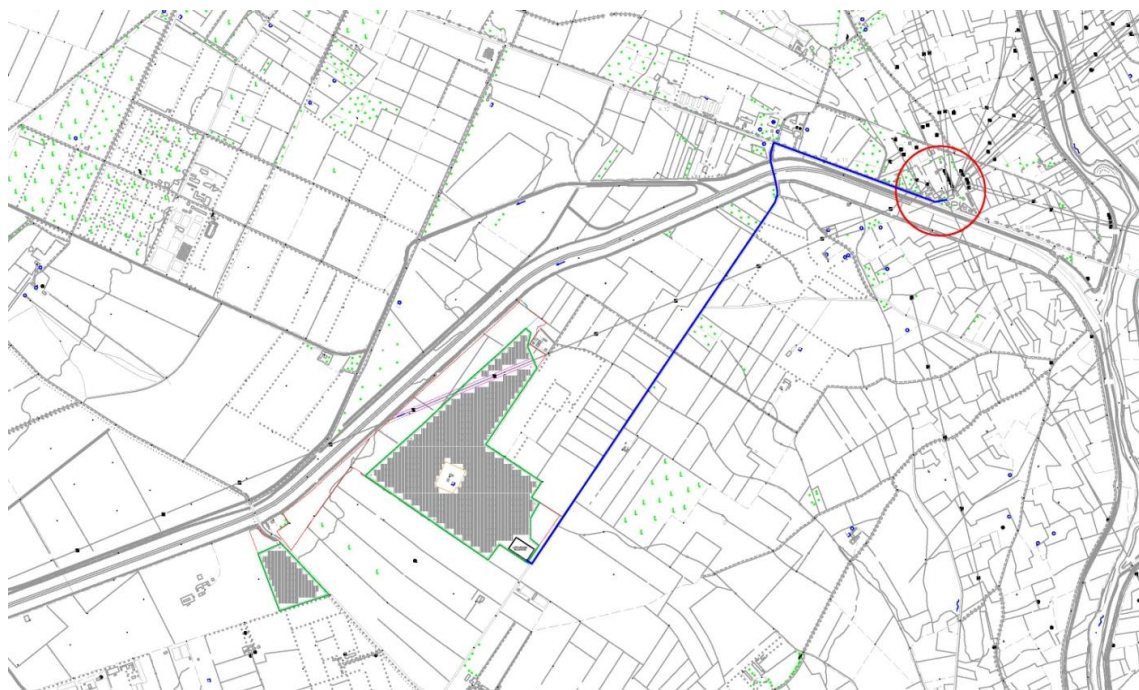
Figura 4: Stralcio mappa CTR Fogli 556030 e 556040 con indicazione del campo AGV e della linea di connessione.
