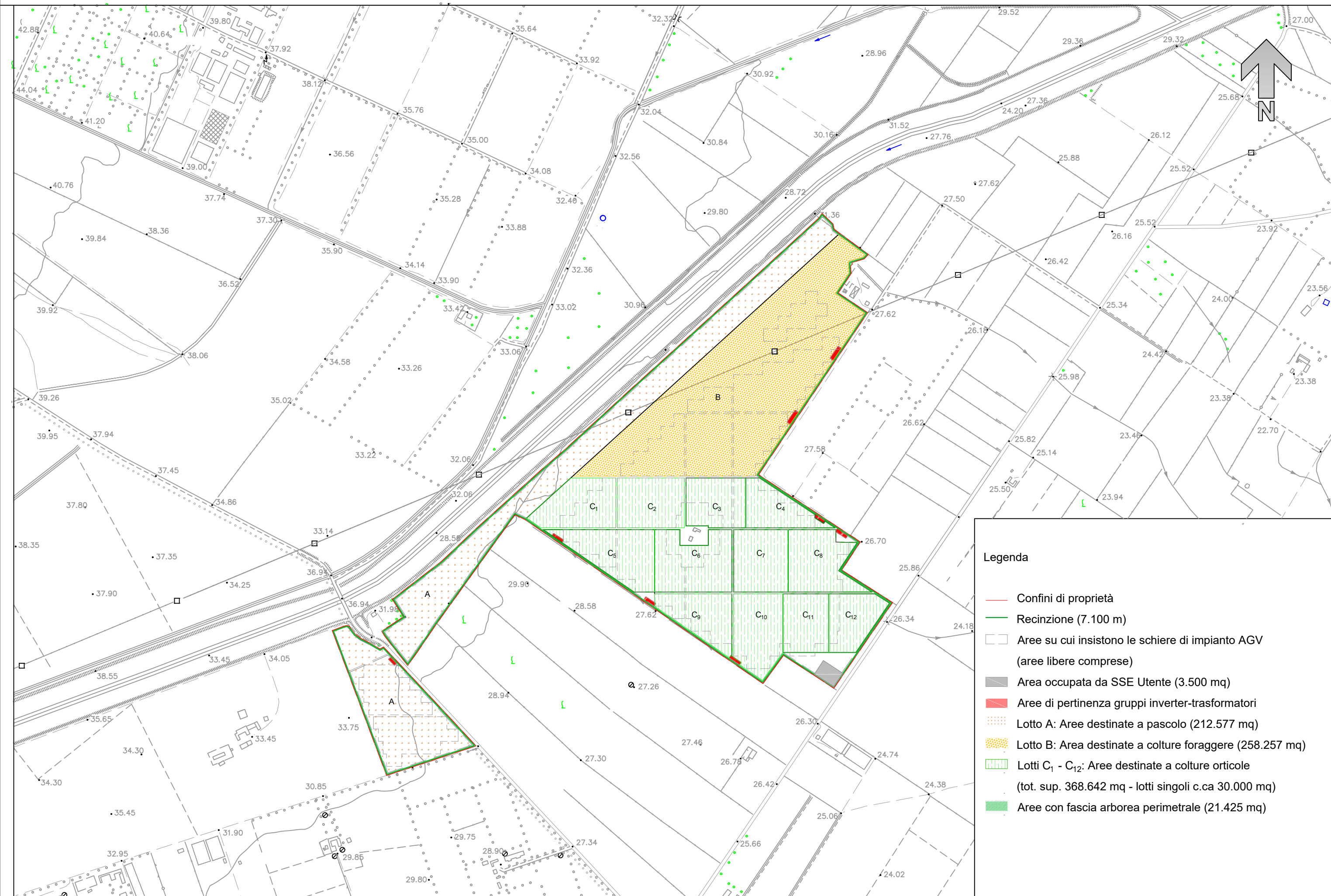
PLANIMETRIA AREA D'INTERVENTO CON INDICAZIONE DELLA DESTINAZIONE AGRICOLA DEI LOTTI
