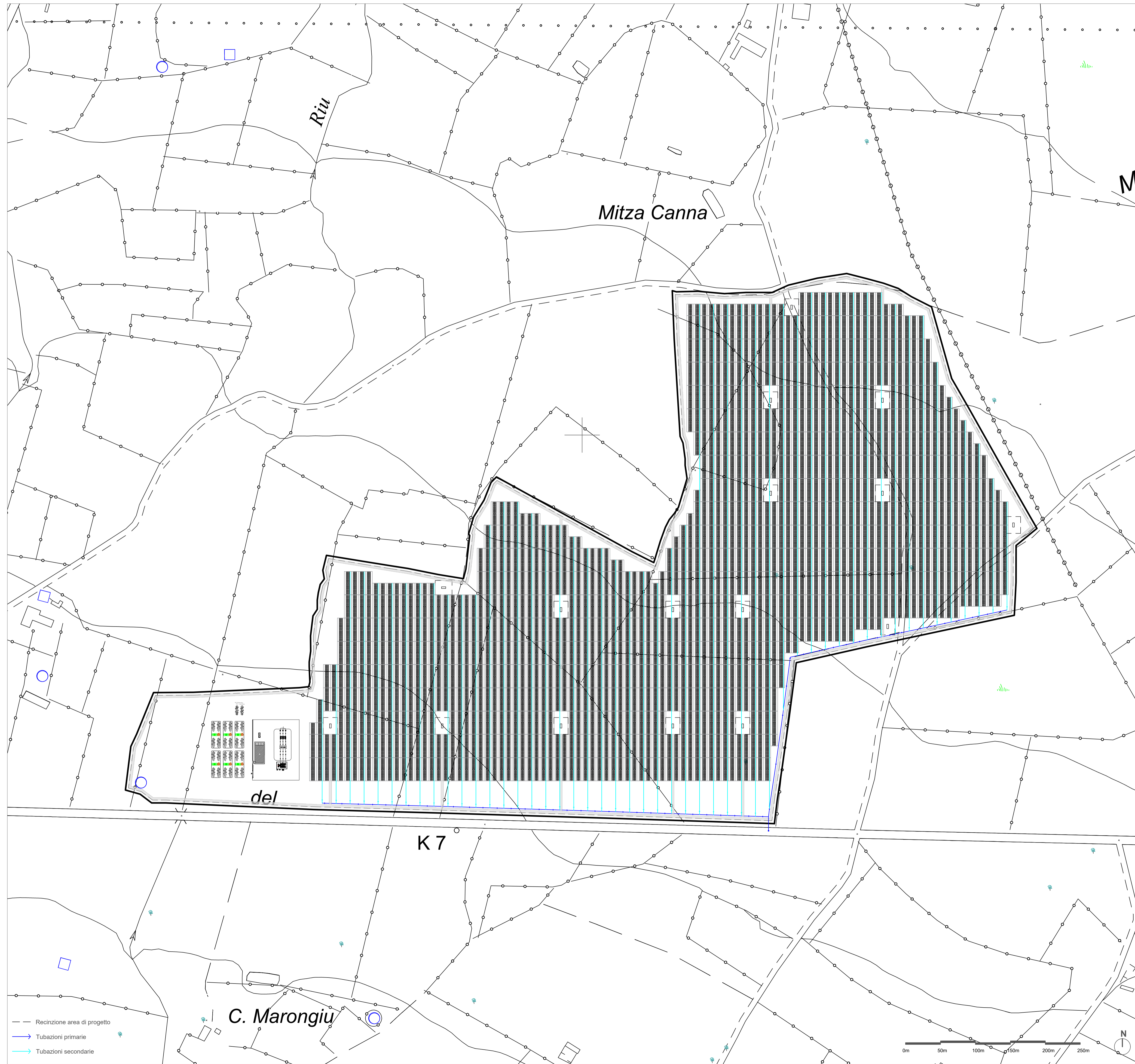
PLANIMETRIA - SMALTIMENTO ACQUE METEORICHE scala 1: 10 000
