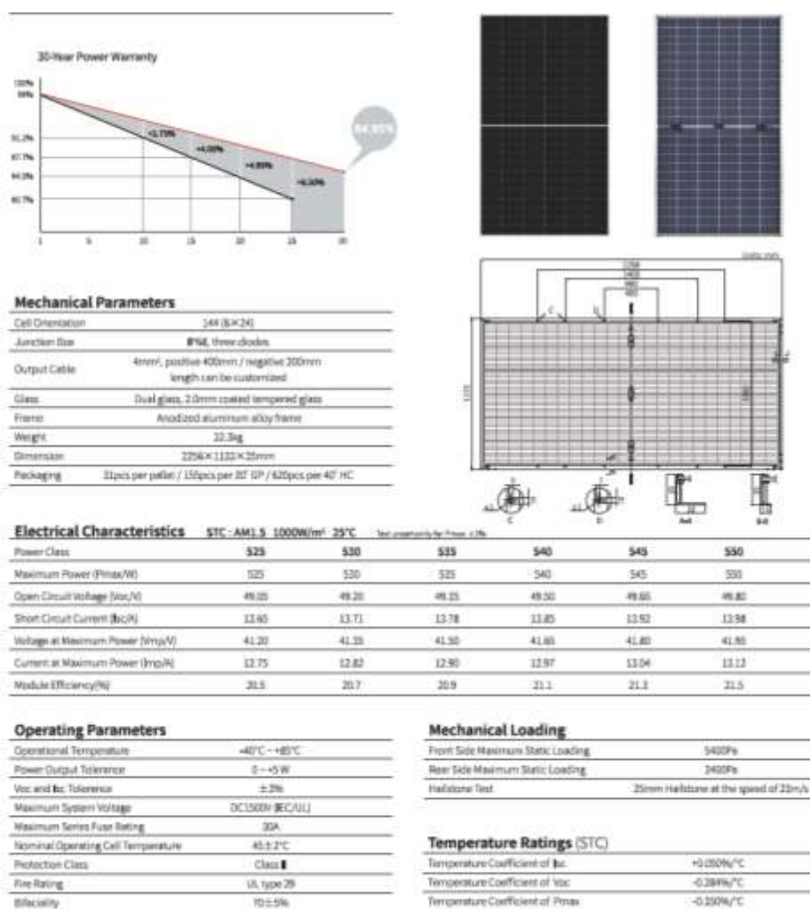
Fig. Pannello longi LR5-72HBD- DA 545W
