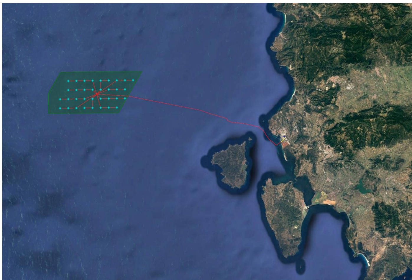
Figura 2 – Localizzazione del parco eolico, con posa in mare e a terra, da stazione offshore a stazione onshore del Sulcis (SU)
