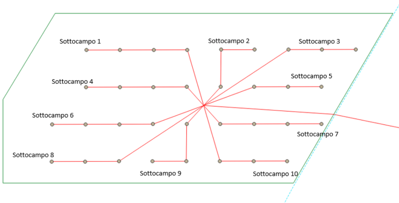
Figura 4 - Struttura del parco eolico con indicazione dei sottocampi e della stazione Off-Shore
