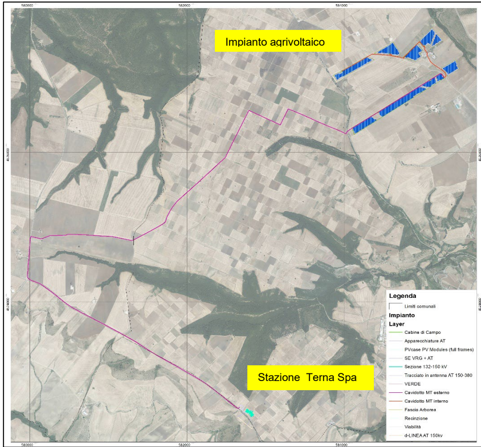
Figura 2: localizzazione dell'area d'impianto e della stazione SE-Terna "Palazzo San Gervasio"
