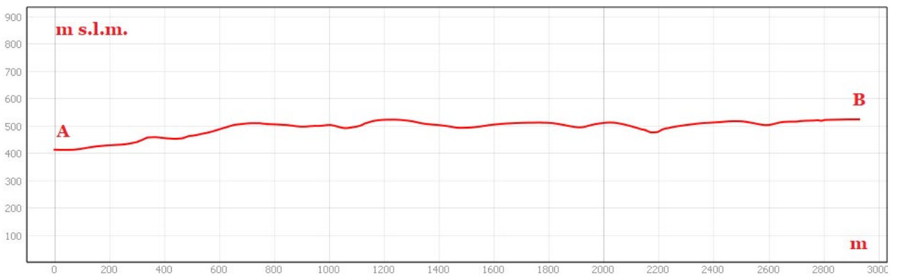
Sezione morfologica del terreno- Punto di presa n°5
