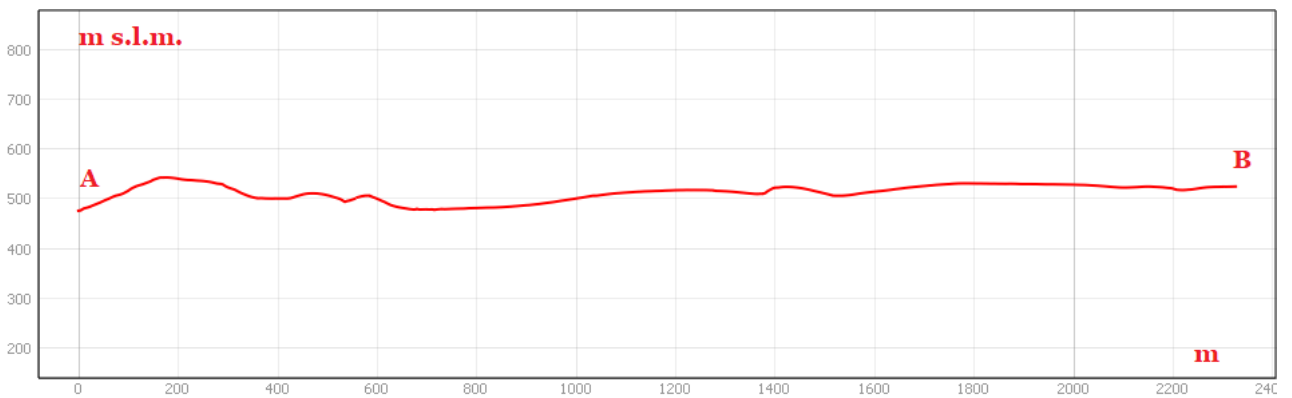
Sezione morfologica del terreno- Punto di presa n°6
