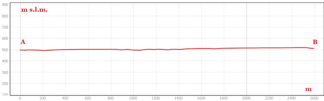
Sezione morfologica del terreno- Punto di presa n°12
