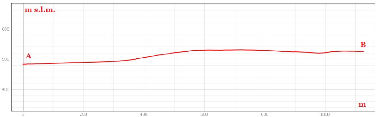
Sezione morfologica del terreno- Punto di presa n°18
