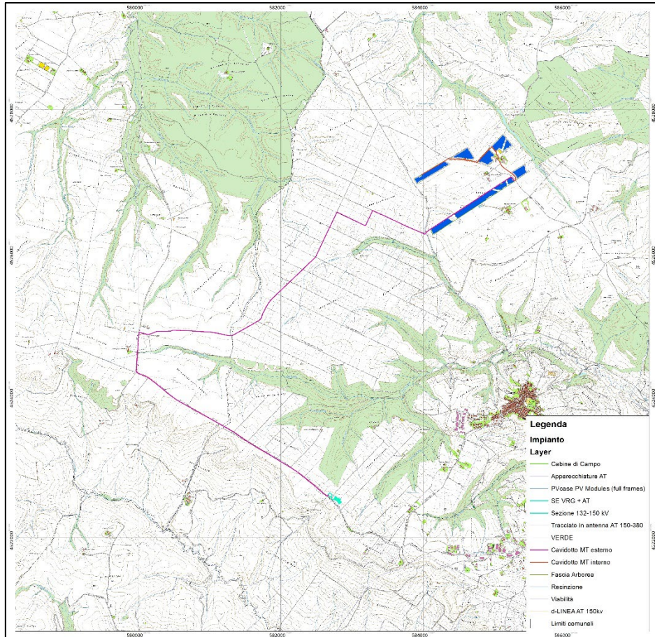
Figura 6 - Progetto dell'impianto FV su CTR
