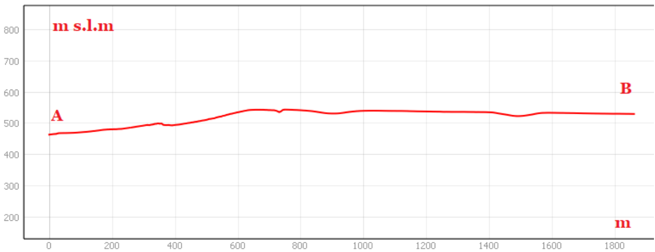
Sezione morfologica del terreno- Punto di presa n°4
