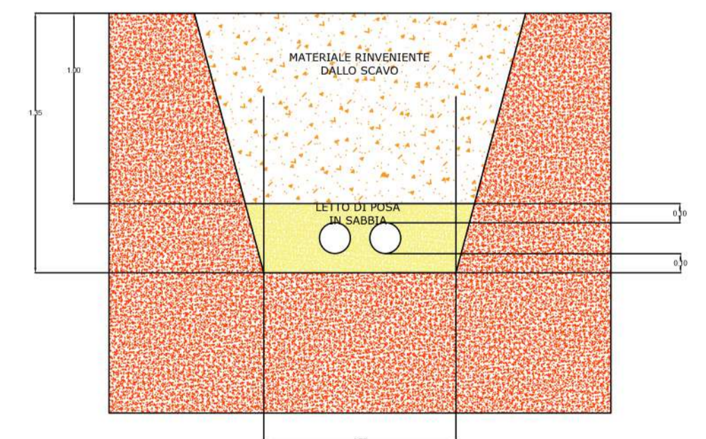
SEZIONE TIPO CAVIDOTTO INTERRATO MT SCALA 1 : 50
