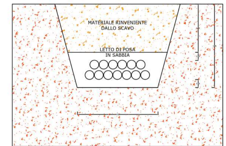
SEZIONE TIPO CAVIDOTTO INTERRATO MT SCALA 1 : 50
